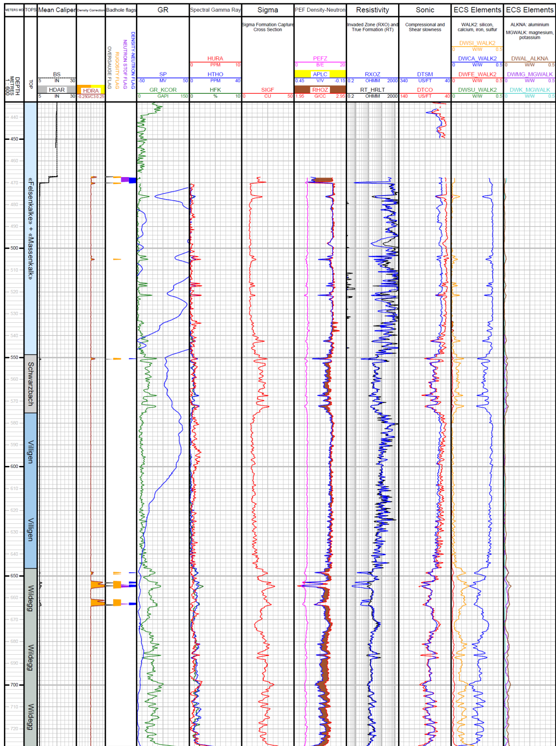
Fig. 3-1: Main logs of the composite dataset in the «Felsenkalke» + «Massenkalk» to Wildeggen Formation
