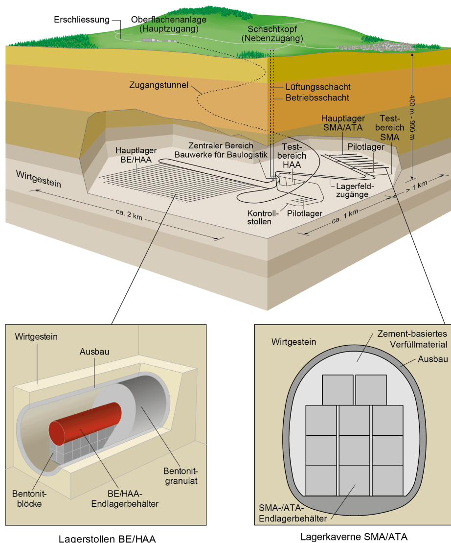
Fig. 3-1: Schematische Übersicht über die Anlagenelemente eines geologischen Tiefenlagers am Beispiel eines Kombilagers (Beispiel mit Zugangstunnel als Hauptzugang).
