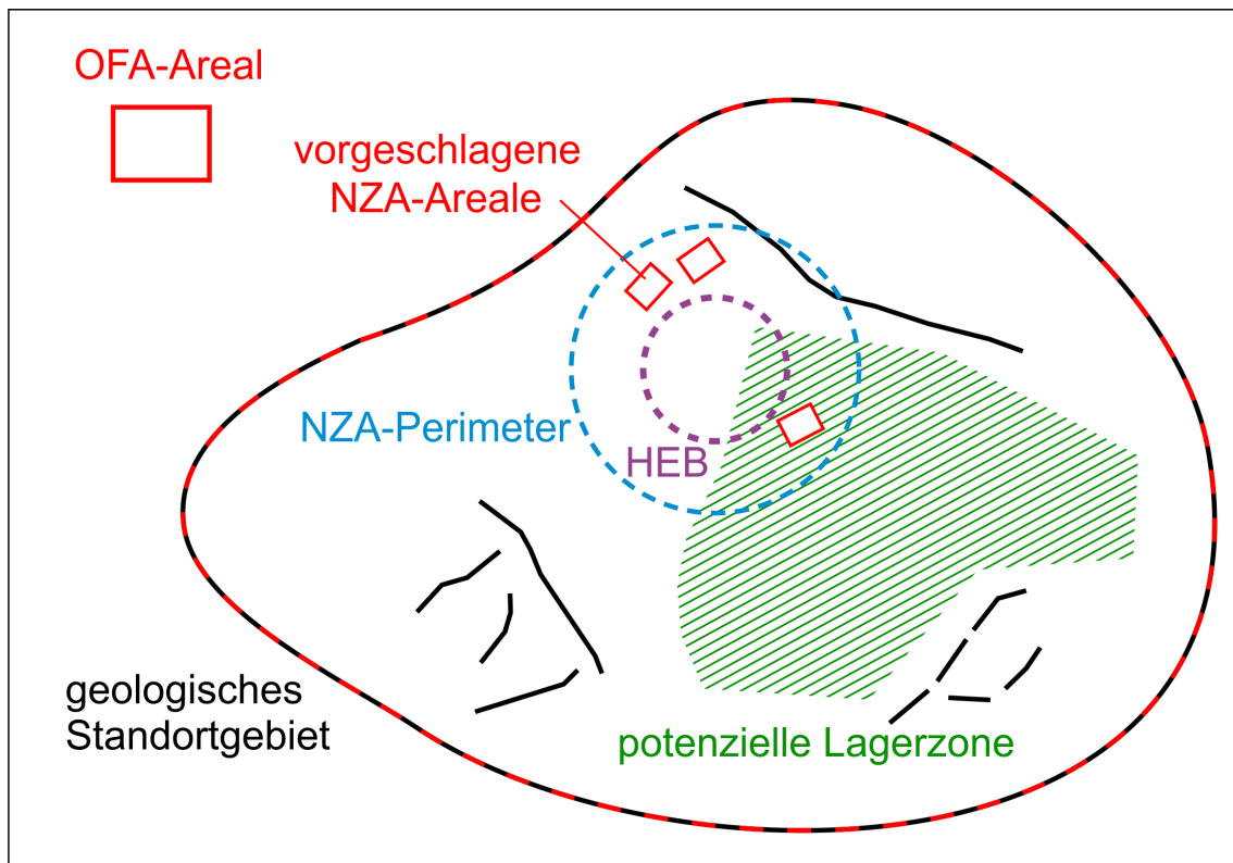
Fig. 5-4: NZA-Areale, die innerhalb des NZA-Perimeters festgelegt werden, der einen Radius von ca. 1'000 m rund um den Mittelpunkt des HEB aufweist.
