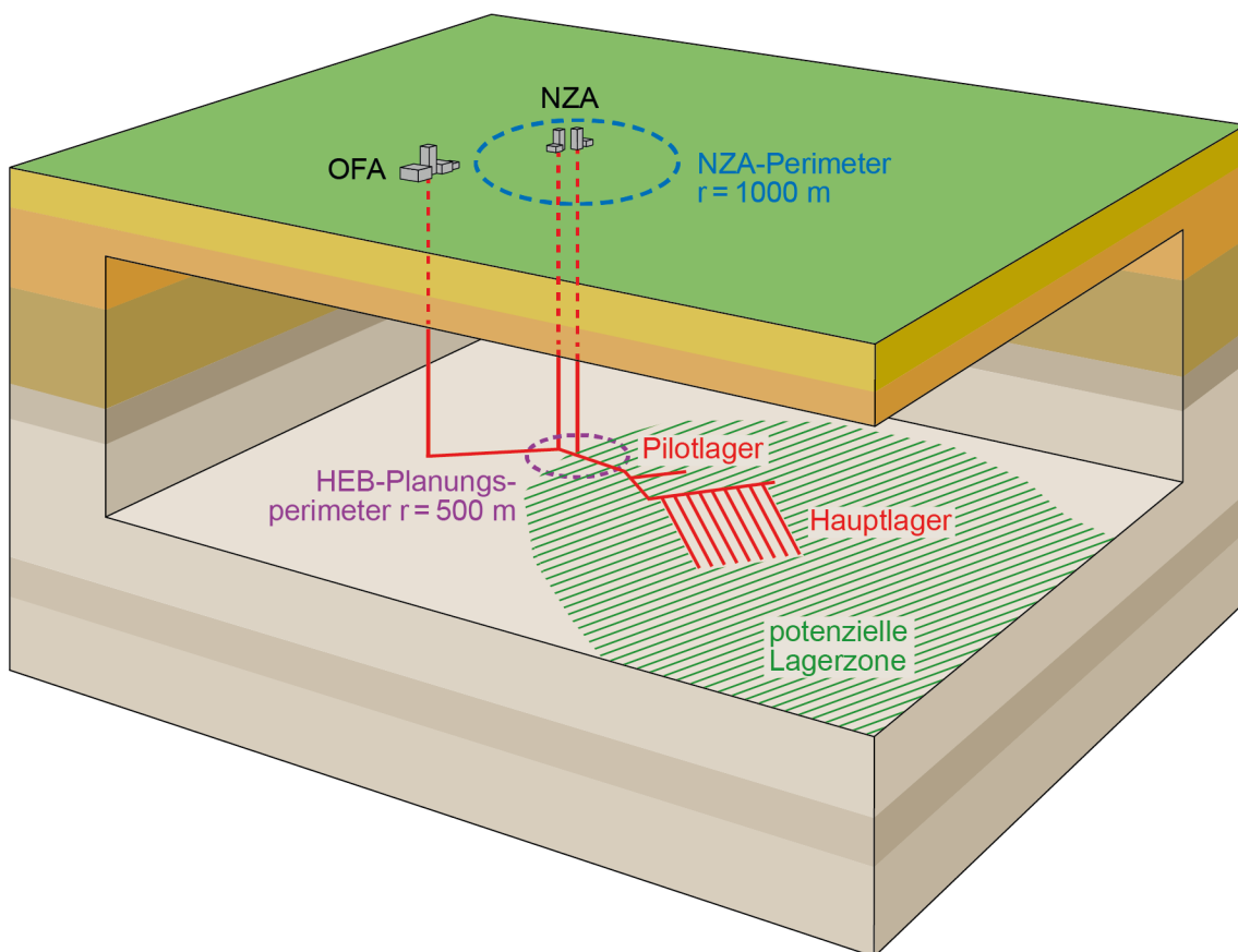
Fig. 5-2: Schematische Darstellung der wichtigsten Elemente des geologischen Tiefenlagers hinsichtlich der Vorschläge und der Zusammenarbeit in Etappe 3.
