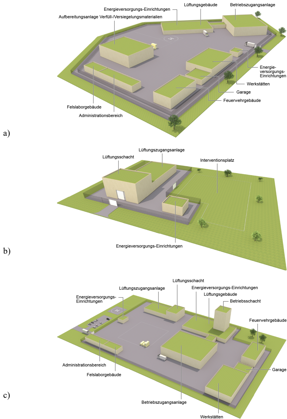
Fig. 3-4: Mögliche Anordnung und Ausgestaltung der funktional erforderlichen Bauwerke der Nebenzugangsanlagen.
