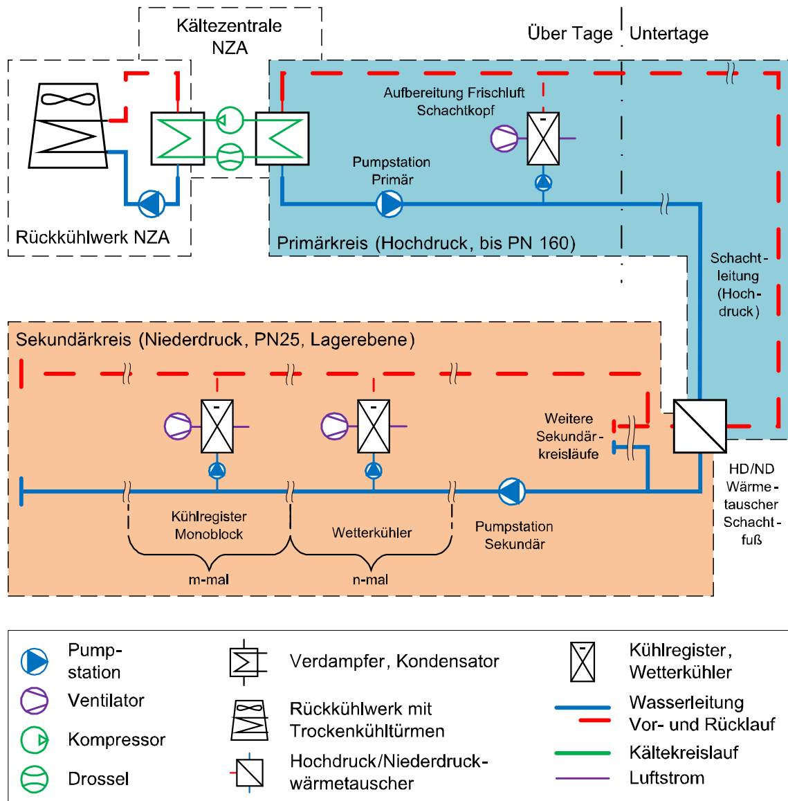
Fig. 4-2: Prinzipschema der Kühlung der UTA mit Anlagenkomponenten übertag und untertag
