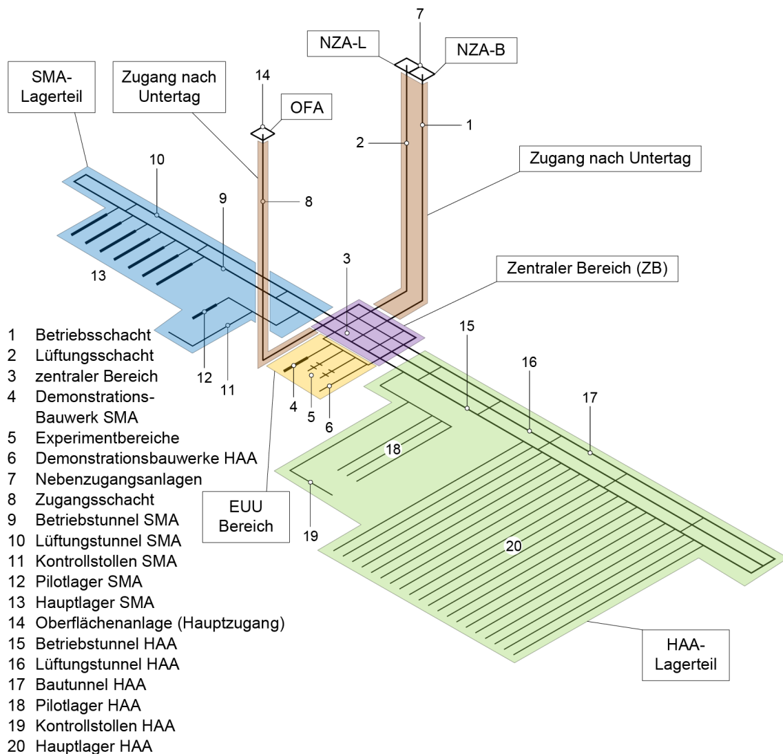
Fig. 2-1: Systemskizze für die untertägigen Bauten und Anlagen eines Kombilagers Siehe auch Nagra (2022)
