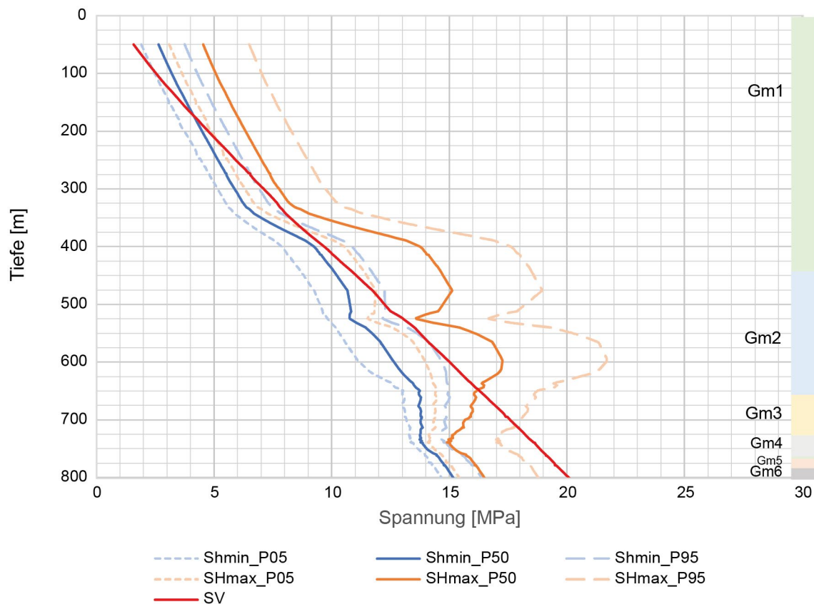
Fig. 6-5: Prognostiziertes Spannungsprofil am Standort des Betriebsschachts
