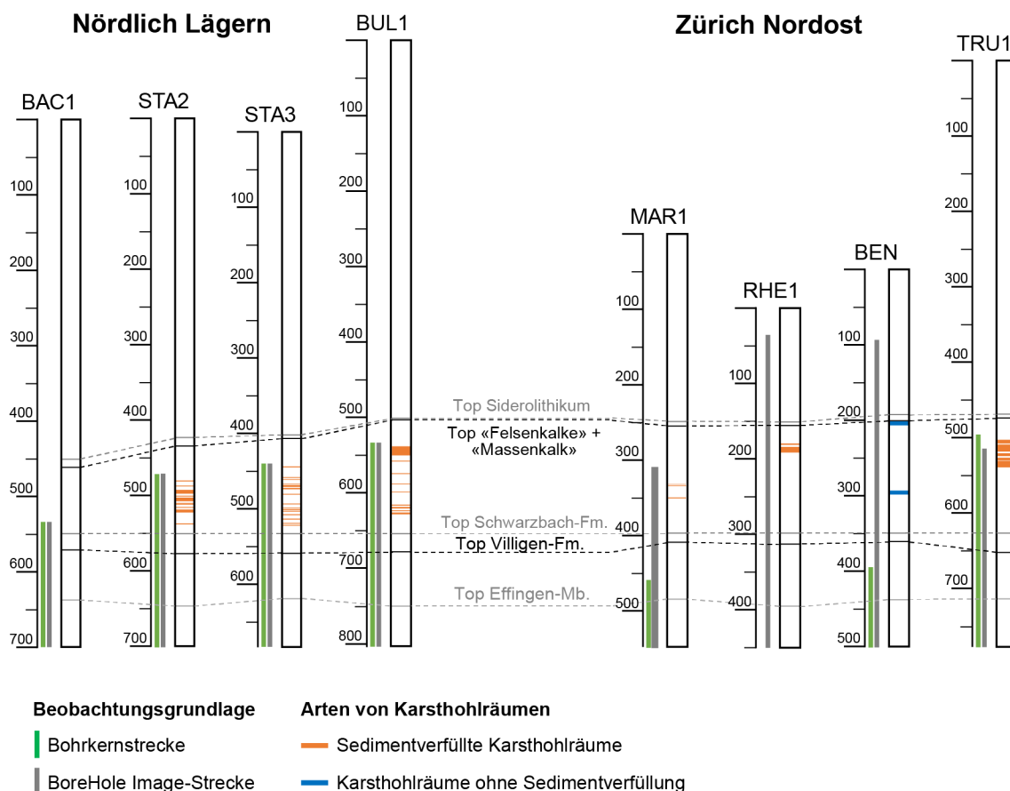
Fig. 7-2: Beobachtete Lösungshohlräume in den TBO der Standortgebiete Nordlich Lägern und Zürich Nordost
