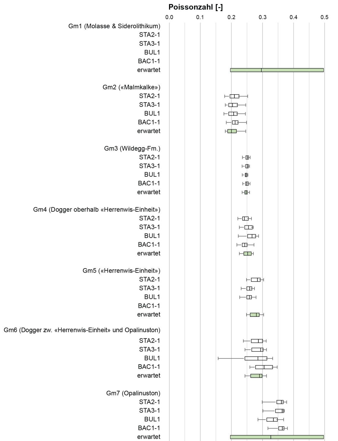
Fig. 6-4: Gegenüberstellung der Verteilung der modellierten Poissonzahlen
