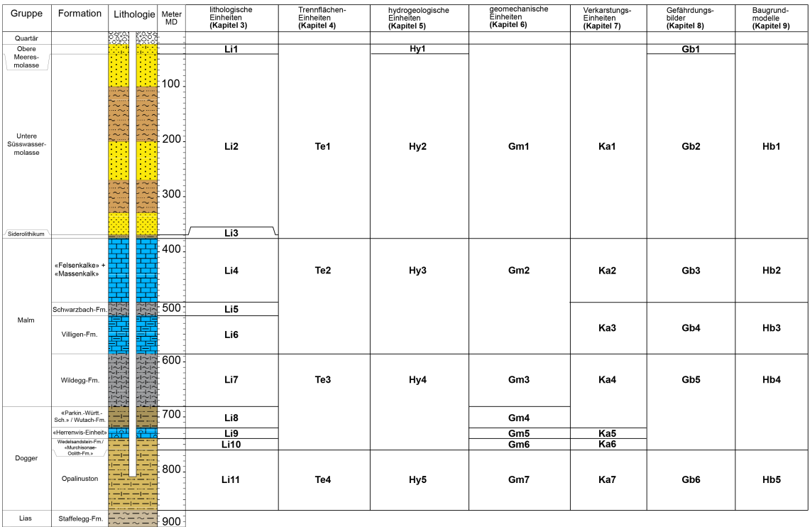
Fig. 1-4: Gegenüberstellung der Einheiten mit ähnlichen Eigenschaften am Standort des Lüftungsschachts (Prognoseprofil)
