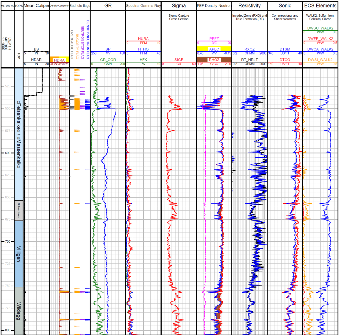
Fig. 3-2: Main logs of the composite dataset in the «Felsenkalke» / «Massenkalk» to Wildegg Formation
