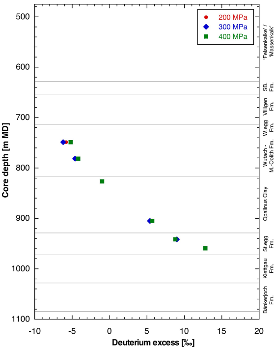
Fig. 4.6-8: Depth trend of deuterium excess
