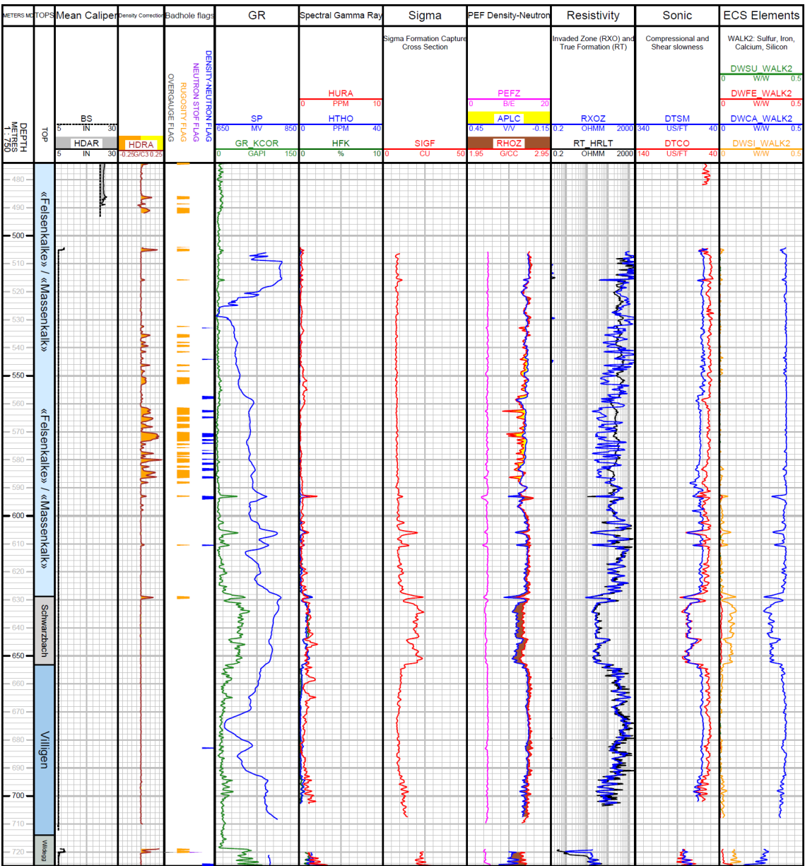
Fig. 3-3: Main logs of the composite dataset in the «Felsenkalke» + «Massenkalk» to Wildegg Formation
