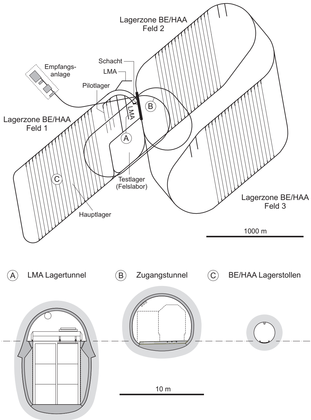
Fig. 2.5-2: Modellhafte Lagerauslegung HAA für das umhüllende Abfallinventar.
