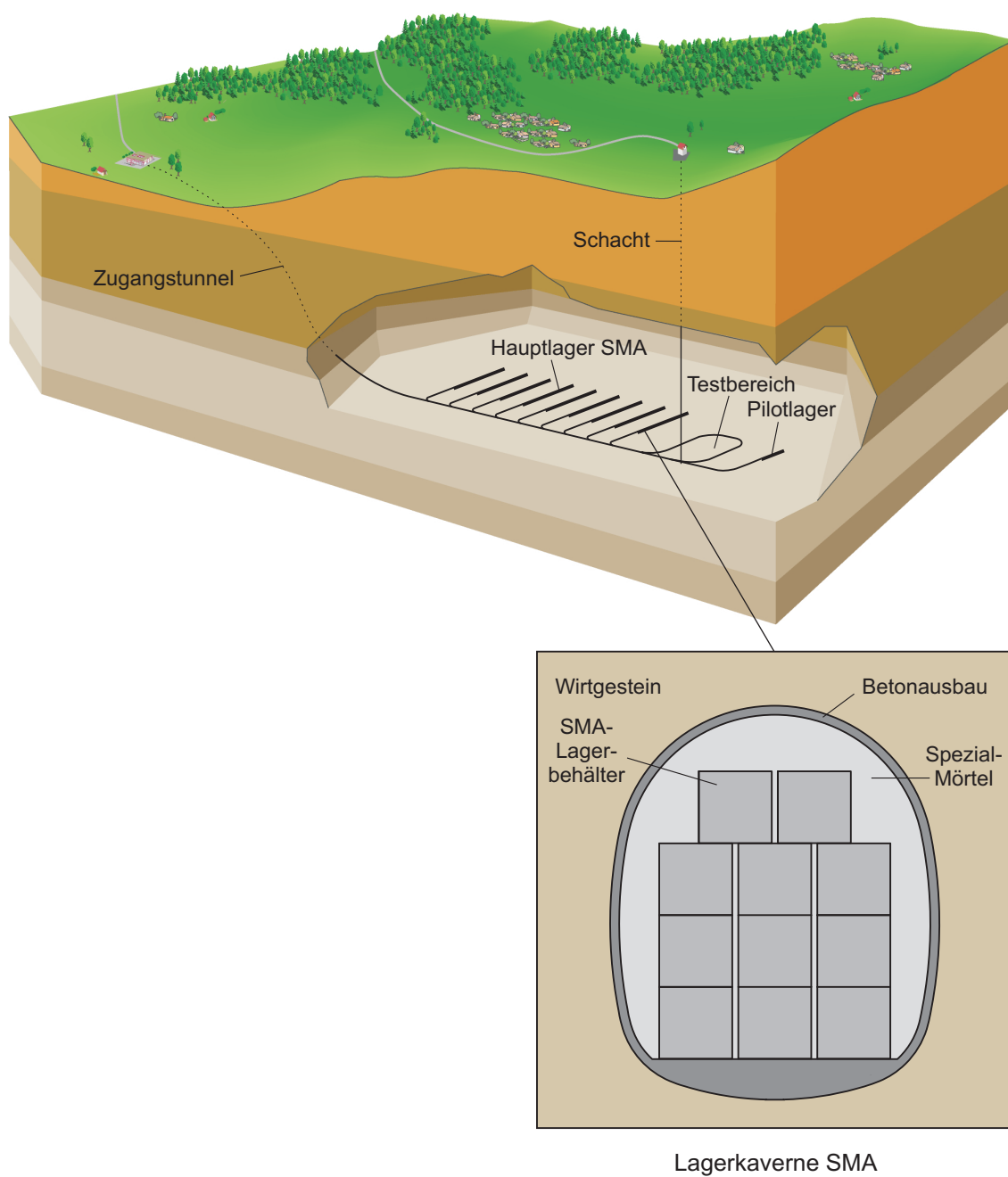
Fig. 4.3-1: Konzeptionelle Darstellung des geologischen Tiefenlagers SMA.
