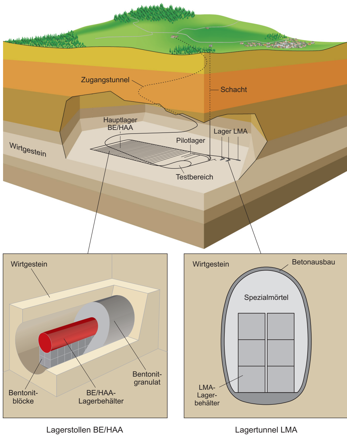
Fig. 4.3-2: Konzeptionelle Darstellung des geologischen Tiefenlagers HAA für abgebrannte Brennelemente (BE), verglaste hochaktive Abfälle aus der Wiederaufarbeitung (HAA) und langlebige mittelaktive Abfälle (LMA).
