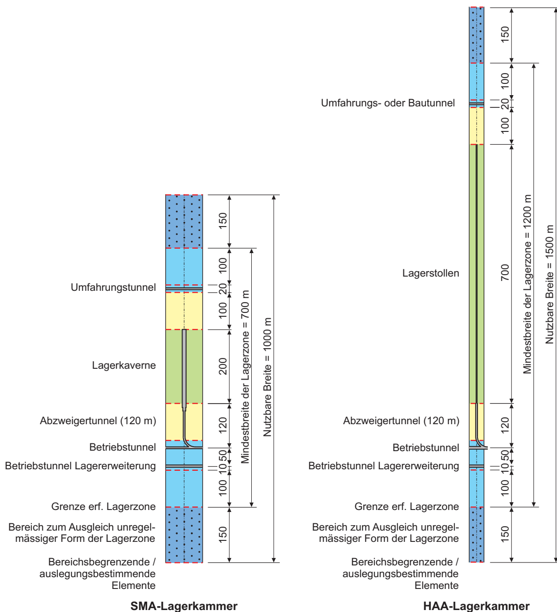
Fig. A2.5-3: Mindestbreite und nutzbare Breite für Lagerzonen SMA und HAA.
