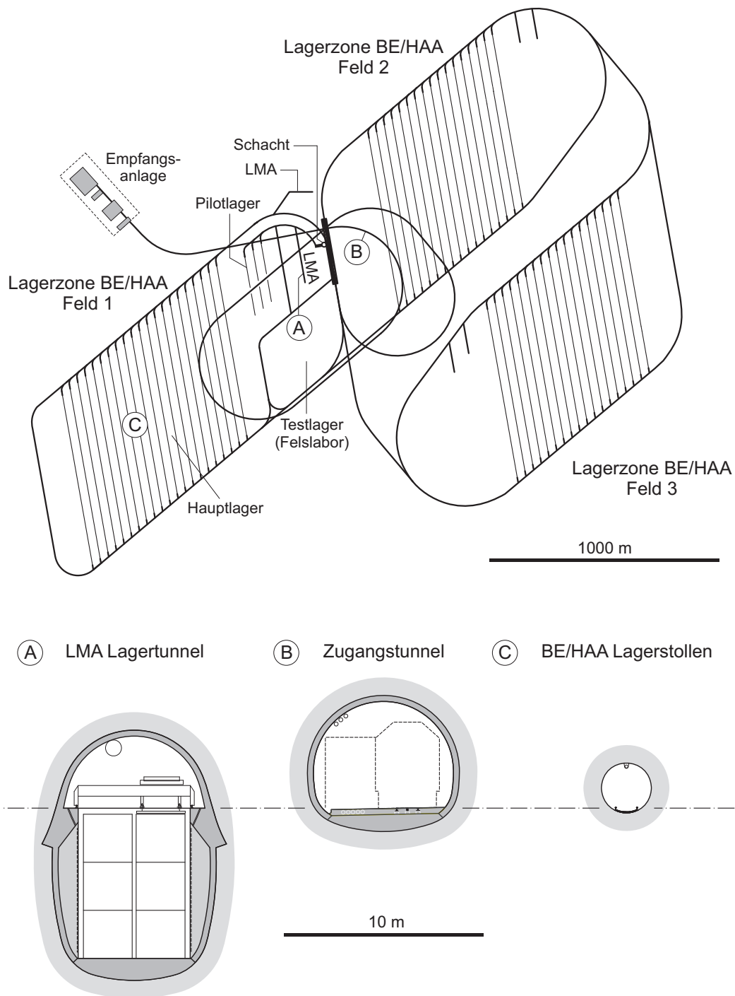
Fig. A2.6-1: Modellhafter Grundriss einer Lagerkonfiguration für ein HAA-Lager für das umhüllende Abfallinventar.
