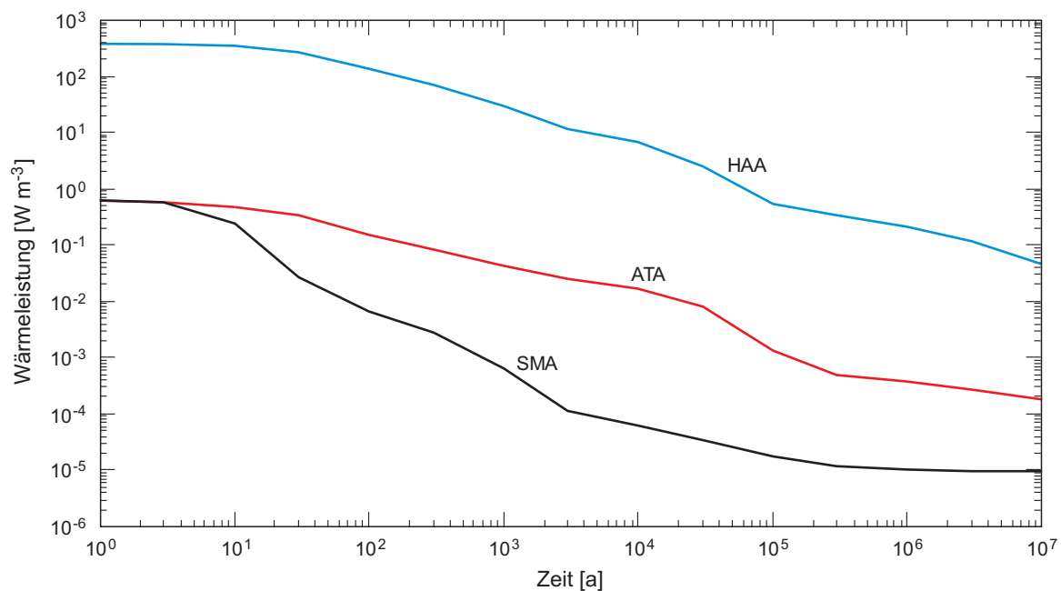
Fig. 3.2-3b: Zeitliche Entwicklung der spezifischen Wärmeleistung der Abfallkategorien gemäss Definition KEV.
