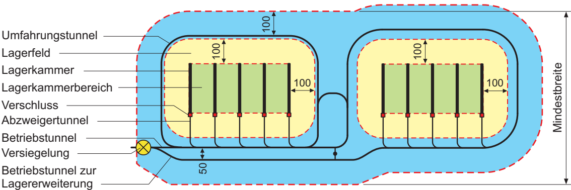
Fig. A2.5-1: Schematische Darstellung des Tiefenlager (Grundriss) mit seinen wichtigsten Elementen für das SMA- bzw. HAA-Lager.
