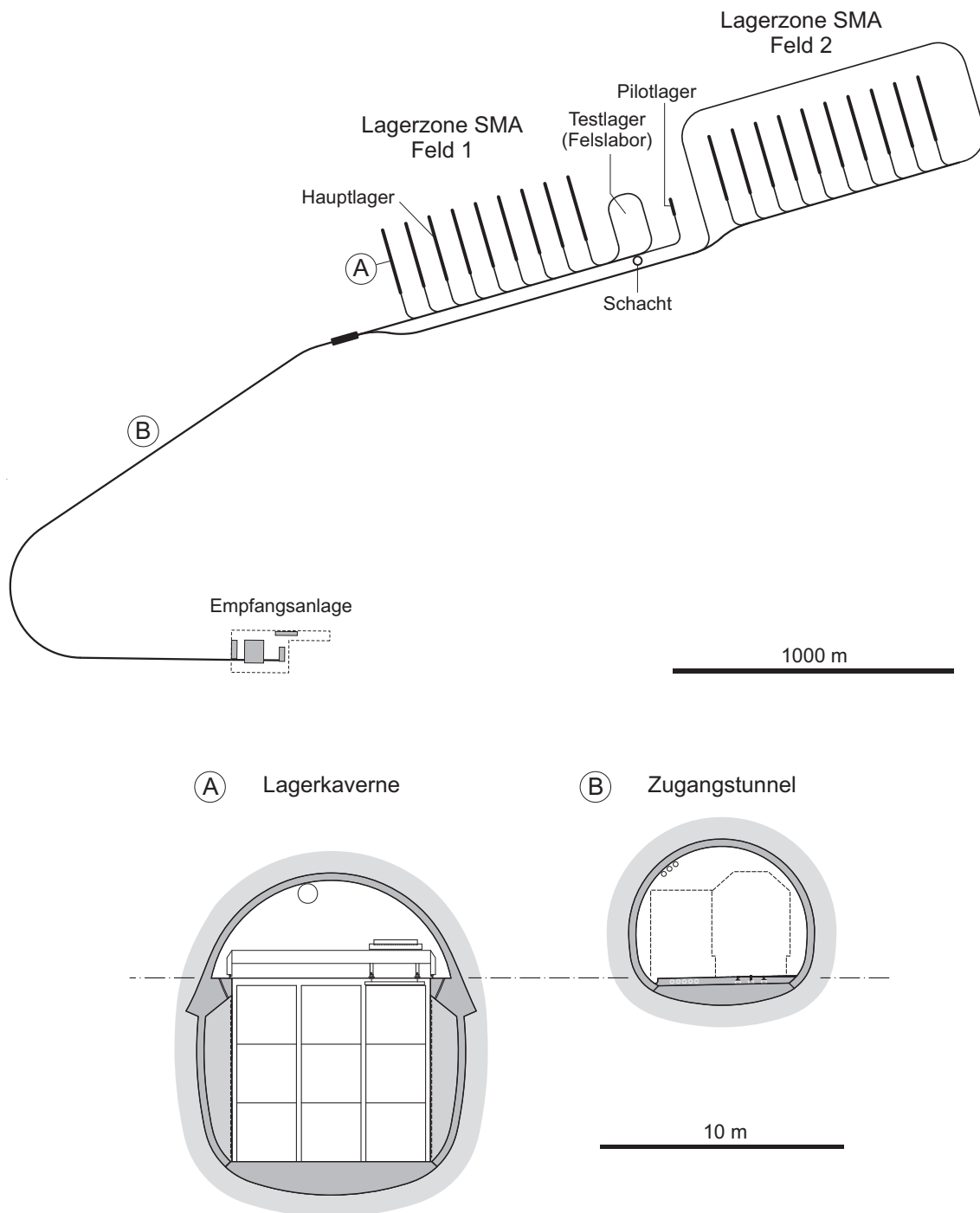
Fig. 2.5-1: Modellhafte Lagerauslegung SMA für das umhüllende Abfallinventar.
