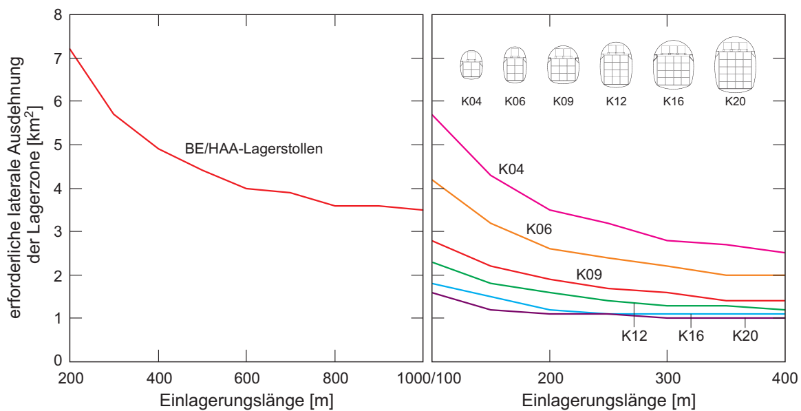
Fig. A2.6-4: Erforderliche Lagerzone in Abhängigkeit zur Einlagerungslänge für BE/HAA-Lagerstollen (links) und in Abhängigkeit zur Einlagerungslänge und Kavernengrösse für SMA-Lagerkavernen (rechts).
