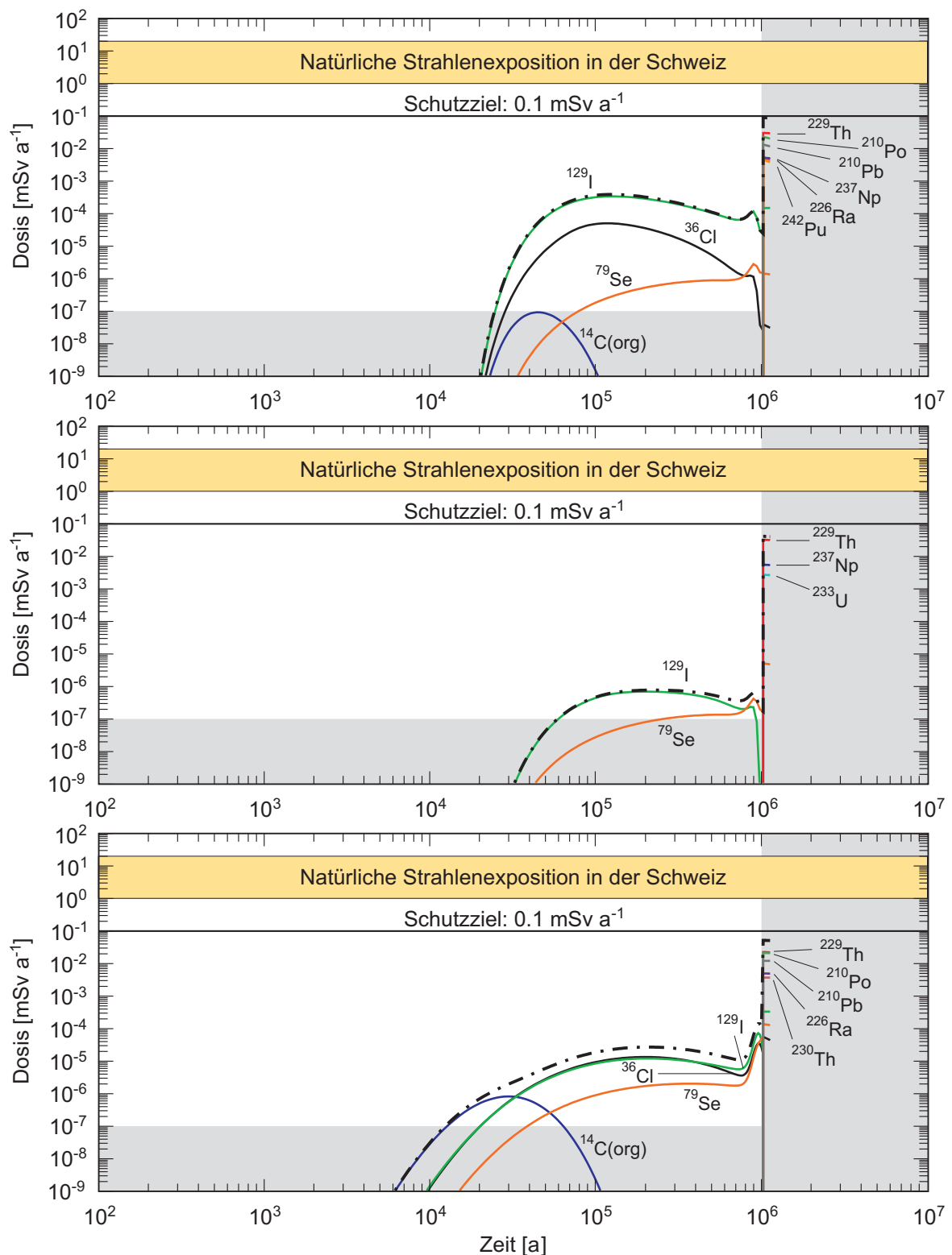
Fig. A5.4-5: Einfluss einer zeitabhängigen Dekompaktion auf ein HAA-Lager am Beispiel des Wirtgesteins Opalinuston gemäss Modell 3.
