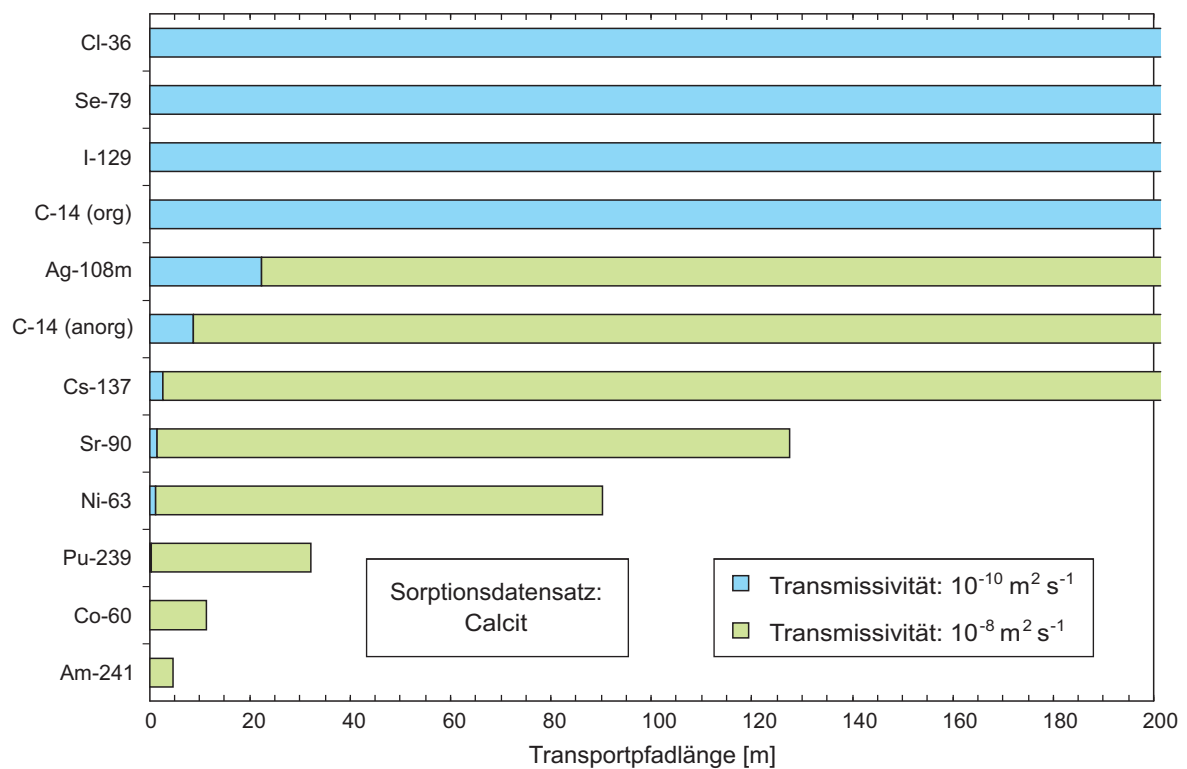
Fig. A5.5-20: Nuklidspezifische Reichweite (99 % Zerfall) in einer Kluft (Sorpton: Calcit).
