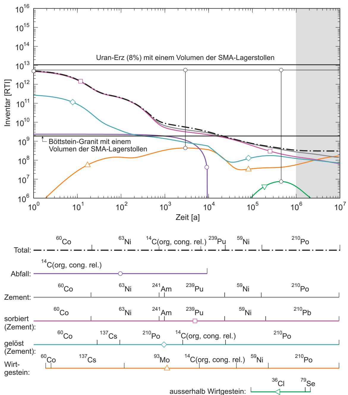
Fig. 4.7-5a: Entwicklung und Aufteilung der Radiotoxizität für ein SMA-Lager für K = 10^{-13} m/s.
