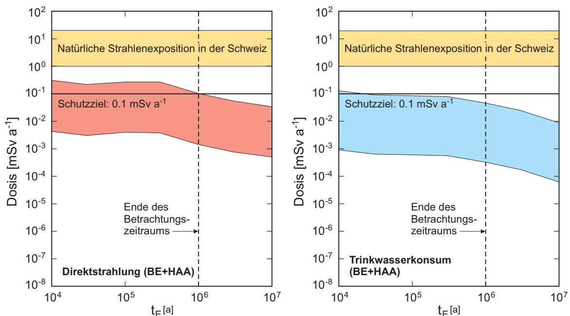
Fig. A5.4-2: Jährliche Strahlendosis gemäss Modell 2 als Funktion des Zeitpunkts der erosiven Freilegung ( t_E ) für das HAA-Lager (BE + HAA).
