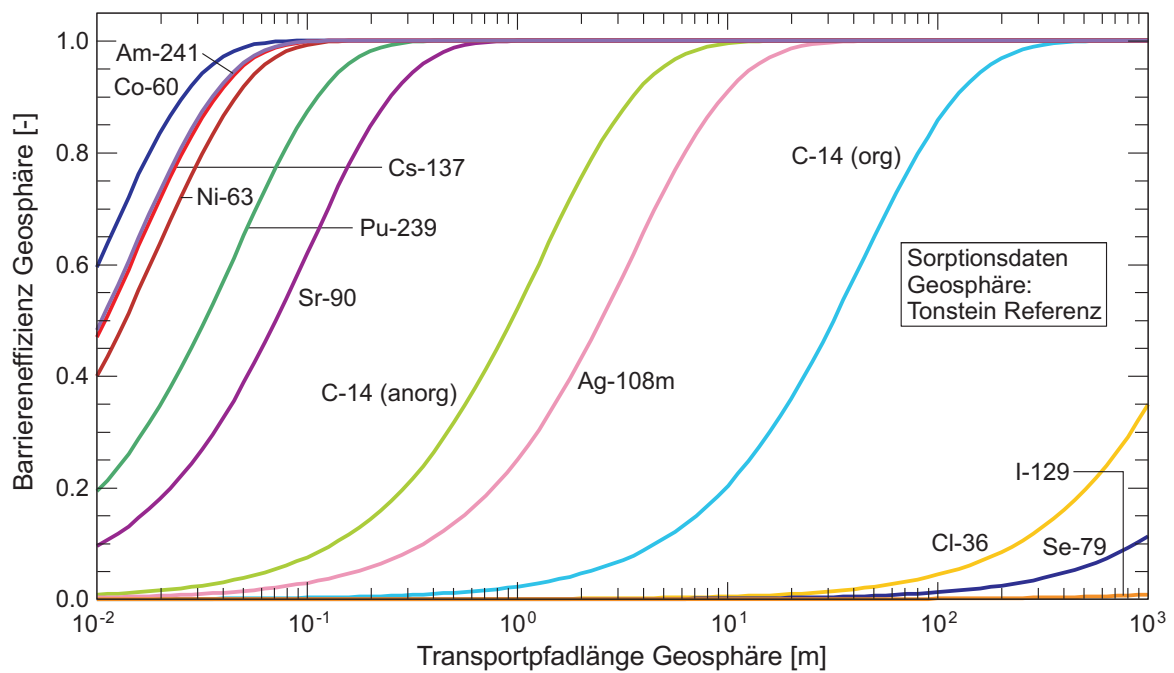
Fig. A5.5-13: Barriereneffizienz als Funktion der Transportpfadlänge (geklüftetes Wirtgestein, i = 0.1 m/m, T = 10^{-10} m 2 /s, Sorption: Tonstein).
