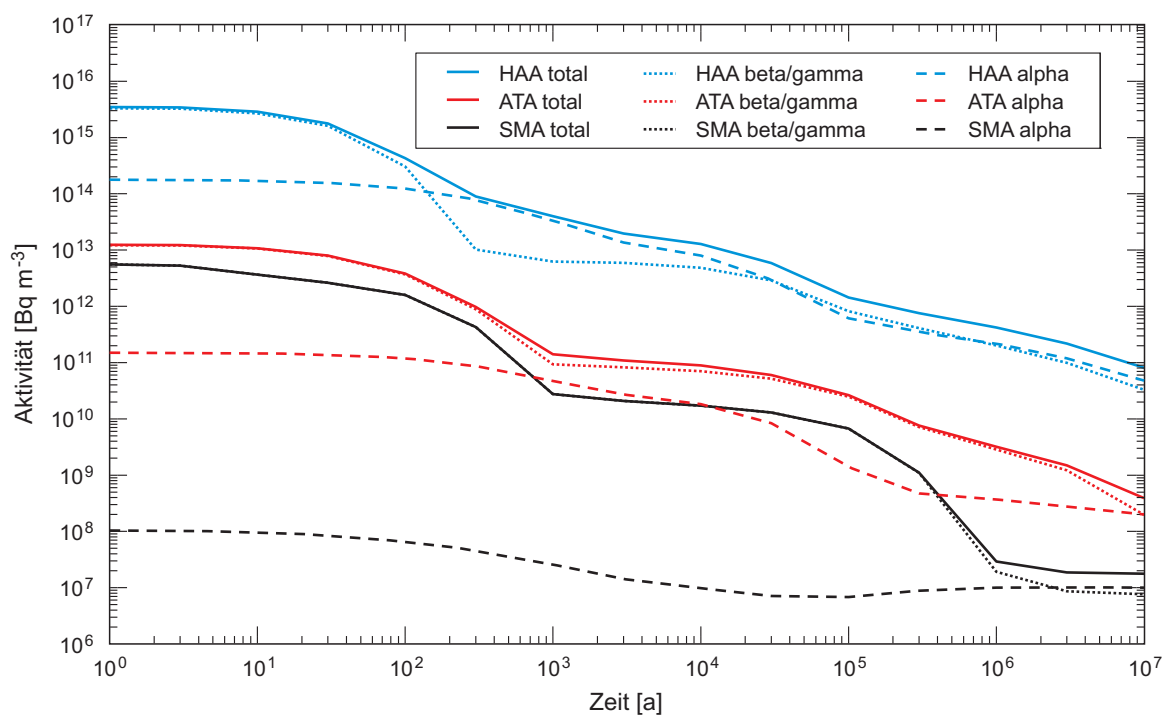
Fig. 3.2-1b: Zeitliche Entwicklung der spezifischen Aktivität der Abfallkategorien gemäss Definition KEV.
