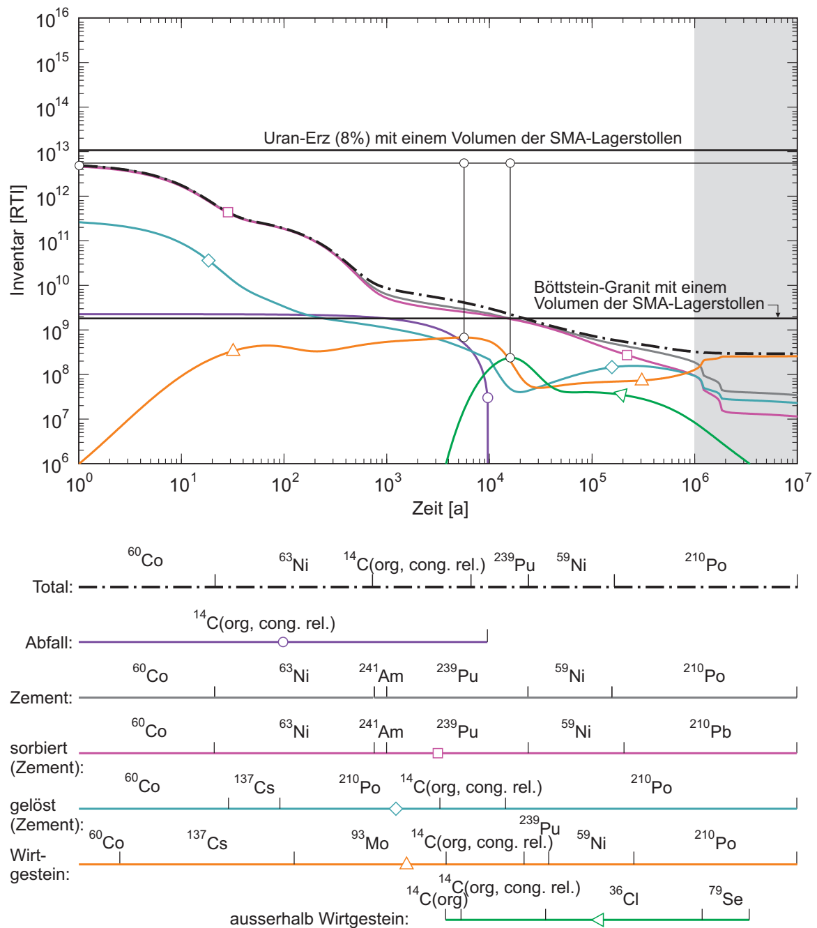
Fig. 4.7-5b: Entwicklung und Aufteilung der Radiotoxizität für ein SMA-Lager für K = 10^{-10} m/s.
