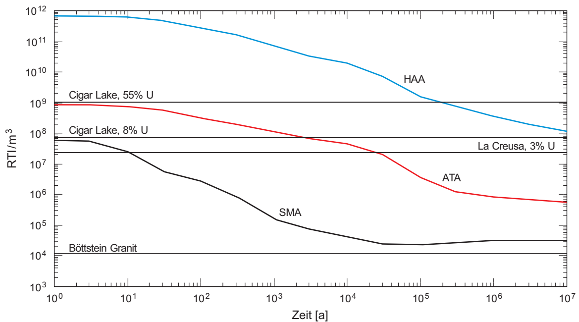
Fig. 3.2-2b: Zeitliche Entwicklung der spezifischen Radiotoxizität der Abfallkategorien gemäss Definition KEV.
