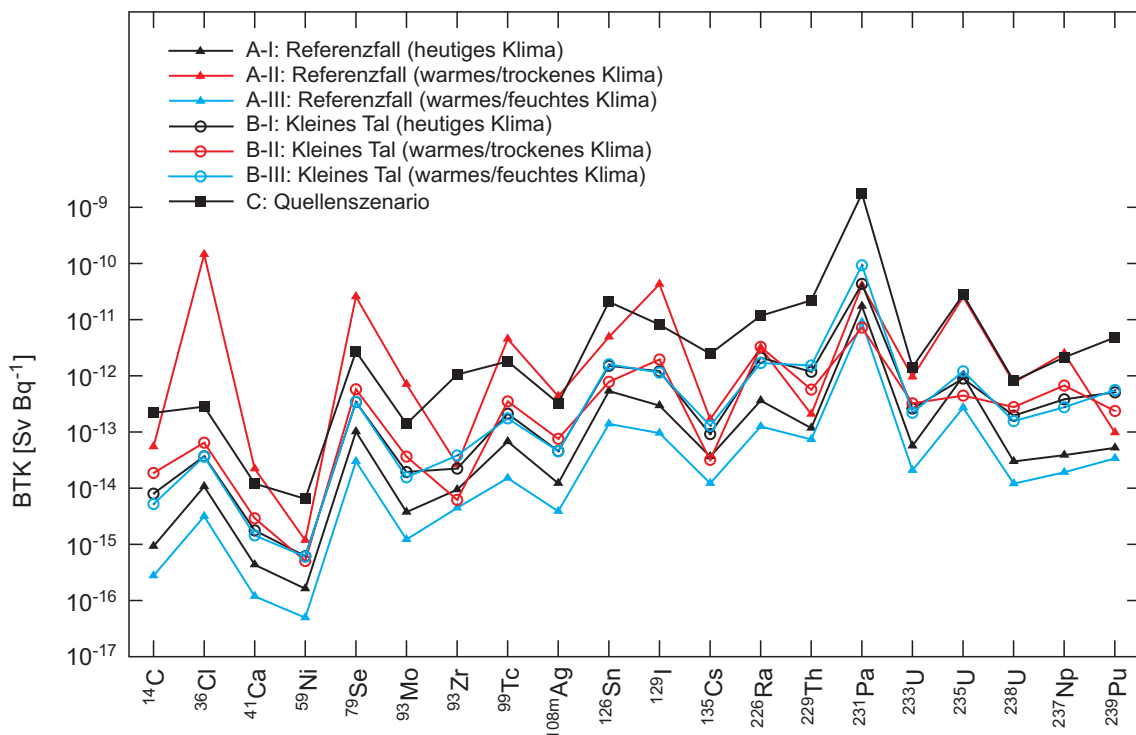
Fig. 2.5-5: Vergleich der Biosphären-Transfer-Koeffizienten für die verschiedenen Biosphärentypen (A, B, C) und Klimaszenarien (I, II, III) für eine Auswahl von sicherheitsrelevanten Nukliden.
