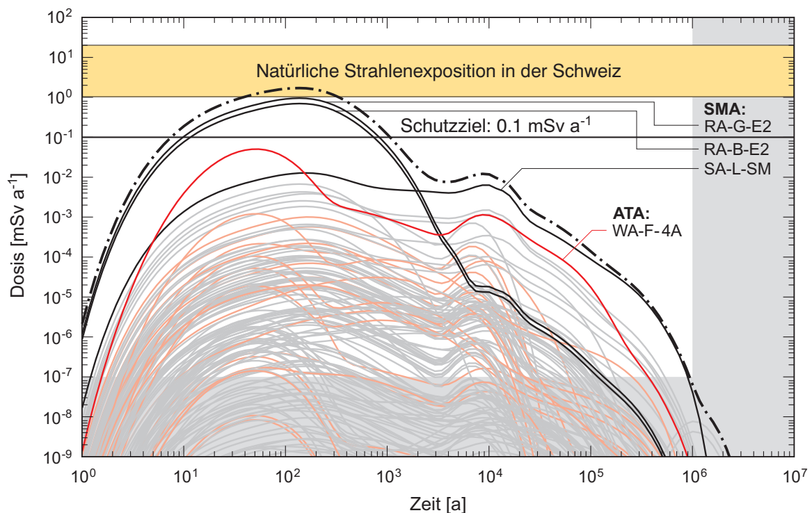
Fig. 3.2-6b: Berechnete Dosen für alle ATA- und SMA-Abfallsorten im SMA-Lager für ein homogen-poröses Wirtgestein mit Störungszonen.
