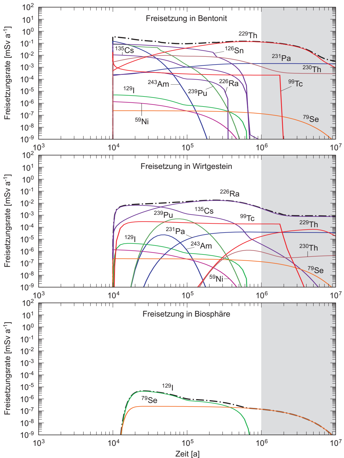
Fig. 4.7-8b: Radionuklid-Transferraten für verglaste hochaktive Abfälle für K = 10^{-10} m/s.
