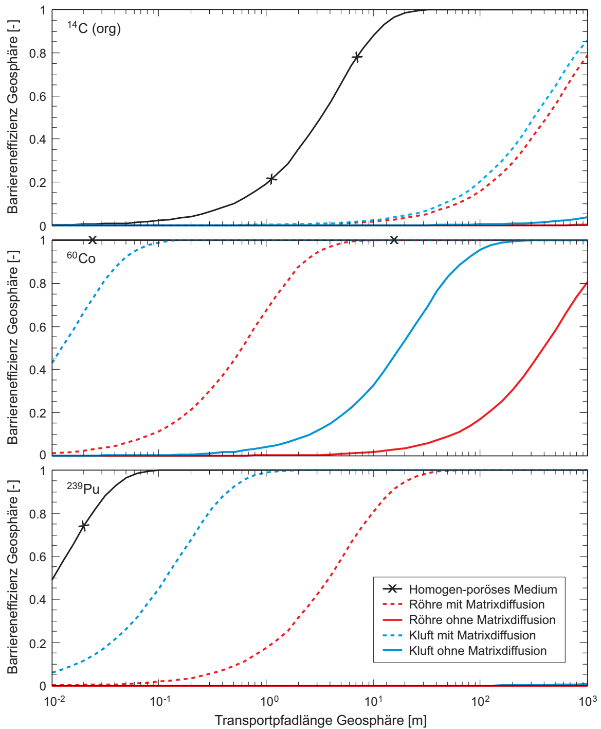
Fig. A5.5-21: Einfluss der Art der Transportpfade (homogen-poröses Medium, Kluft, Röhre bzw. Channel) und der Ausbildung des Porenraums (mit/ohne diffusionszugänglicher Matrix) auf die Barriereneffizienz für drei ausgewählte Beispielnuklide.
