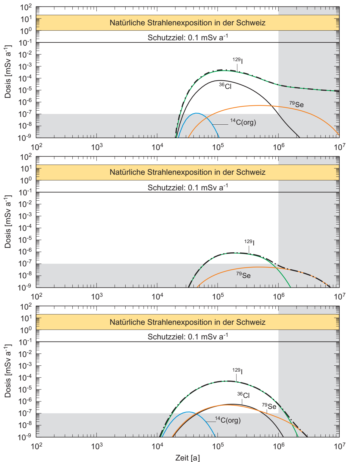
Fig. 4.7-4a: Berechnete Dosen für ein HAA-Lager in einem homogen-porösen Wirtgestein für K = 10^{-13} m/s.
