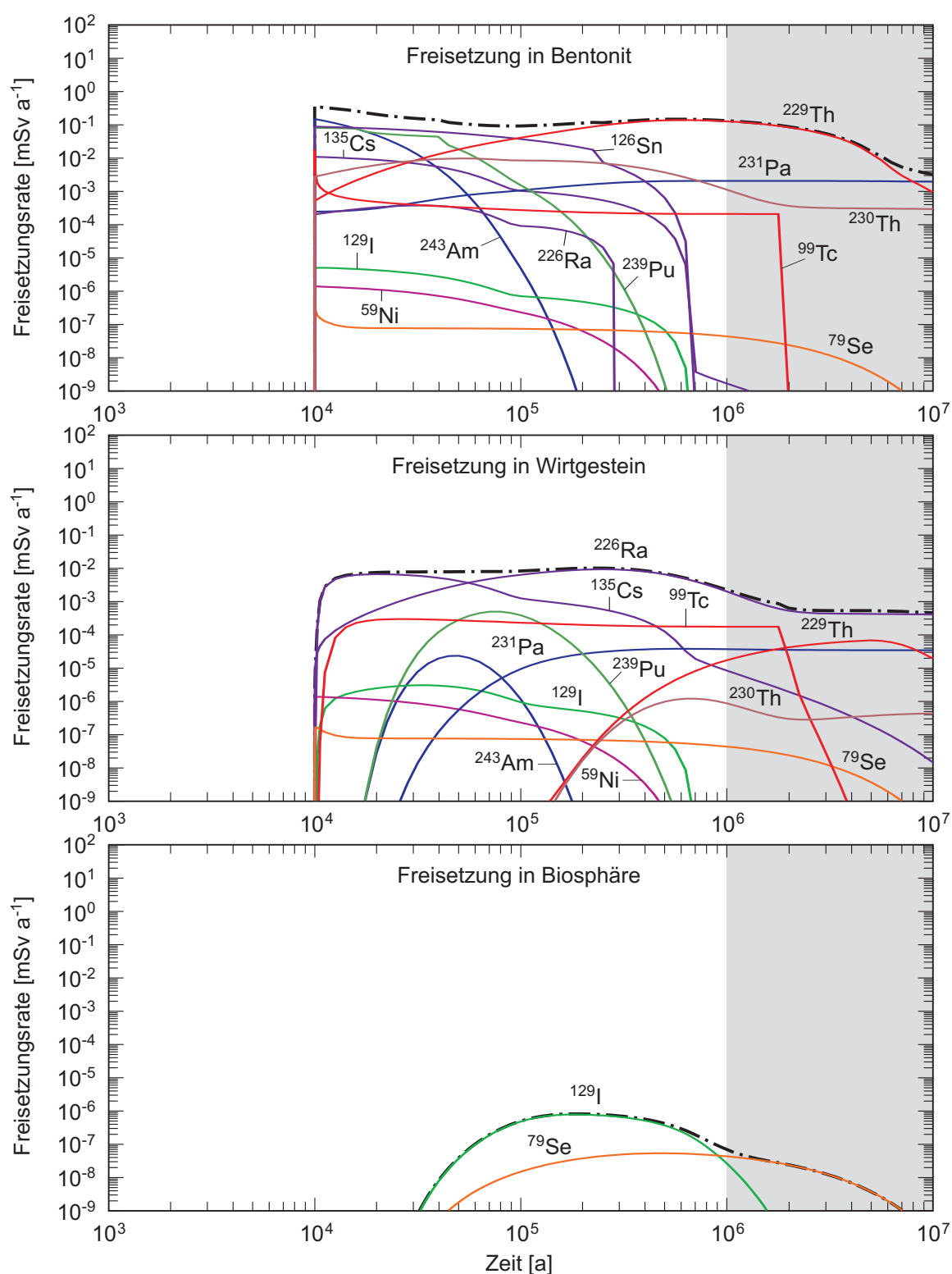
Fig. 4.7-8a: Radionuklid-Transferraten für verglaste hochaktive Abfälle für K = 10^{-13} m/s.
