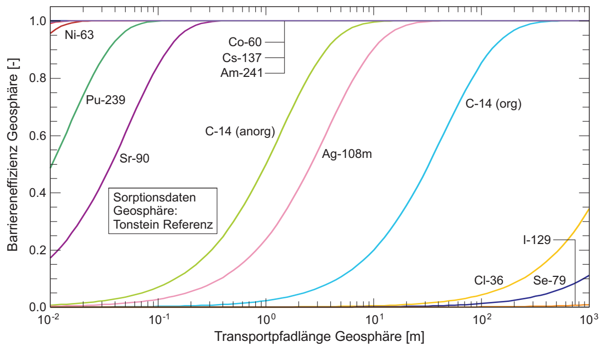
Fig. A5.5-10: Barriereneffizienz als Funktion der Transportpfadlänge (homogen-poröses Wirtgestein, i = 0.1 m/m, K = 10^{-10} m/s, Sorption: Tonstein).
