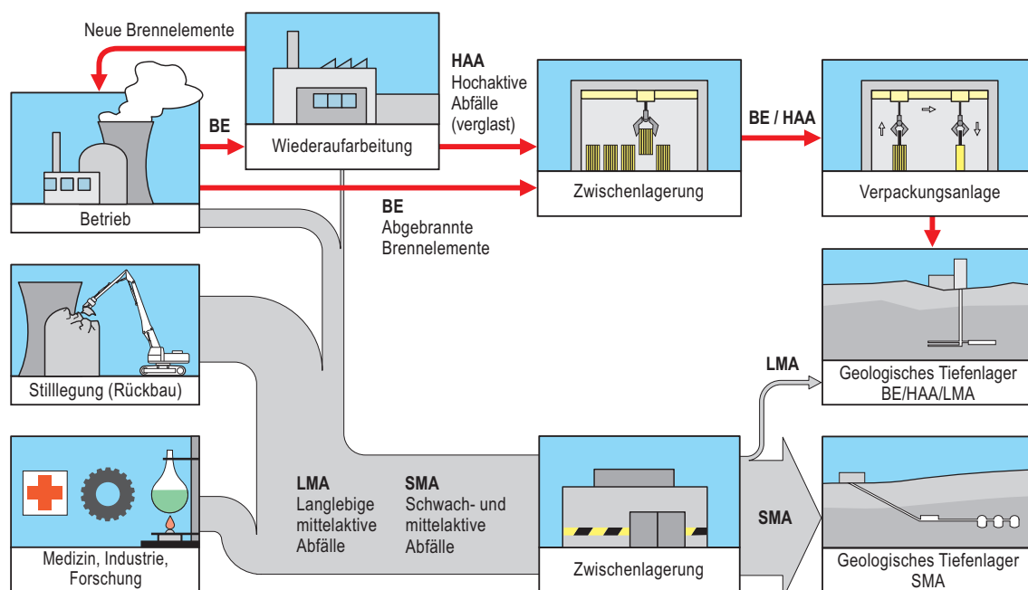
Fig. 1.2-1: Übersicht über die Verursacher von radioaktiven Abfällen und das Entsorgungskonzept.
