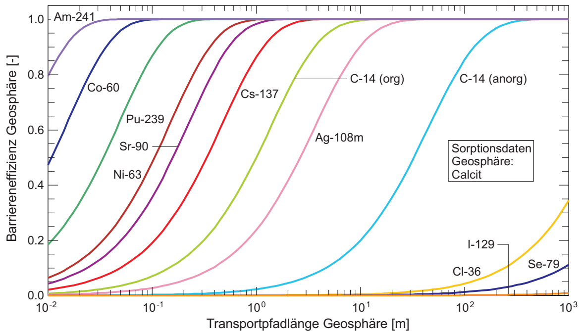
Fig. A5.5-12: Barriereneffizienz als Funktion der Transportpfadlänge (homogen-poröses Wirtgestein, i = 0.1 \text{ m/m} , K = 10^{-10} \text{ m/s} , Sorption: Calcit).
