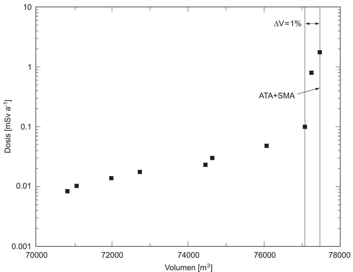
Fig. 3.2-6a: Berechnete Dosis als Funktion des Abfallvolumens im SMA-Lager für ein homogen-poröses Wirtgestein mit Störungszonen.
