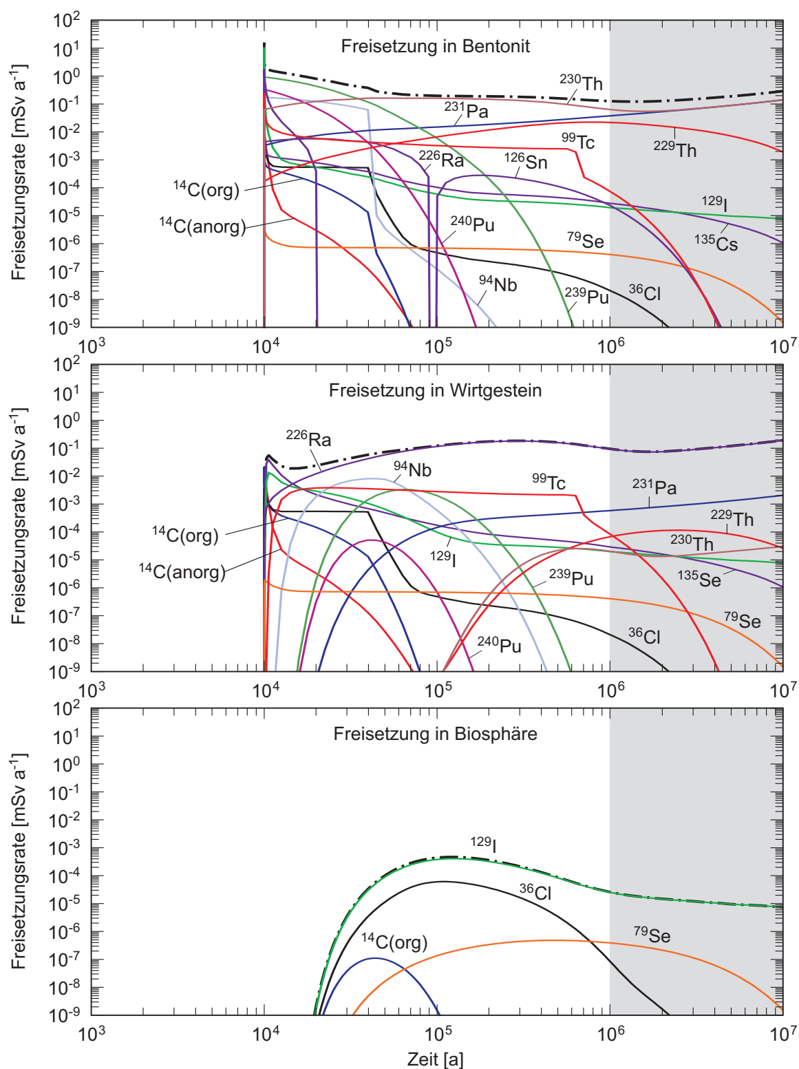
Fig. 4.7-7a: Radionuklid-Transferraten für abgebrannte Brennelemente für K = 10^{-13} m/s.
