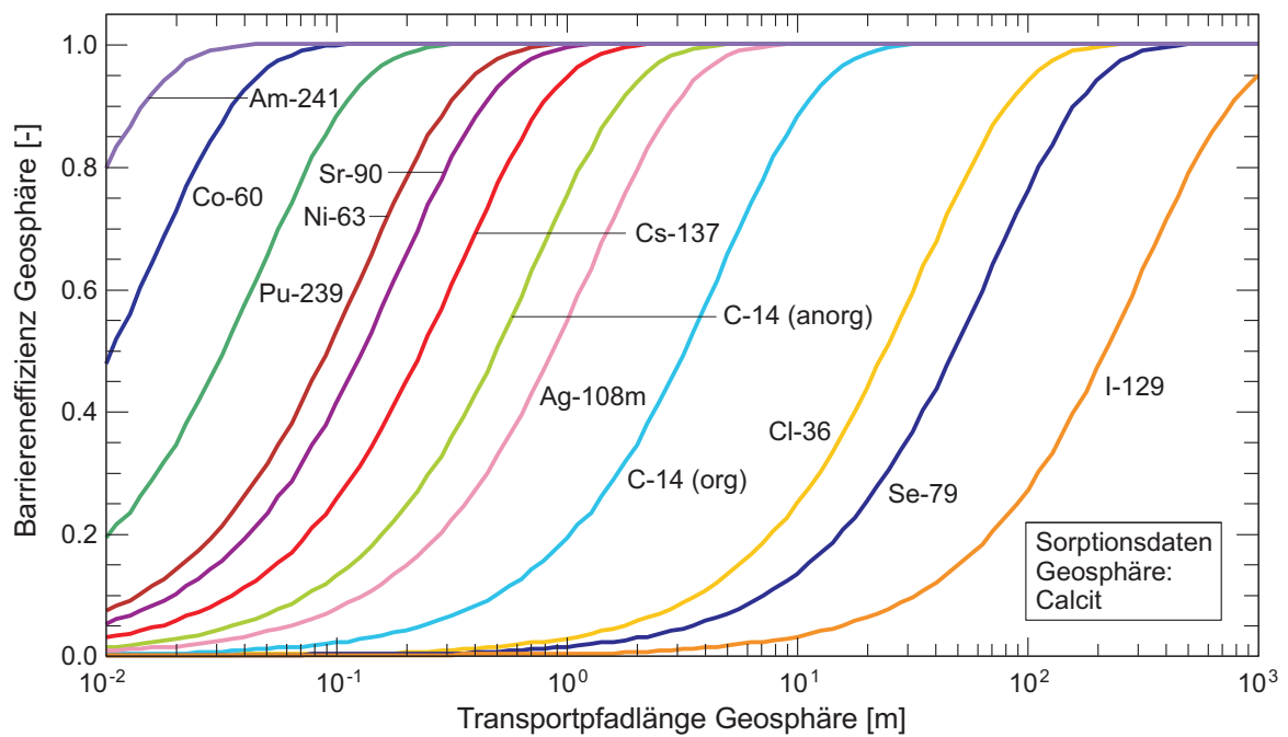
Fig. A5.5-11: Barriereneffizienz als Funktion der Transportpfadlänge (homogen-poröses Wirtgestein, i = 0.1 \text{ m/m} , K = 10^{-13} \text{ m/s} , Sorption: Calcit).
