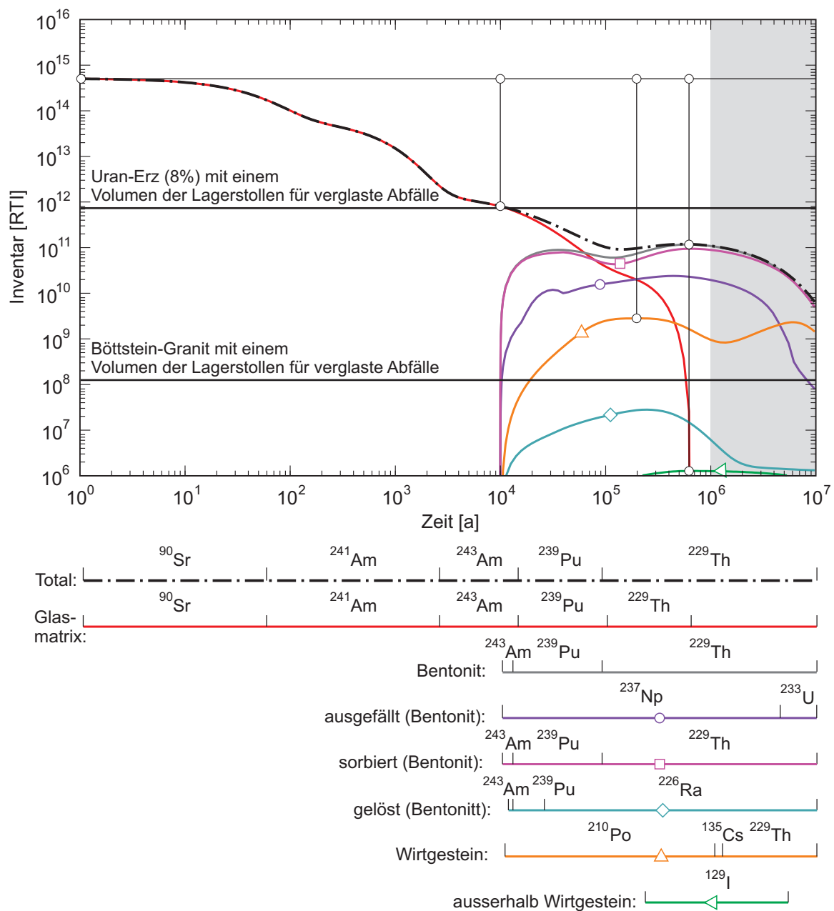
Fig. 4.7-2b: Entwicklung und Aufteilung der Radiotoxizität für verglaste hochaktive Abfälle auf die verschiedenen Komponenten des Nahfelds, das Wirtgestein und das Gebiet ausserhalb des Wirtgesteins für K = 10^{-10} m/s.
