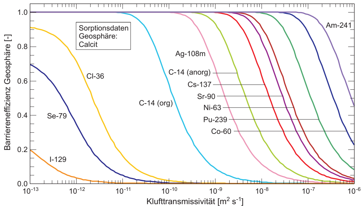
Fig. A5.5-8: Barriereneffizienz als Funktion der Transmissivität (geklüftetes WG, i = 0.1 \text{ m/m} , L = 40 \text{ m} , Sorption: Calcit).
