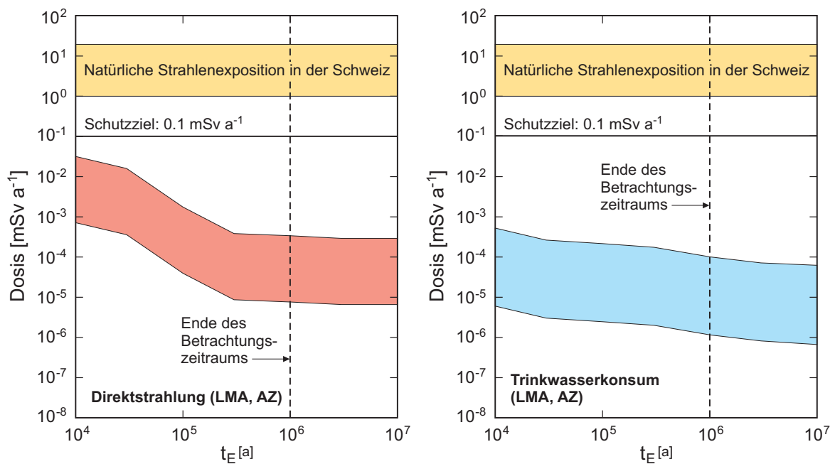
Fig. A5.4-3: Jährliche Strahlendosis gemäss Modell 2 als Funktion des Zeitpunkts der erosiven Freilegung ( t_E ) für das HAA-Lager (LMA-Teil).
