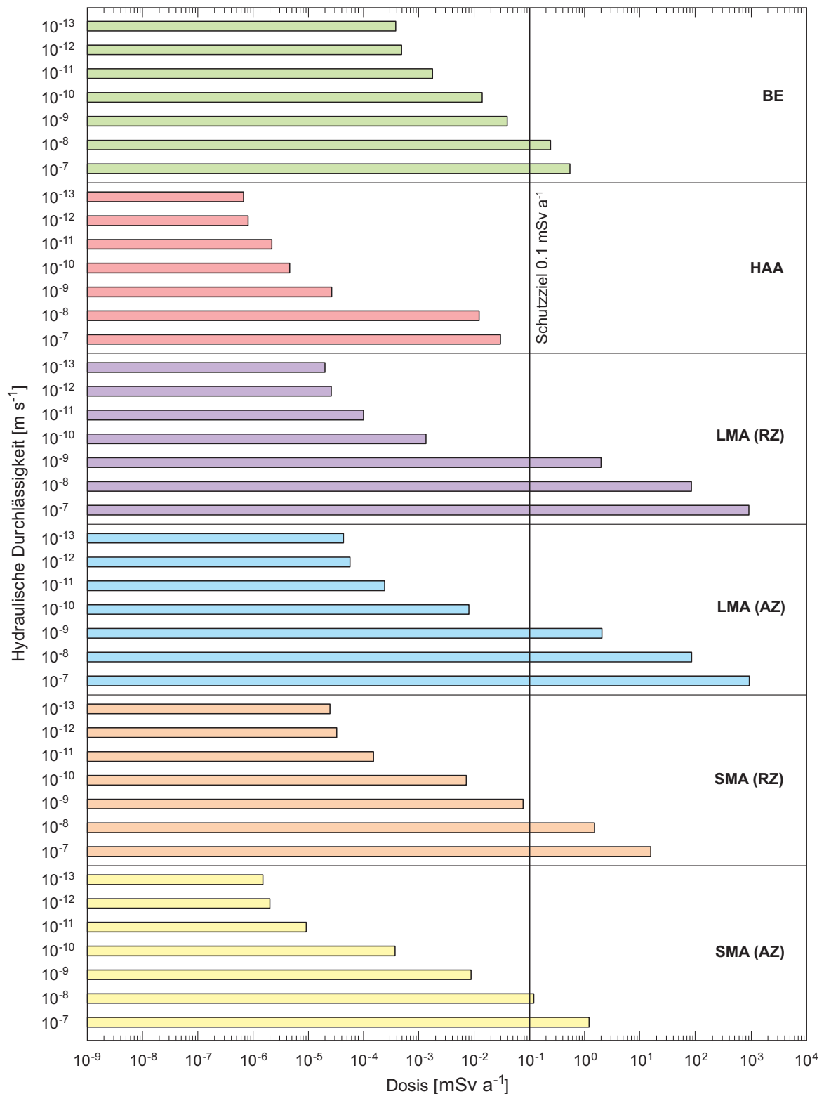
Fig. A5.2-1: Einfluss der hydraulischen Durchlässigkeit eines homogen-porösen Wirtgesteins auf die berechneten Dosismaxima.
