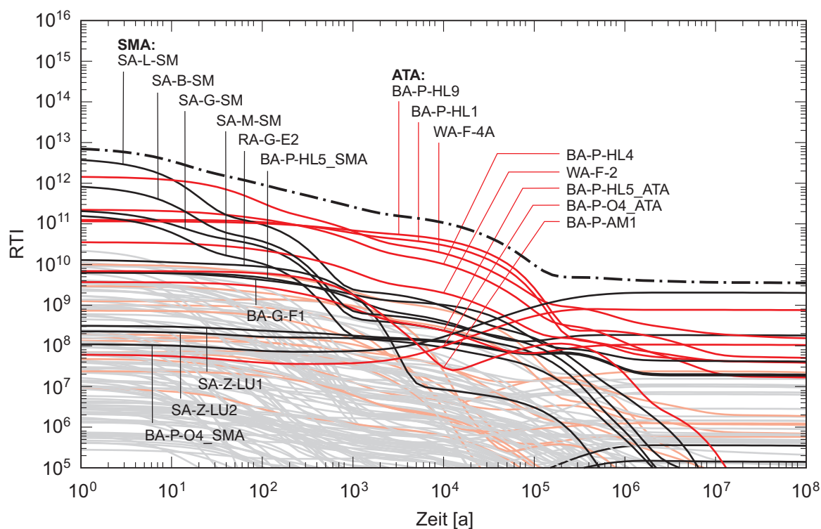
Fig. 3.2-2c: Zeitliche Entwicklung der Radiotoxizität der einzelnen Abfallsorten der Abfallkategorien ATA (rot) und SMA (schwarz).
