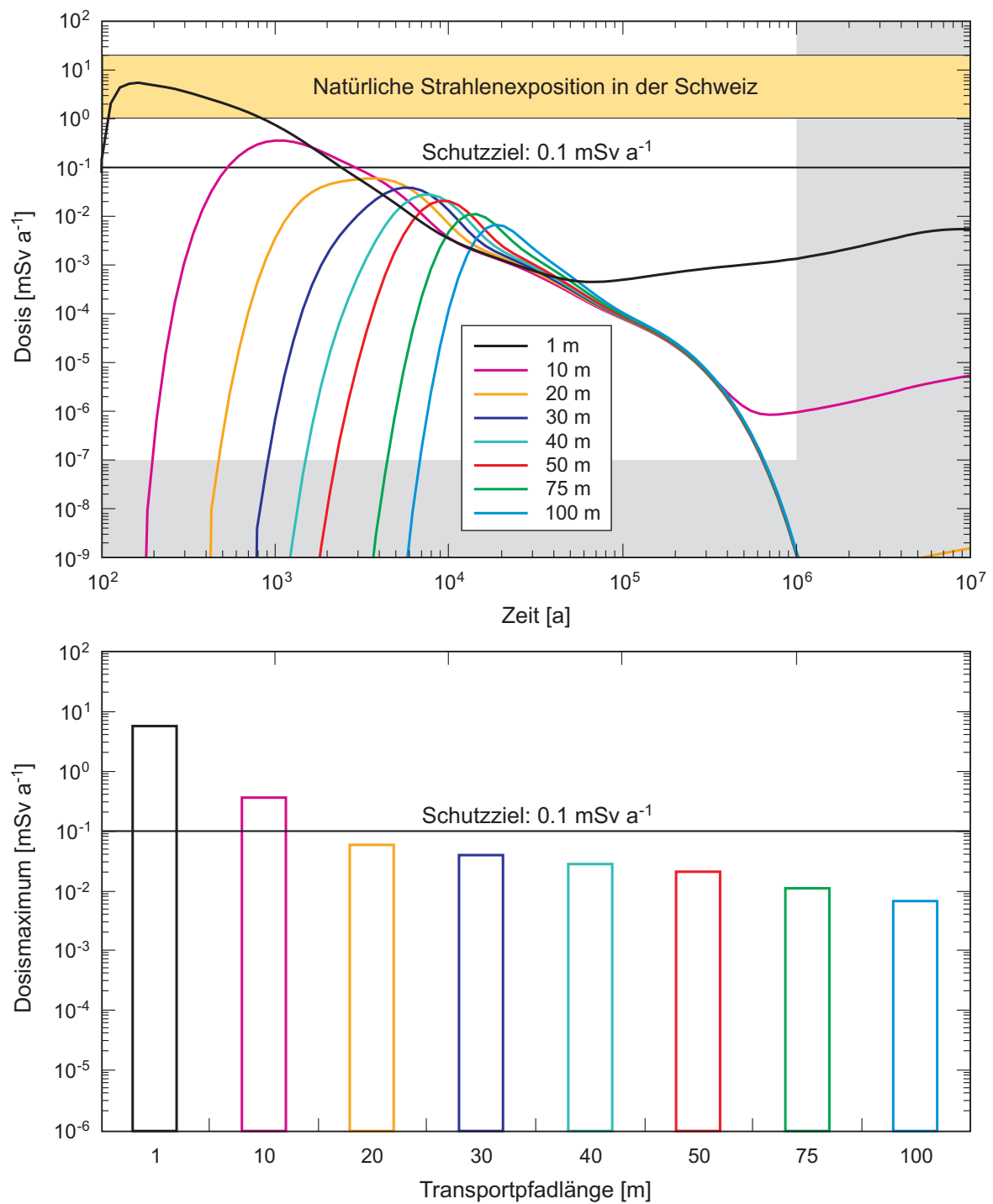
Fig. A5.3-4: Einfluss der Transportpfadlänge auf die berechneten Dosismaxima für ein HAA-Lager (LMA) in einem homogen-porösen Wirtgestein für K = 10^{-10} m/s.
