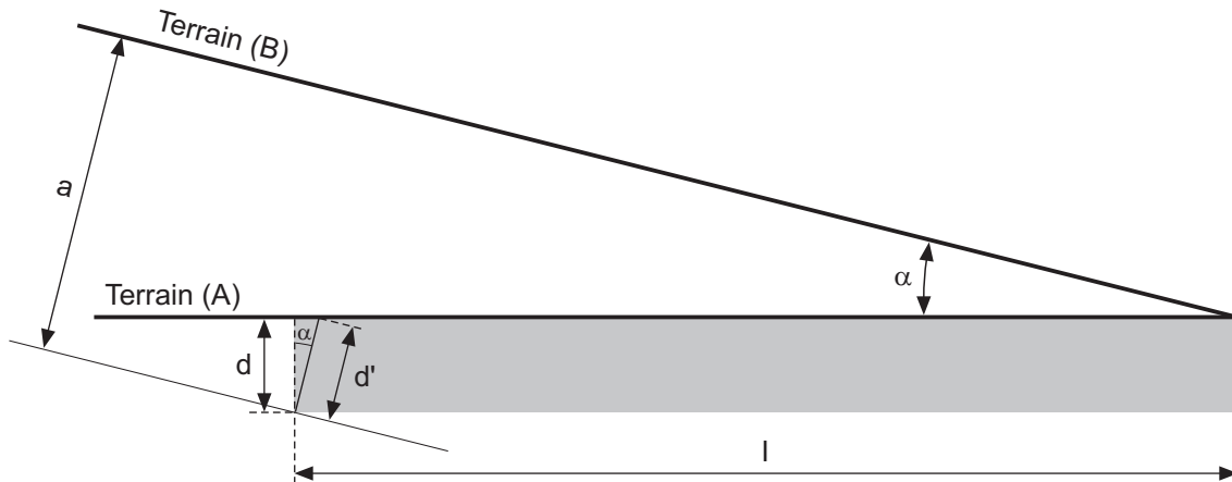
Fig. 2.5-7: Modell 2: Auswirkung der Neigung des Lagers während der erosiven Freilegung.
