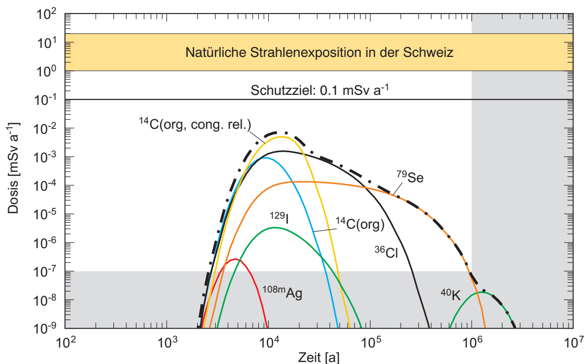
Fig. 3.3-6: Berechnete Dosen für ein SMA-Lager in einem homogen-porösen Wirtgestein (RZ).
