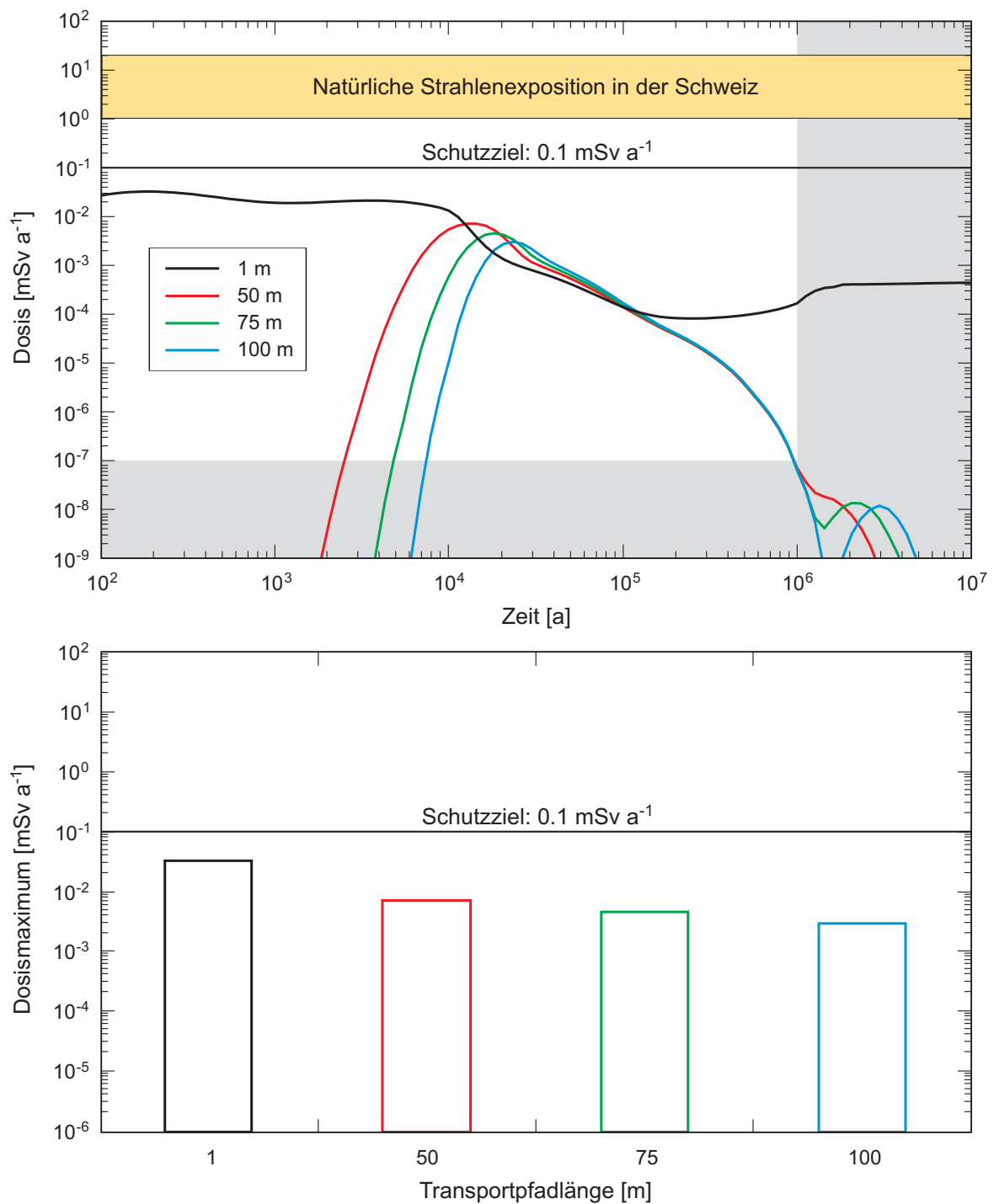
Fig. A5.3-7: Einfluss der Transportpfadlänge auf die berechneten Dosismaxima für ein SMA-Lager in einem kleinräumig geklüfteten Wirtgestein für K = 10^{-10} m/s.
