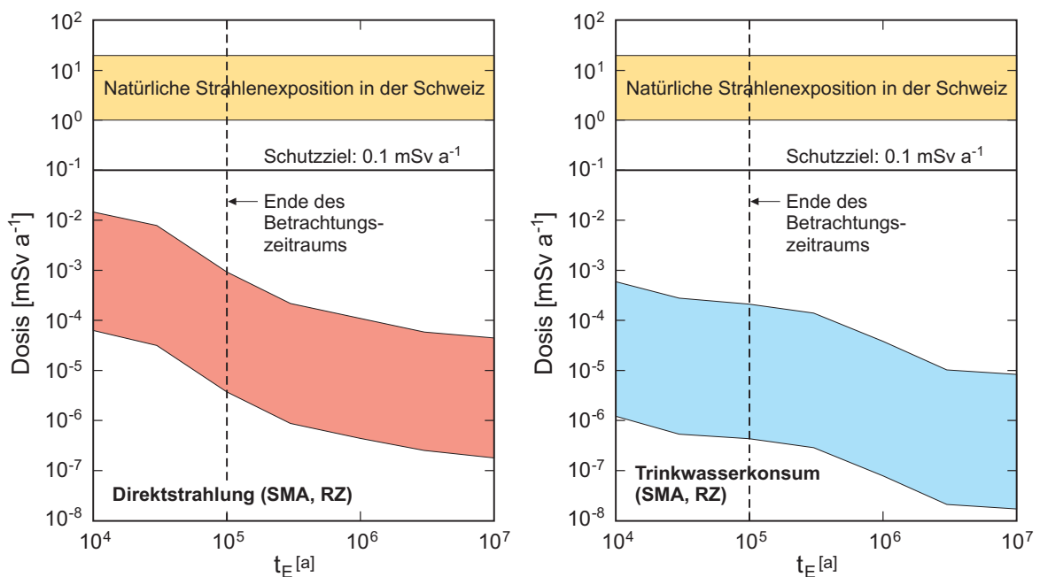
Fig. A5.4-4: Jährliche Strahlendosis gemäss Modell 2 als Funktion des Zeitpunkts der erosiven Freilegung ( t_E ) für das SMA-Lager.
