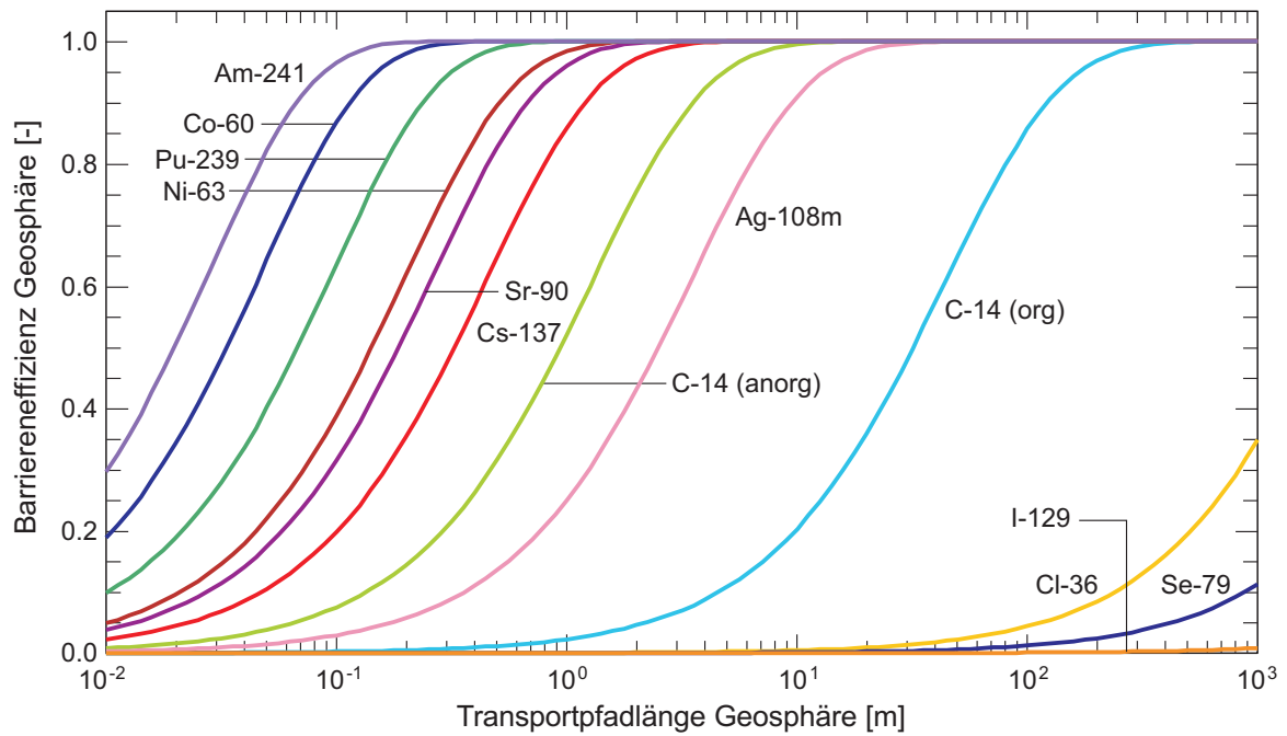
Fig. A5.5-15: Barriereneffizienz als Funktion der Transportpfadlänge (geklüftetes Wirtgestein, i = 0.1 \text{ m/m} , T = 10^{-10} \text{ m}^2/\text{s} , Sorption: Calcit).
