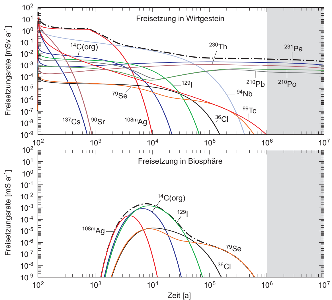
Fig. 4.7-9b: Radionuklid-Transferraten für LMA für K = 10^{-10} m/s.
