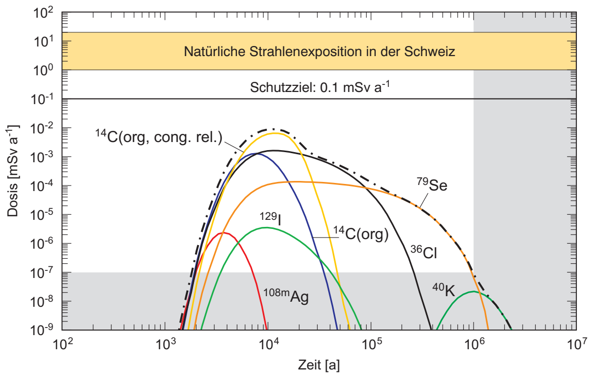
Fig. 4.7-6b: Berechnete Dosen für ein SMA-Lager in einem homogen-porösen Wirtgestein für K = 10^{-10} m/s.
