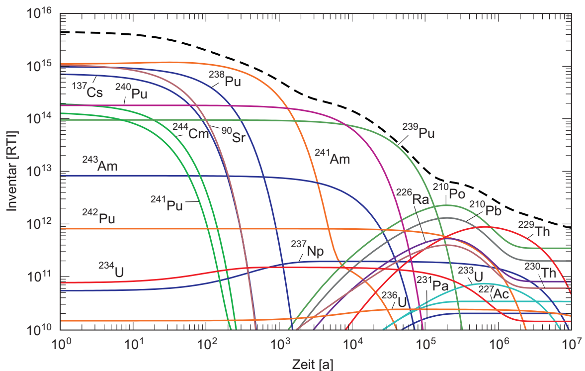
Fig. A5.5-1: Radiotoxizität als Funktion der Zeit für abgebrannte Brennelemente.
