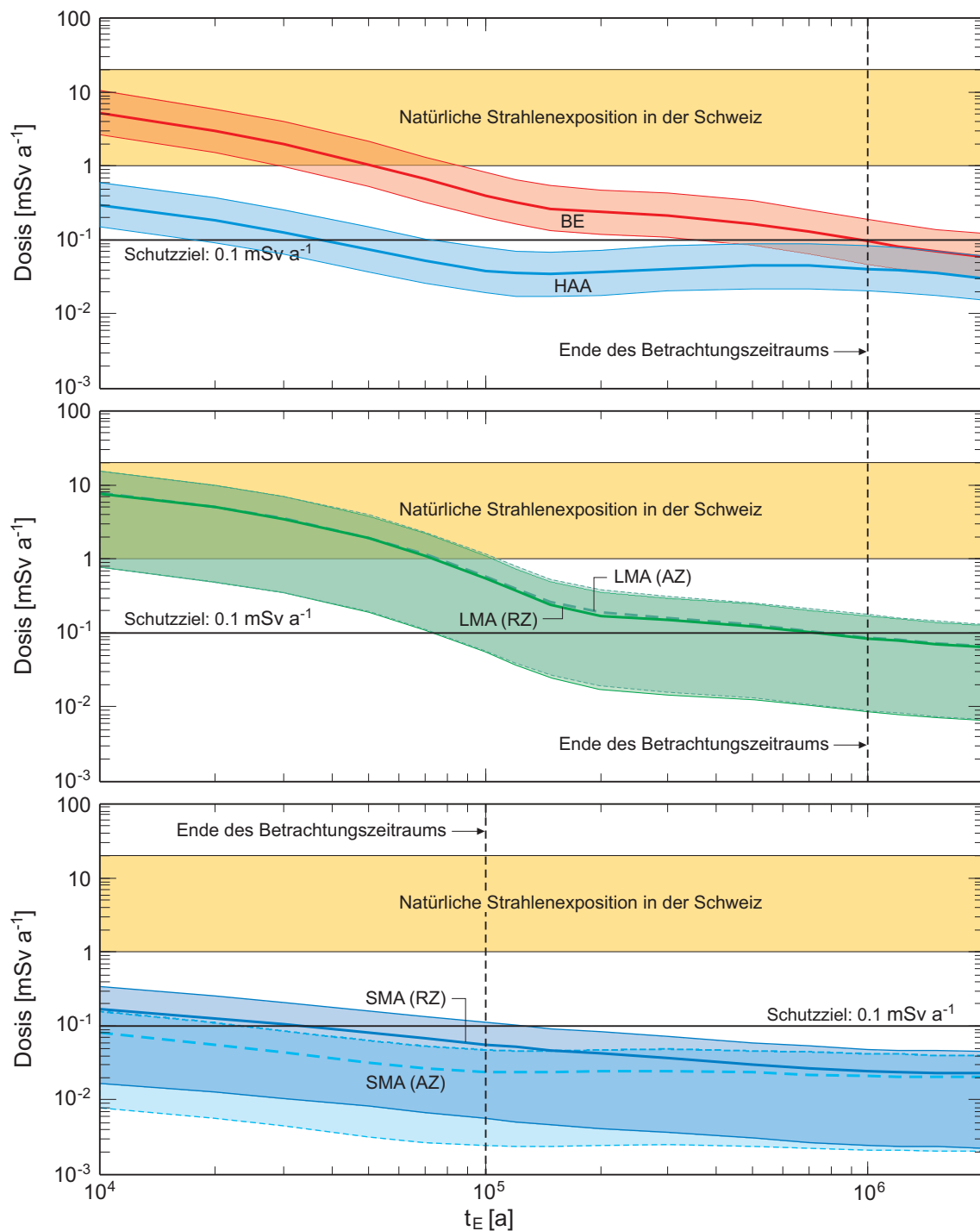
Fig. A5.4-1: Jährliche Strahlendosis gemäss Modell 1 als Funktion des Zeitpunkts t_E , nach welchem das Lager in den Einflussbereich der Erdoberfläche gelangt.
