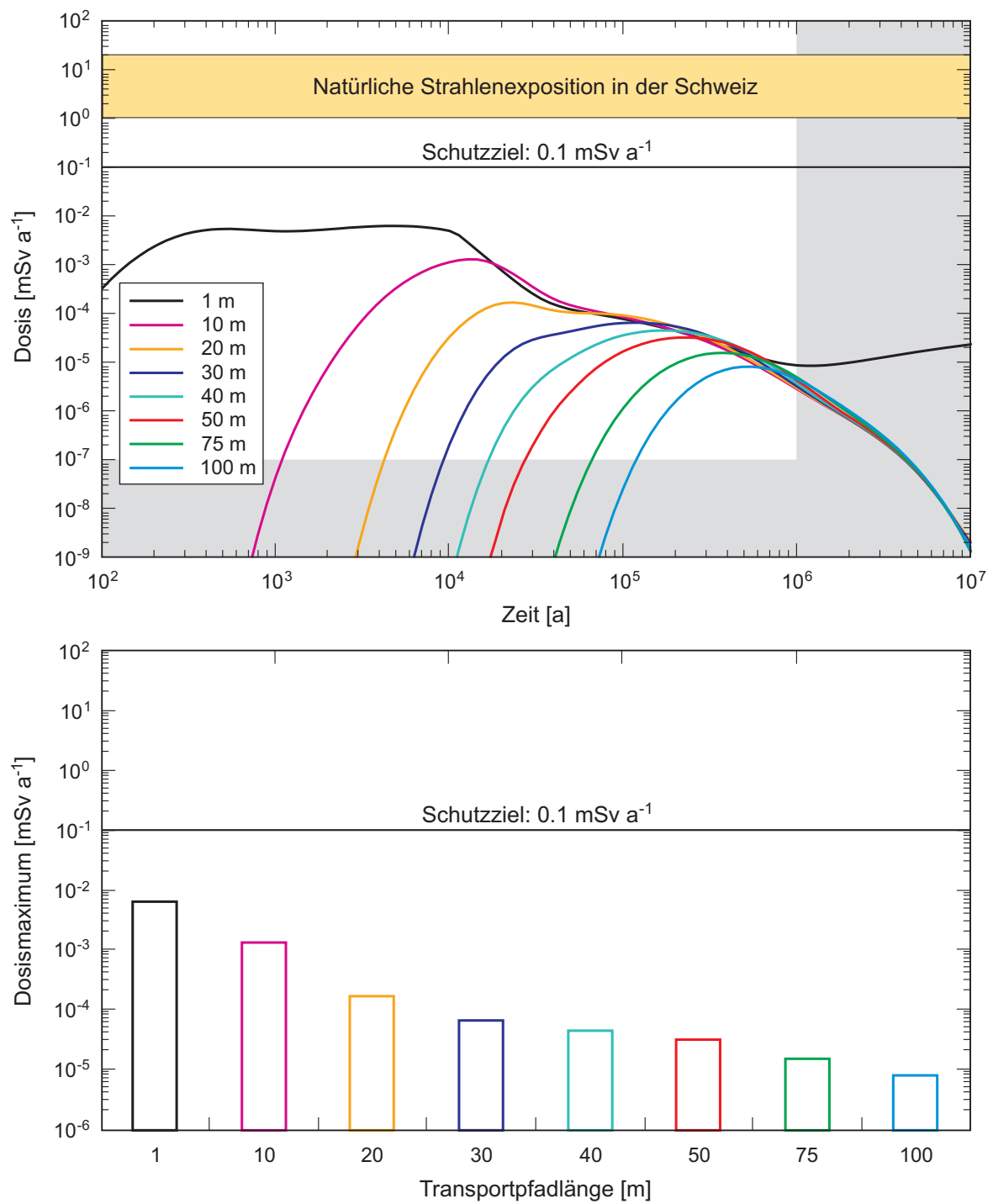
Fig. A5.3-5: Einfluss der Transportpfadlänge auf die berechneten Dosismaxima für ein SMA-Lager in einem homogen-porösen Wirtgestein für K = 10^{-13} m/s.
