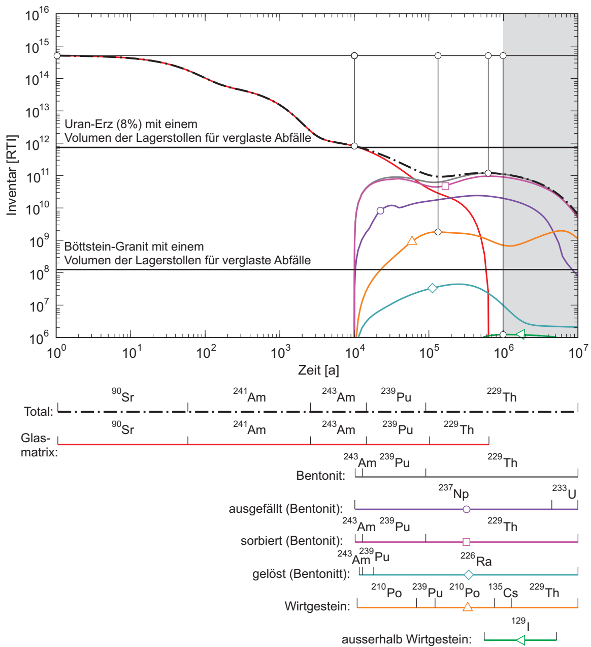
Fig. 4.7-2a: Entwicklung und Aufteilung der Radiotoxizität für verglaste hochaktive Abfälle auf die verschiedenen Komponenten des Nahfelds, das Wirtgestein und das Gebiet ausserhalb des Wirtgesteins für K = 10^{-13} m/s.
