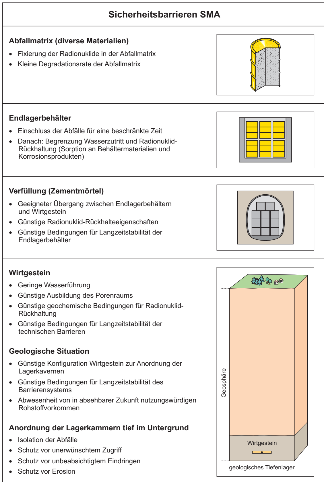
Fig. 4.3-3: Referenz-Barrierenkonzept für schwach- und mittelaktive Abfälle (SMA).
