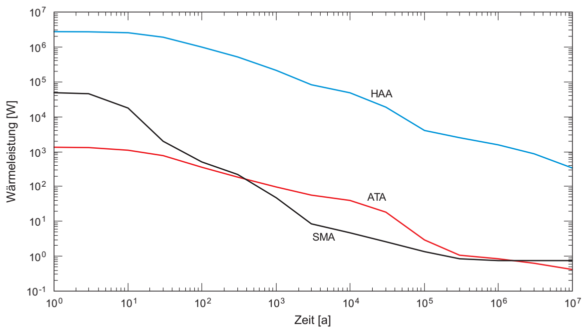
Fig. 3.2-3a: Zeitliche Entwicklung der Wärmeleistung der Abfallkategorien gemäss Definition KEV.
