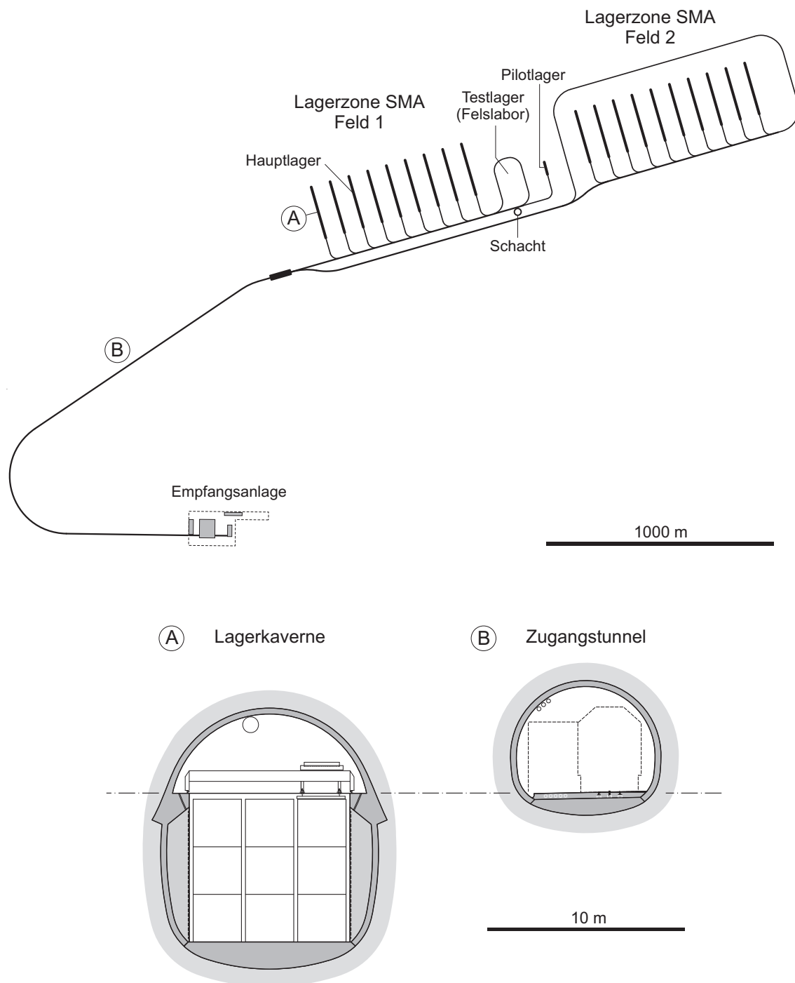
Fig. A2.6-2: Modellhafter Grundriss einer Lagerkonfiguration für ein SMA-Lager mit dem Kavernentyp K09 für das umhüllende Abfallinventar.
