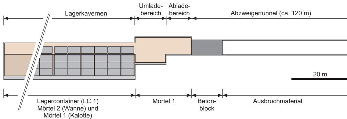
Fig. A2.3-2: Modellhaftes Konzept für SMA-Lagerkaverne des Typs K09 (Längsschnitt).
