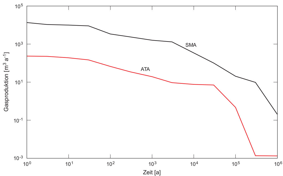
Fig. 3.2-4a: Zeitliche Entwicklung der Gasbildungsrate für ATA und SMA gemäss KEV.
