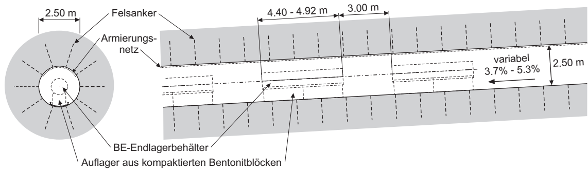
Fig. A2.3-1: Modellhaftes Konzept für BE/HAA-Lagerstollen.
