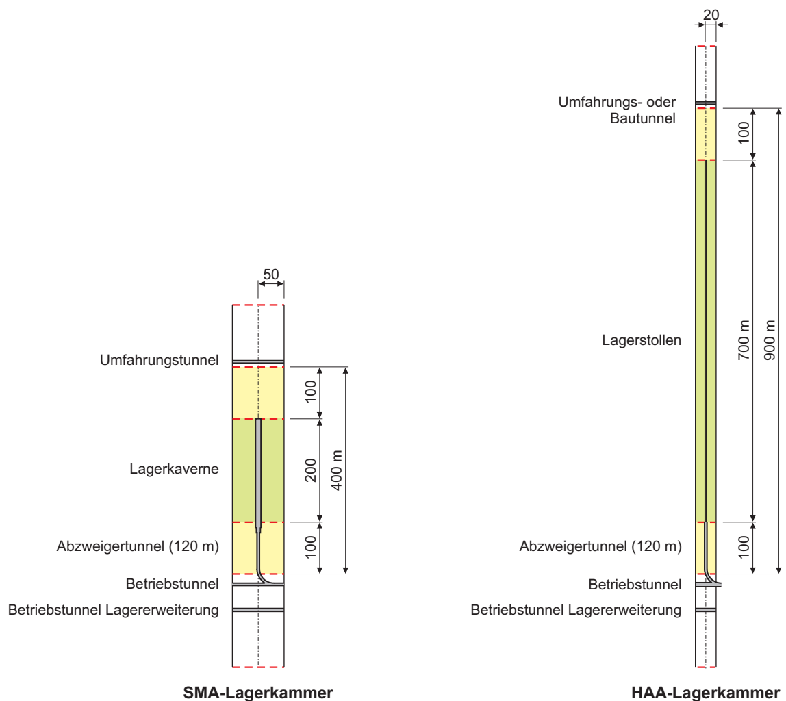
Fig. A2.4-2: Bevorzugte Lagerfeldbreite für SMA-Lagerkavernen und BE/HAA-Lagerstollen.
