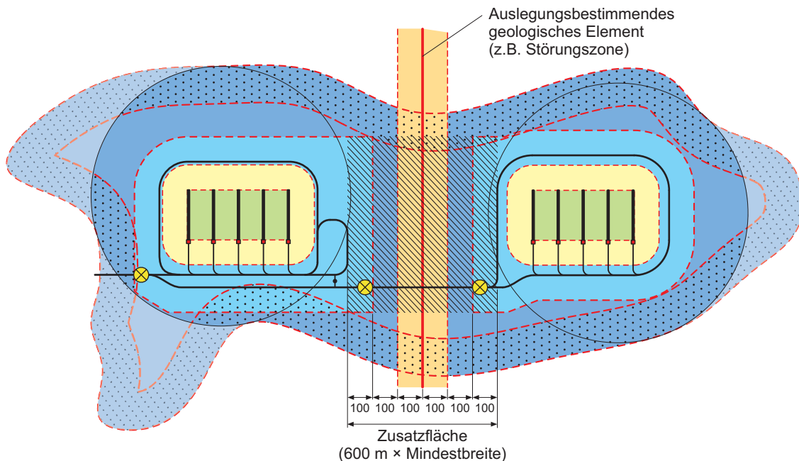
Fig. A2.6-3: Schematische Darstellung (beispielhaft) der Lagerzone für das SMA- bzw. das HAA-Lager bei ungünstiger geologischer Konfiguration infolge einer auslegungsbestimmenden Störungzone.
