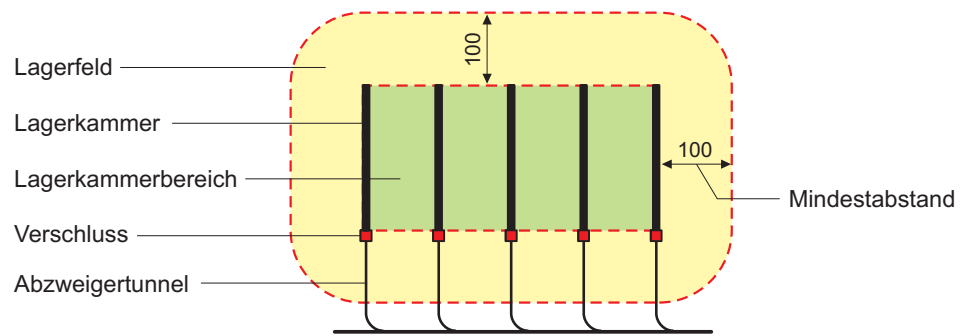
Fig. A2.4-1: Schematische Darstellung des Lagerfelds (Grundriss) mit seinen wichtigsten Elementen für das SMA- bzw. das HAA-Lager
