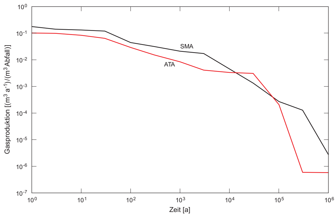
Fig. 3.2-4b: Zeitliche Entwicklung der spezifischen Gasbildungsrate für ATA und SMA gemäss KEV pro Kubikmeter verpacktes Volumen.
