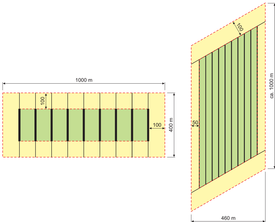
Fig. A2.6-5: Grundmodul SMA (links) und HAA (rechts).
