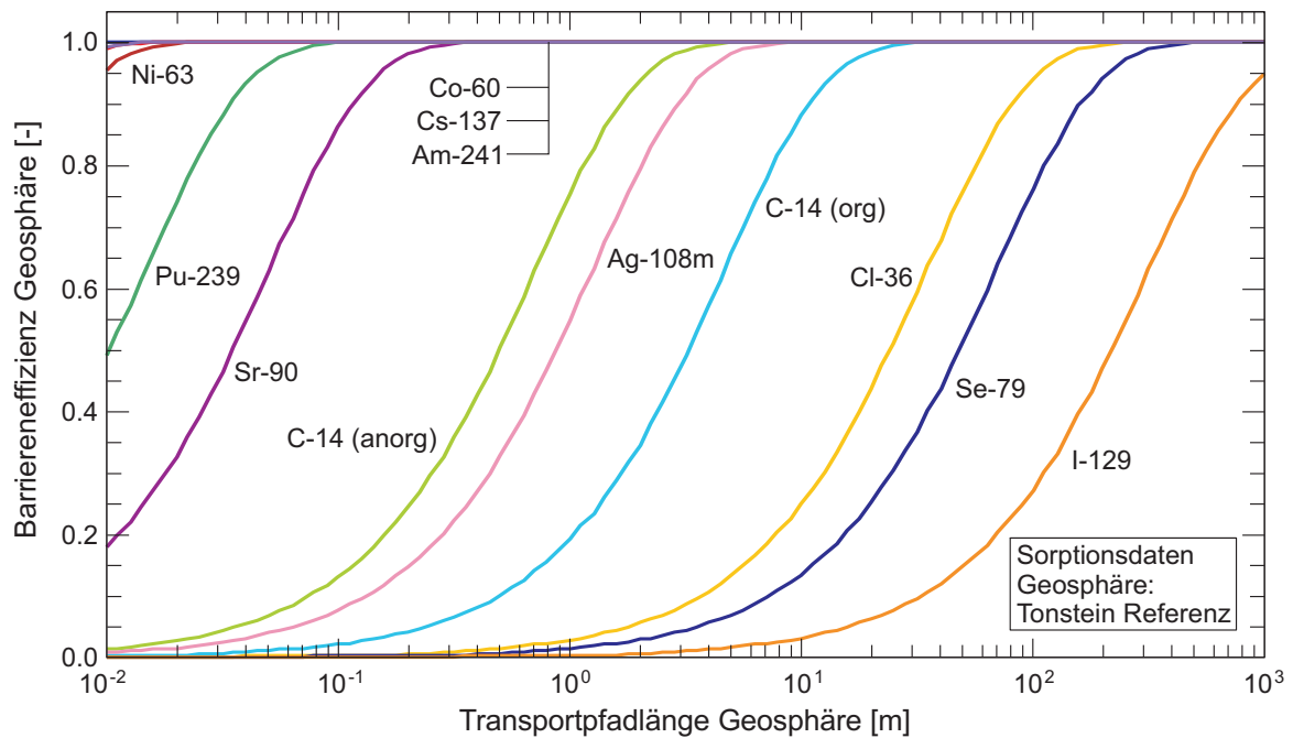
Fig. A5.5-9: Barriereneffizienz als Funktion der Transportpfadlänge (homogen-poröses Wirtgestein, i = 0.1 m/m, K = 10^{-13} m/s, Sorption: Tonstein).
