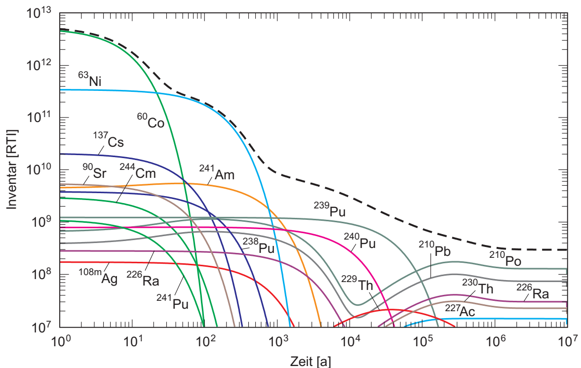
Fig. A5.5-4: Radiotoxizität als Funktion der Zeit für SMA (Referenzzuteilung).
