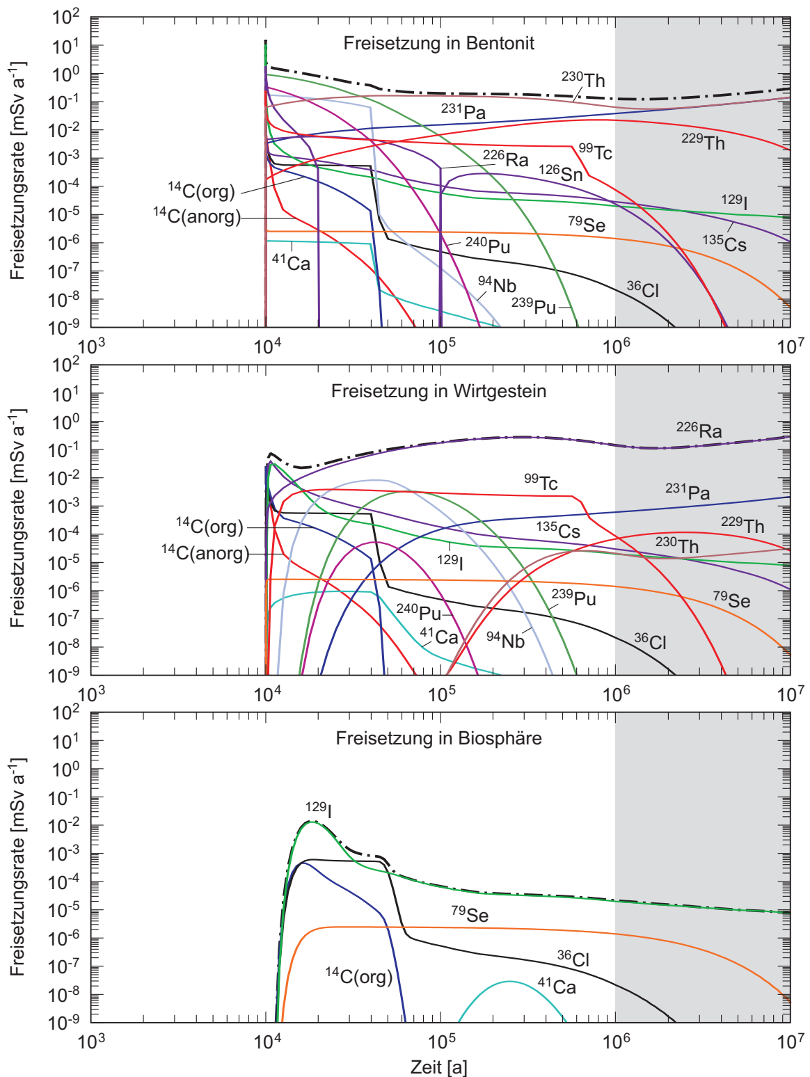
Fig. 4.7-7b: Radionuklid-Transferraten für abgebrannte Brennelemente für K = 10^{-10} m/s.
