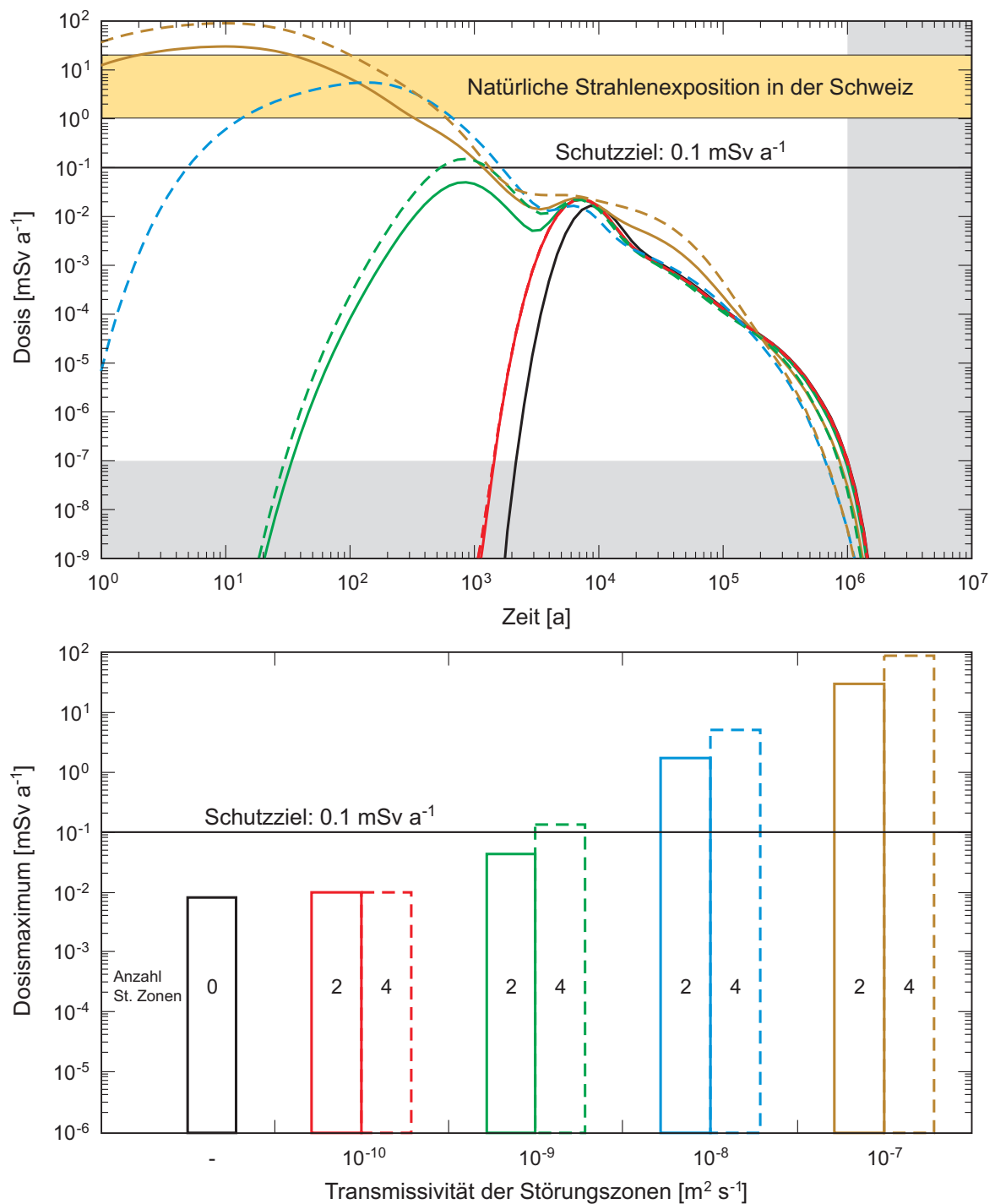
Fig. A5.2-6: Einfluss der Anzahl und Transmissivität von Störungszonen senkrecht zur Tunnelachse auf die berechneten Dosismaxima für das LMA-Lager in einem homogen-porösen Wirtgestein.
