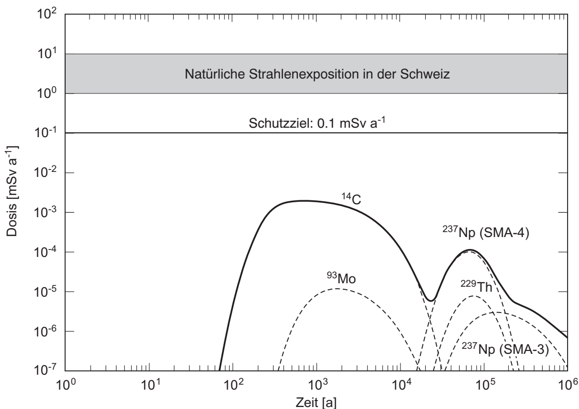
Fig. 2.4-1: Zeitlicher Verlauf der im Projekt Wellenberg für ein SMA-Lager berechneten Gesamtdosis für den Referenzfall.
