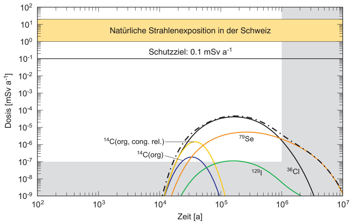
Fig. 4.7-6a: Berechnete Dosen für ein SMA-Lager in einem homogen-porösen Wirtgestein für K = 10^{-13} m/s.
