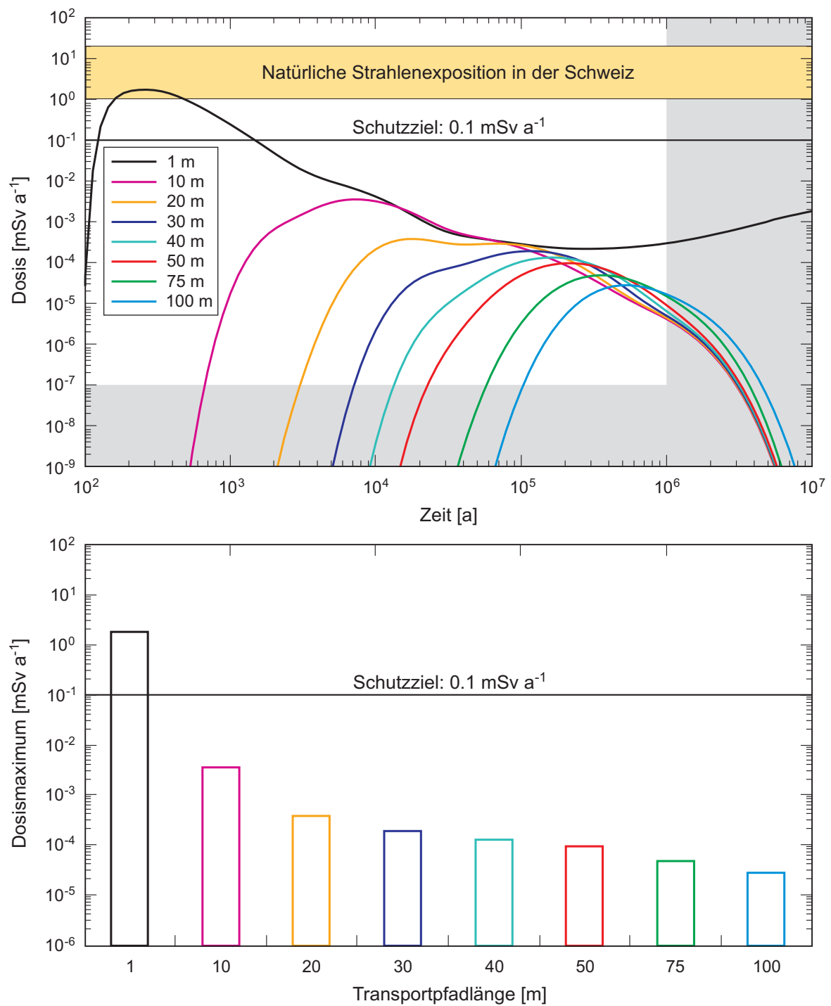
Fig. A5.3-3: Einfluss der Transportpfadlänge auf die berechneten Dosismaxima für ein HAA-Lager (LMA) in einem homogen-porösen Wirtgestein für K = 10^{-13} m/s.
