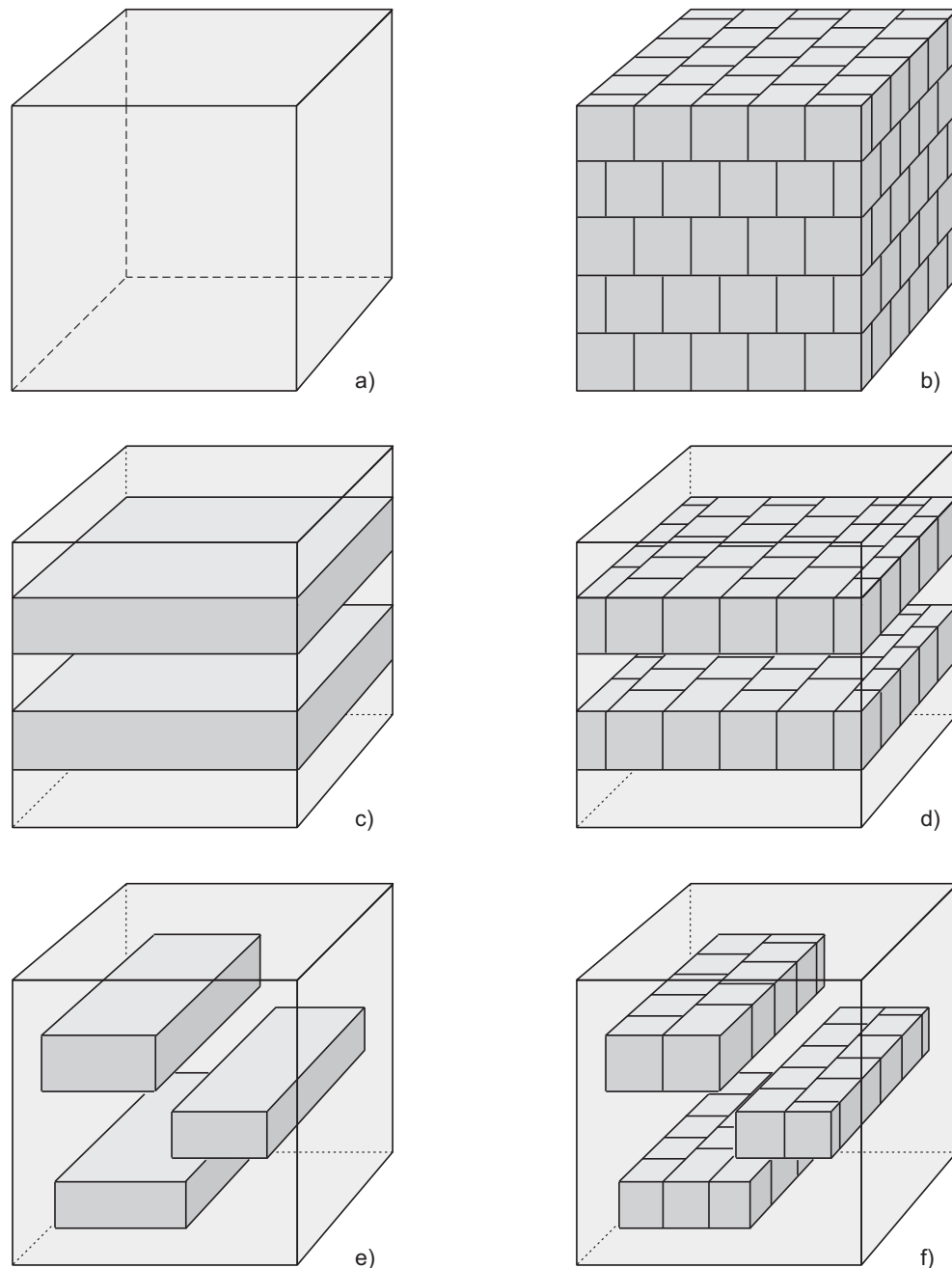
Fig. 2.5-3 Verschiedene Konzeptualisierungen des Wirtgesteins (WG) bzw. des einschlusswirksamen Gebirgsbereichs (EG).
