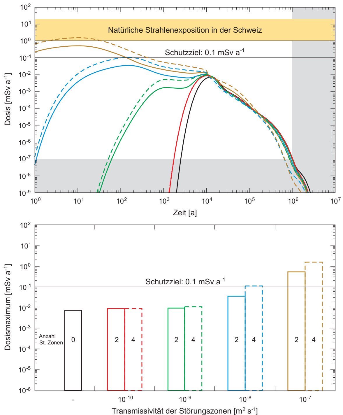
Fig. A5.2-4: Einfluss der Anzahl und Transmissivität von Störungszonen senkrecht zur Achse der Lagerkavernen auf die berechneten Dosismaxima für das SMA-Lager in einem homogen-porösen Wirtgestein.
