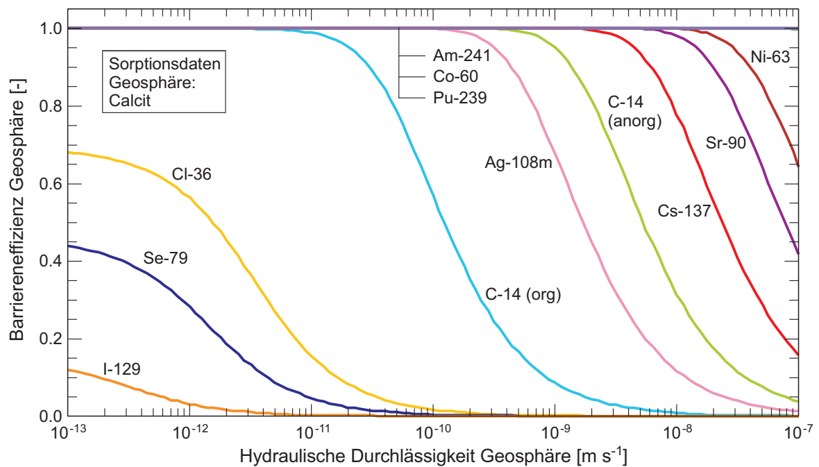
Fig. A5.5-6: Barriereffizienz als Funktion der hydraulischen Durchlässigkeit (homogenporöses WG, i = 0.1 \text{ m/m} , L = 40 \text{ m} , Sorption: Calcit).
