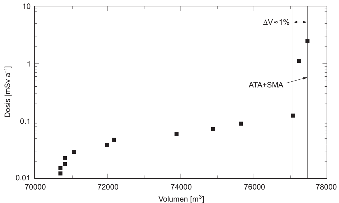
Fig. 3.2-5a: Berechnete Dosis als Funktion des Abfallvolumens im SMA-Lager für ein homogen-poröses Wirtgestein ohne Störungzonen.
