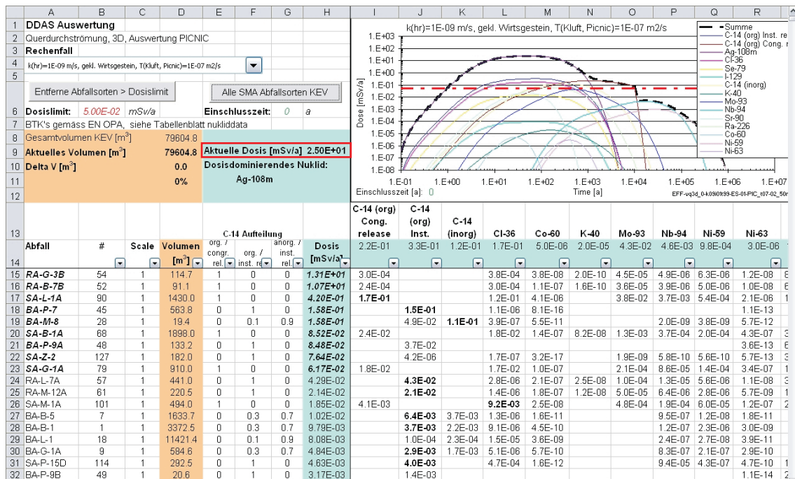
Fig. A4.5-1: Auswertung der dosisdominierenden Abfallsorten: Beispiel einer Berechnung der abfallsorten- und rechenfallspezifischen Dosisbeiträge.
