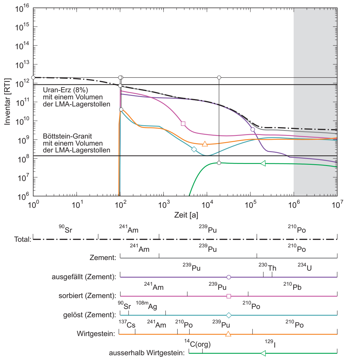
Fig. 4.7-3b: Entwicklung und Aufteilung der Radiotoxizität für langlebige mittelaktive Abfälle auf die verschiedenen Komponenten des Nahfelds, das Wirtgestein und das Gebiet ausserhalb des Wirtgesteins für K = 10^{-10} m/s.
