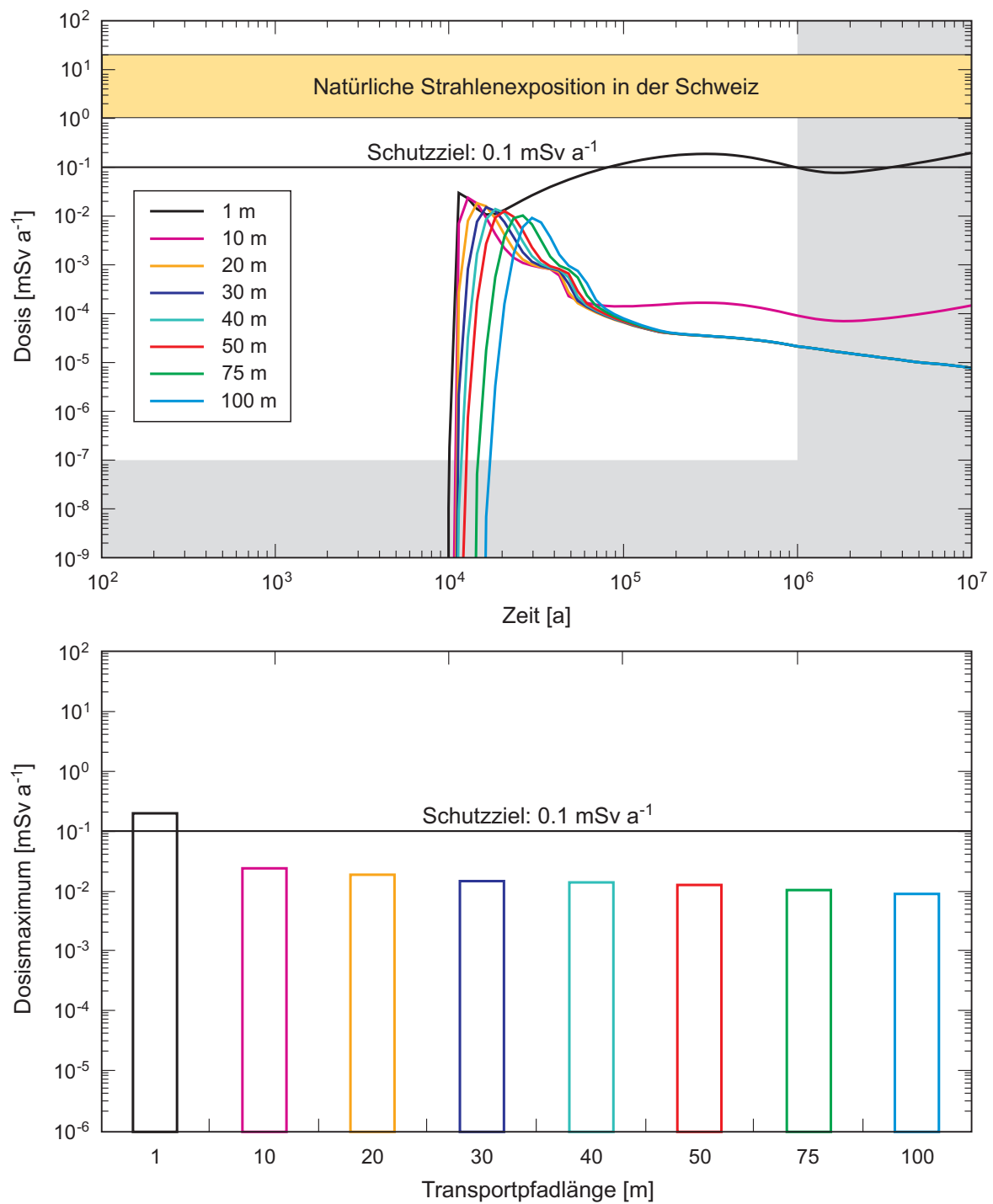
Fig. A5.3-2: Einfluss der Transportpfadlänge auf die berechneten Dosismaxima für ein HAA-Lager (BE) in einem homogen-porösen Wirtgestein für K = 10^{-10} m/s.
