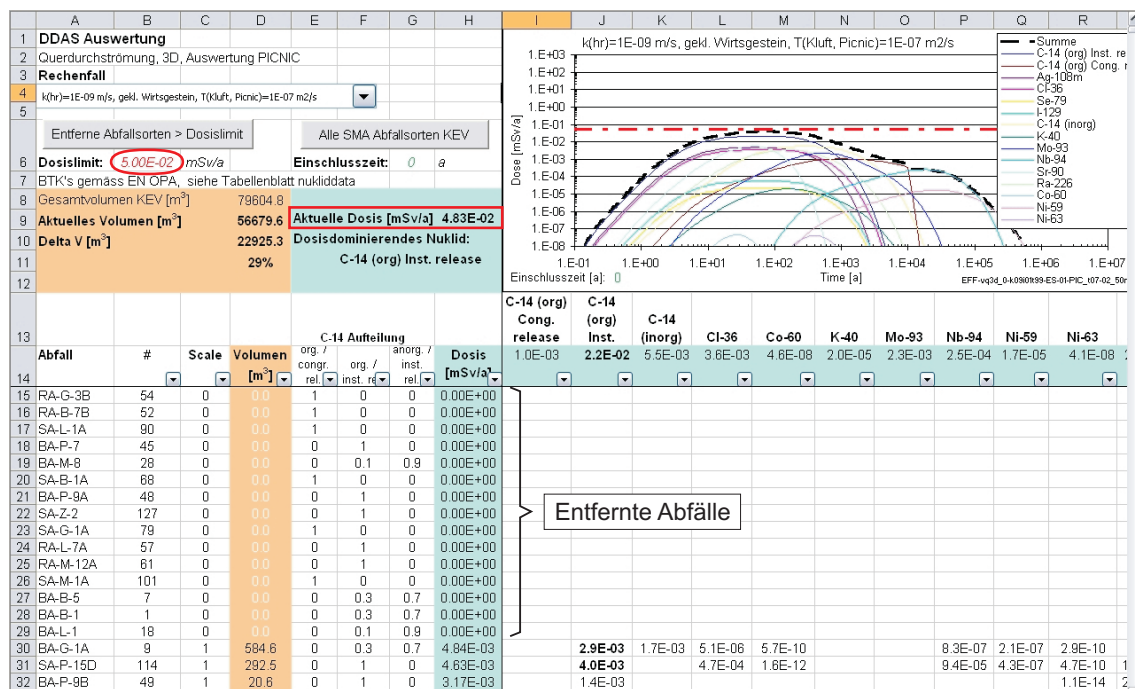
Fig. A4.5-2: Auswertung der dosisdominierenden Abfallsorten: Beispiel für das sukzessive Entfernen der Abfälle mit den grössten Dosisbeiträgen, bis ein definierter Dosisgrenzwert eingehalten wird.
