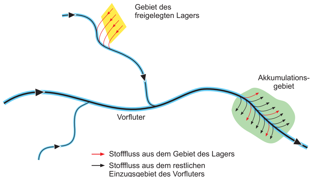
Fig. 2.5-6: Modell 2: Erosion, Verfrachtung, Verdünnung und Ablagerung von Material aus dem Gebiet des freigelegten Lagers.
