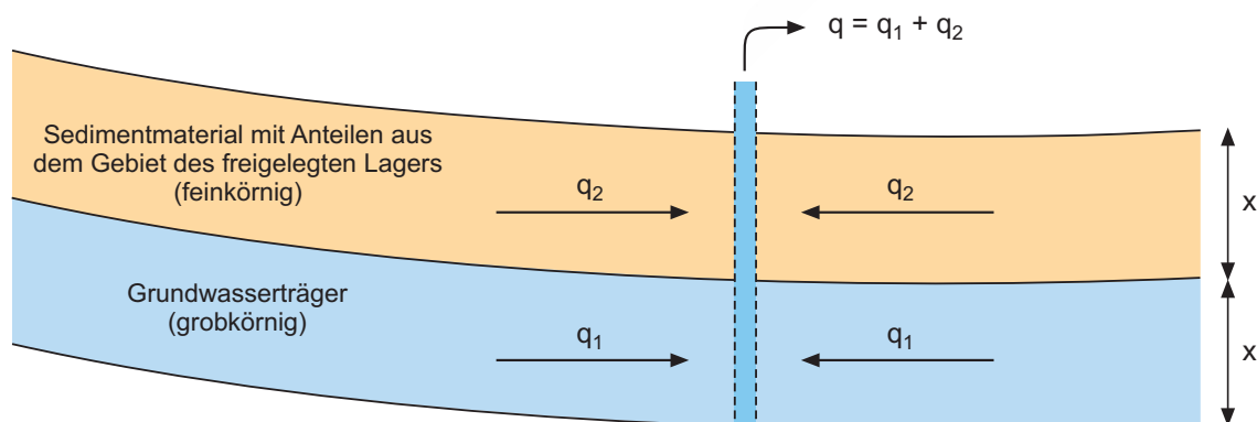
Fig. 2.5-8: Modell 2: Gewinnung und Verdünnung von Trinkwasser aus einem Grundwasserträger im Gebiet, das vom Vorfluter deponiertes radionuklidhaltiges Sedimentmaterial enthält.
