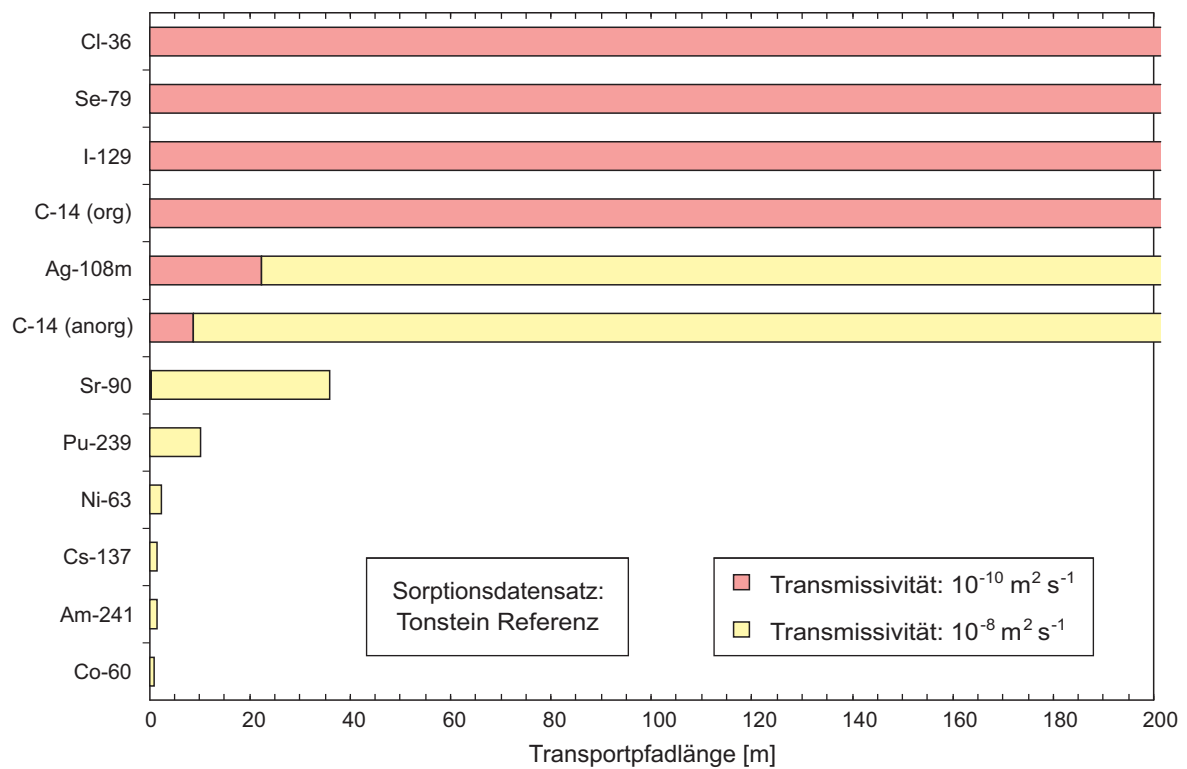
Fig. A5.5-19: Nuklidspezifische Reichweite (99 % Zerfall) in einer Kluft (Sorpton: Tonstein).
