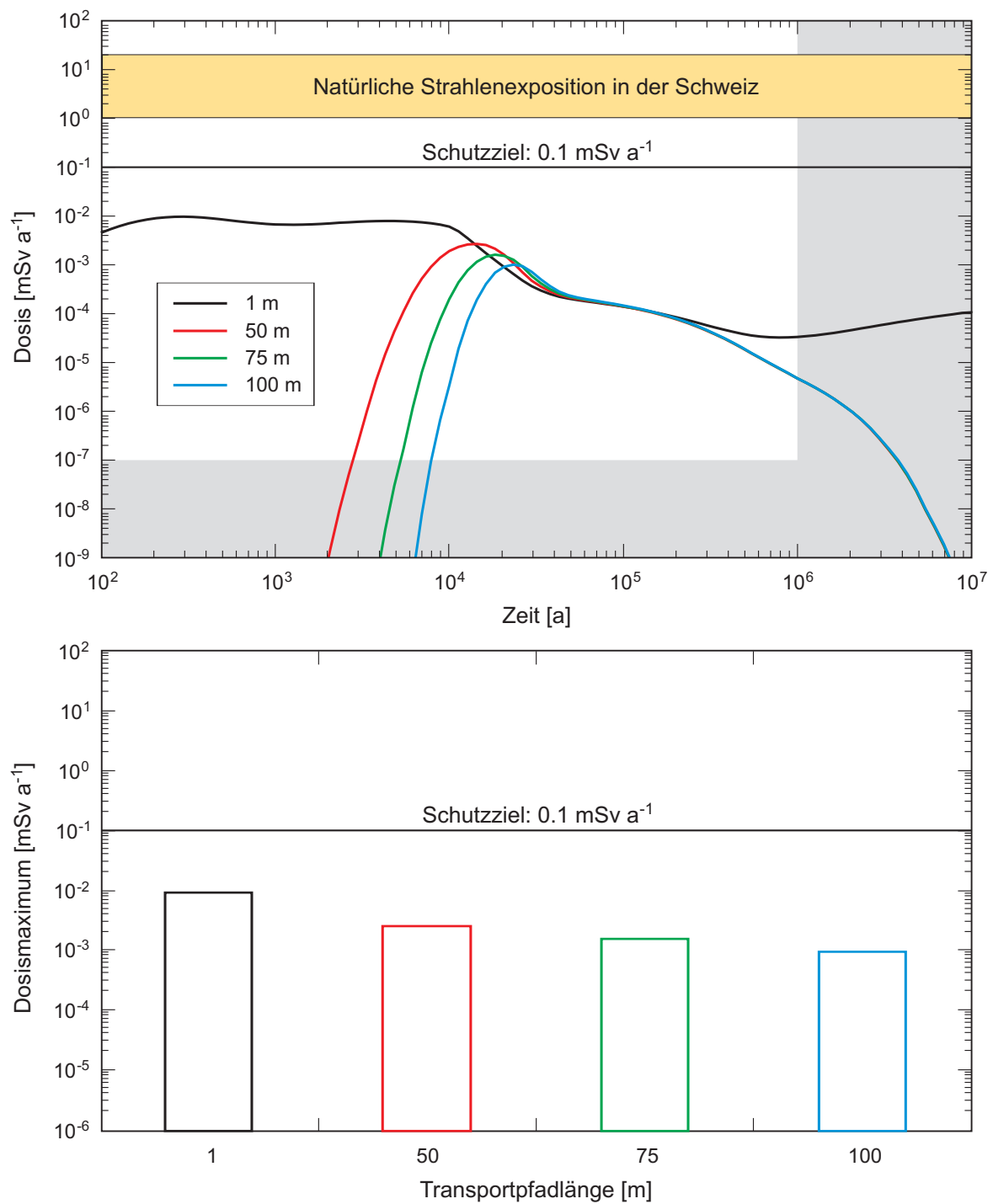
Fig. A5.3-8: Einfluss der Transportpfadlänge auf die berechneten Dosismaxima für ein SMA-Lager in einem kleinräumig geklüfteten Wirtsgestein für K = 10^{-11} \text{ m/s} .
