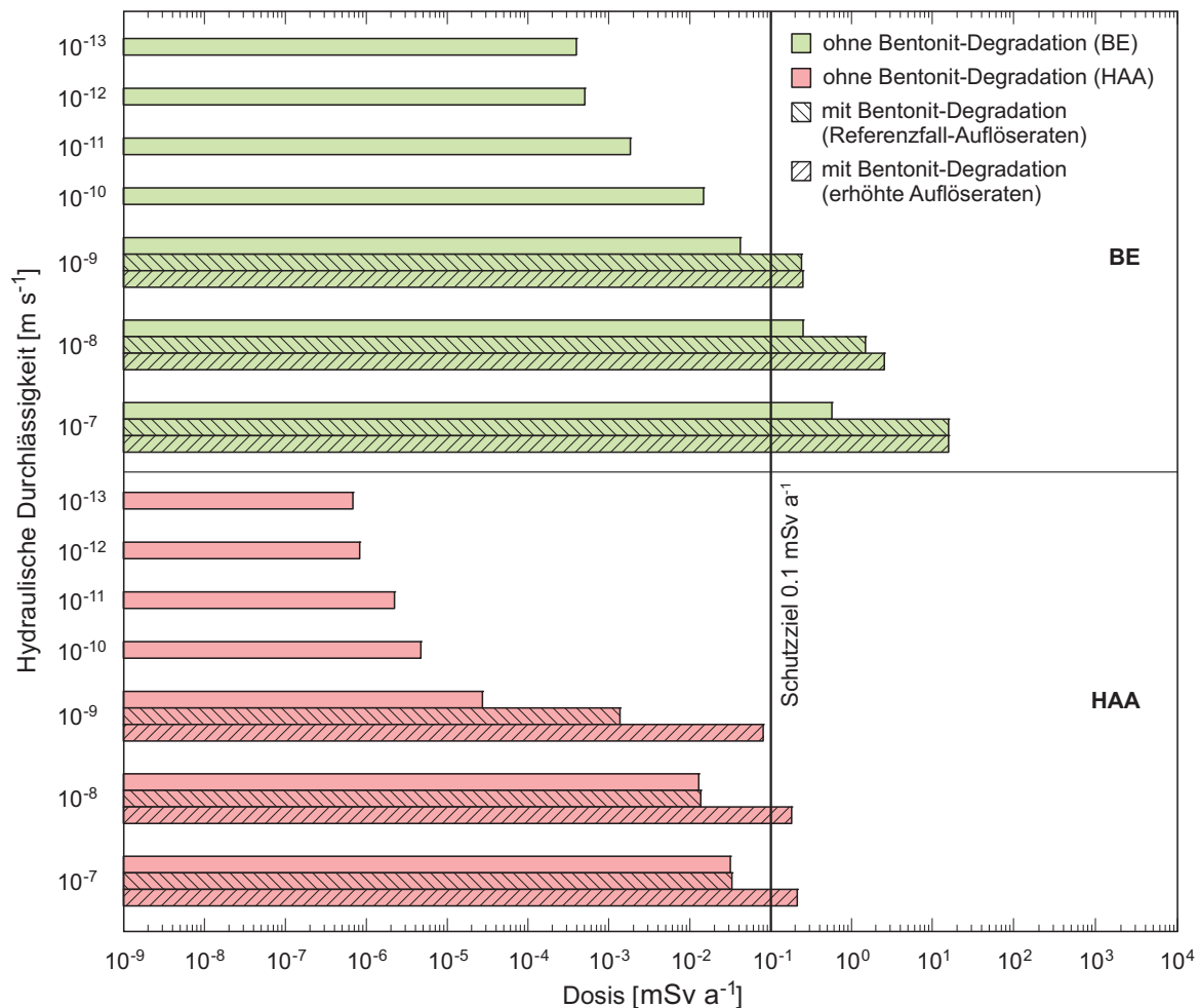
Fig. A5.2-2: Einfluss der hydraulischen Durchlässigkeit eines homogen-porösen Wirtgesteins auf die berechneten Dosismaxima für BE und HAA mit und ohne Bentonit-Degradation.
