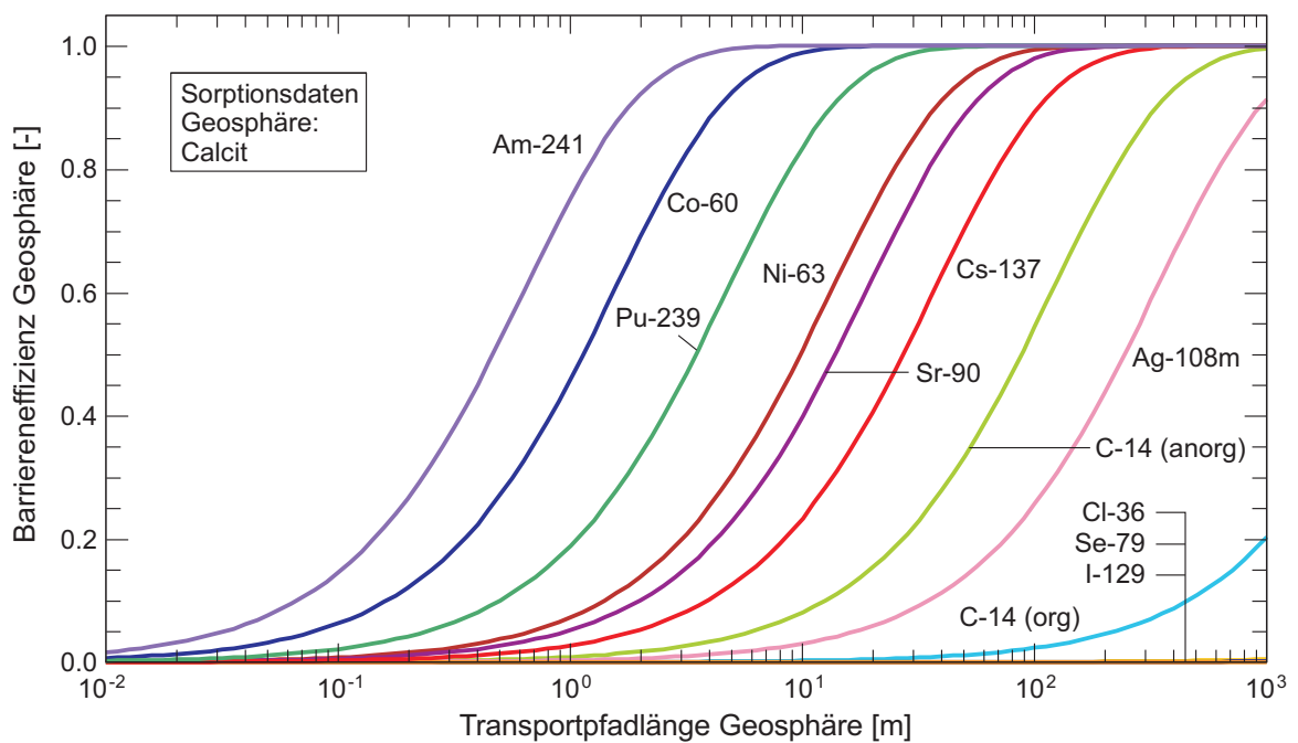
Fig. A5.5-16: Barriereneffizienz als Funktion der Transportpfadlänge (geklüftetes Wirtgestein, i = 0.1 \text{ m/m} , T = 10^{-8} \text{ m}^2/\text{s} , Sorption: Calcit).
