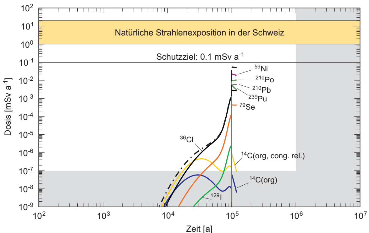
Fig. A5.4-6: Einfluss einer zeitabhängigen Dekompaktion auf ein SMA-Lager am Beispiel des Wirtgesteins Opalinuston gemäss Modell 3.
