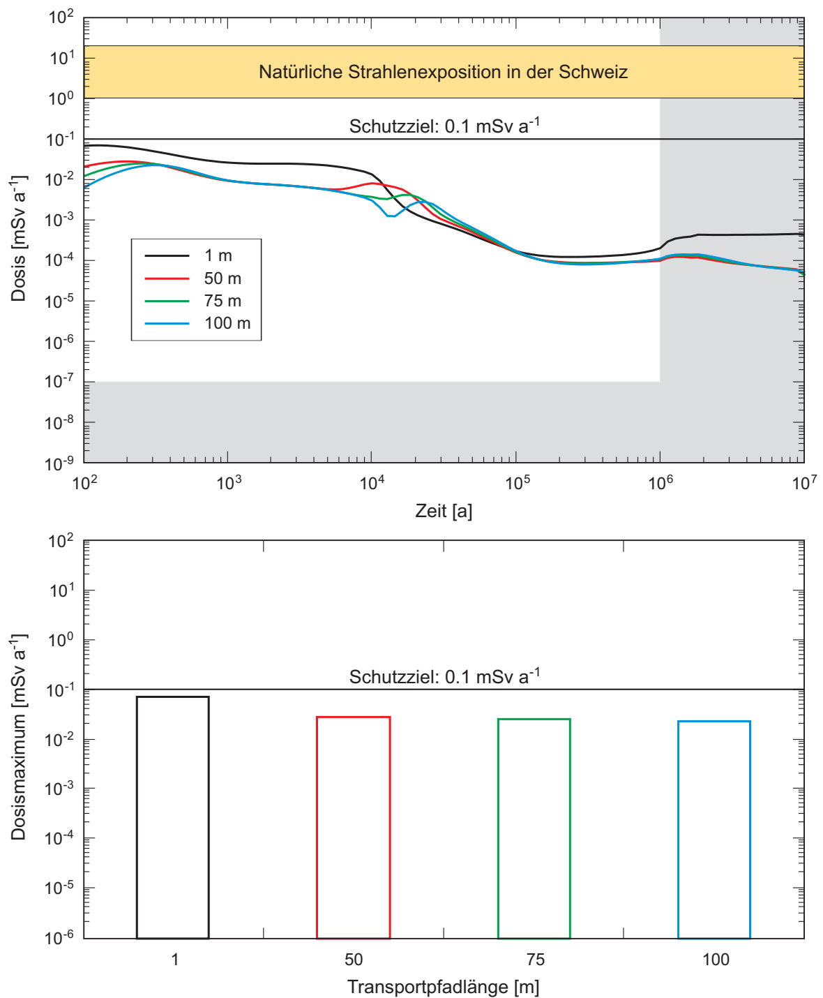
Fig. A5.3-9: Einfluss der Transportpfadlänge auf die berechneten Dosismaxima für ein SMA-Lager in einem homogen-porösen Wirtgestein mit zwei Störungzonen senkrecht zur Kavernenachse für K = 10^{-10} \text{ m/s} .
