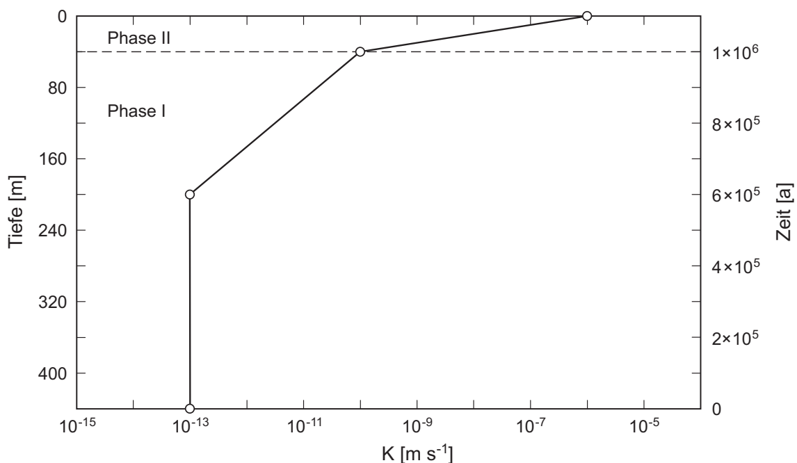
Fig. 2.5-9: Schematische Darstellung der hydraulischen Durchlässigkeit von Opalinuston als Funktion der Tiefe bzw. der Zeit für ein HAA-Lager.
