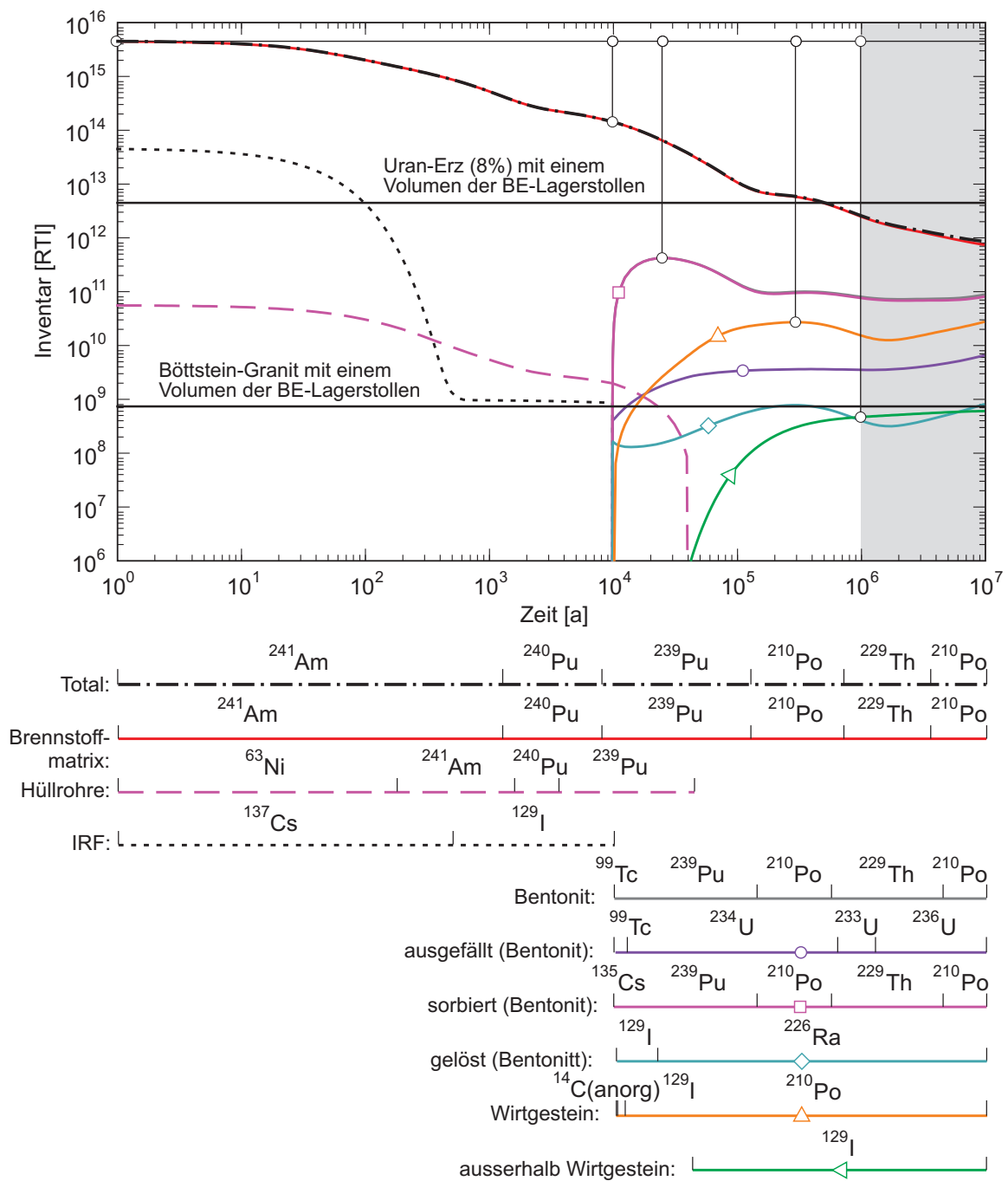
Fig. 4.7-1a: Entwicklung und Aufteilung der Radiotoxizität für abgebrannte Brennelemente auf die verschiedenen Komponenten des Nahfelds, das Wirtgestein und das Gebiet ausserhalb des Wirtgesteins für K = 10^{-13} m/s.
