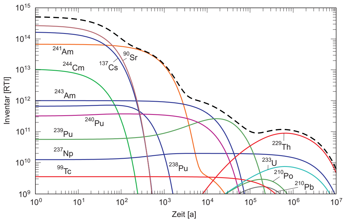
Fig. A5.5-2: Radiotoxizität als Funktion der Zeit für verglaste hochaktive Abfälle.
