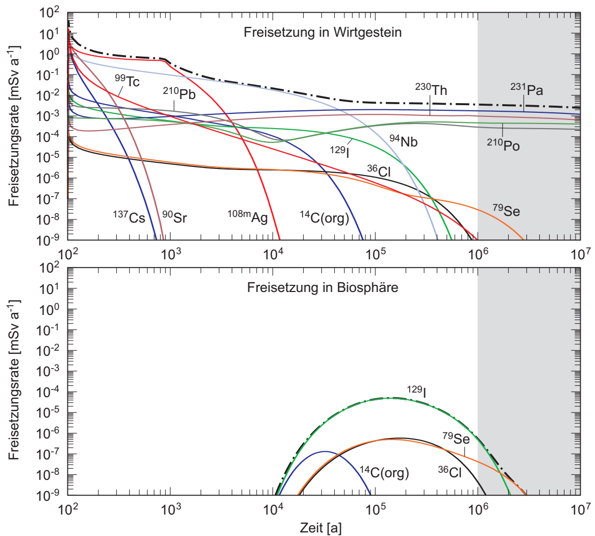
Fig. 4.7-9a: Radionuklid-Transferraten für LMA für K = 10^{-13} m/s.
