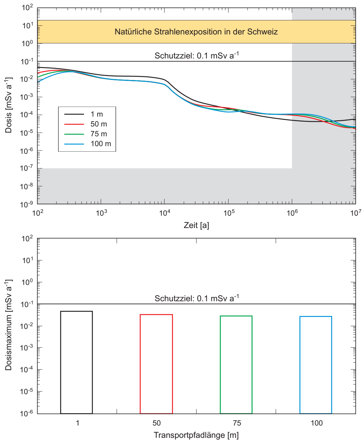
Fig. A5.3-10: Einfluss der Transportpfadlänge auf die berechneten Dosismaxima für ein SMA-Lager in einem homogen-porösen Wirtgestein mit zwei Störungzonen senkrecht zur Kavernenachse für K = 10^{-11} \text{ m/s} .
