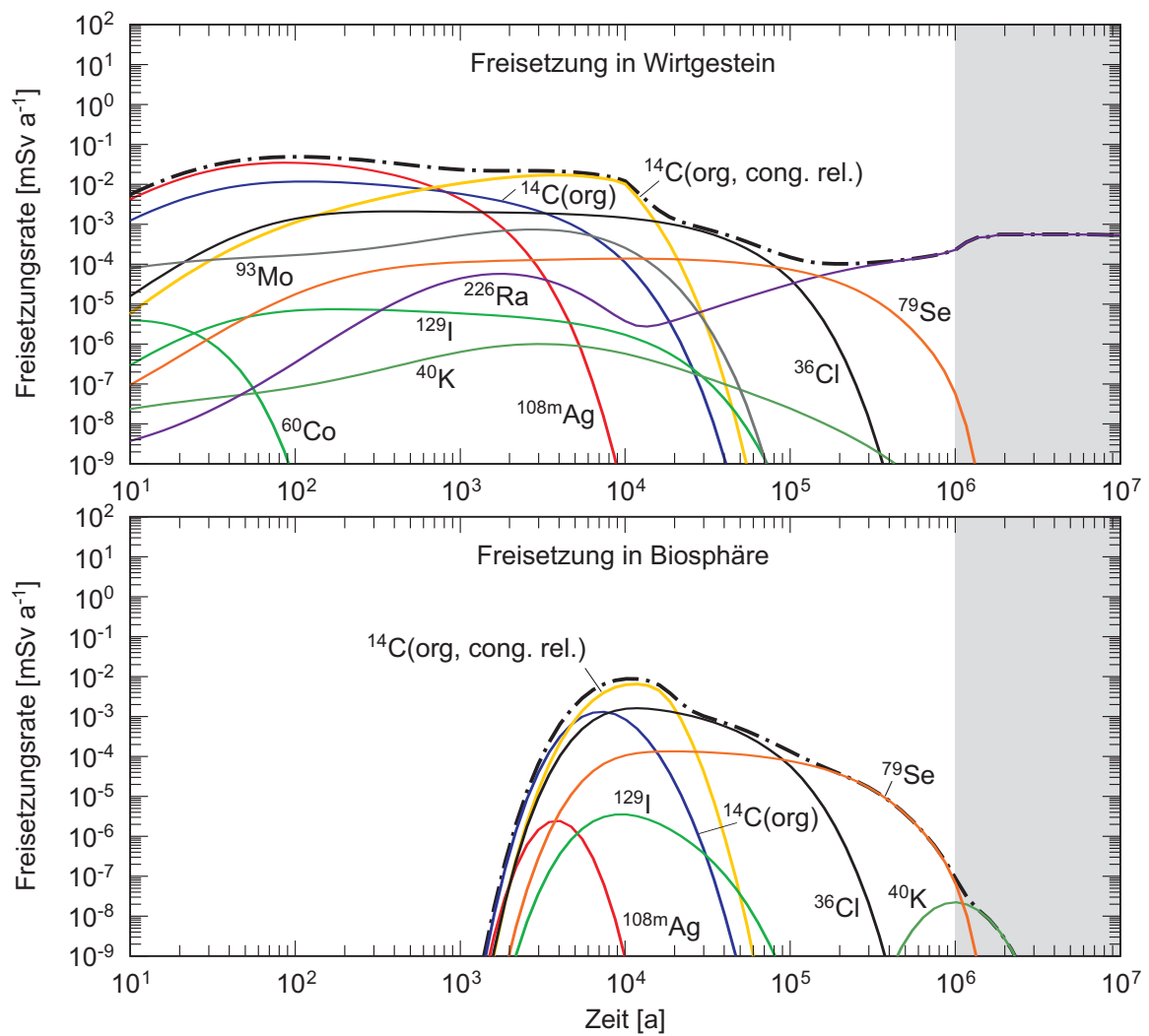
Fig. 4.7-10b: Radionuklid-Transferraten für SMA für K = 10^{-10} m/s.
