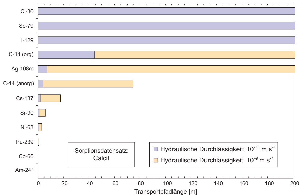
Fig. A5.5-18: Nuklidspezifische Reichweite (99 % Zerfall) im homogen-porösen Wirtgestein (Sorptions: Calcit).
