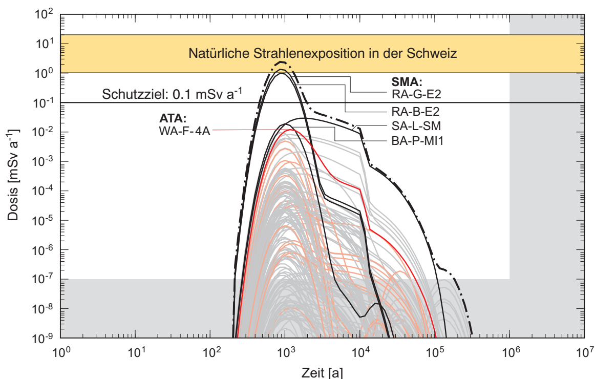
Fig. 3.2-5b: Berechnete Dosen für alle ATA- und SMA-Abfallsorten im SMA-Lager für ein homogen-poröses Wirtgestein ohne Störungzonen.
