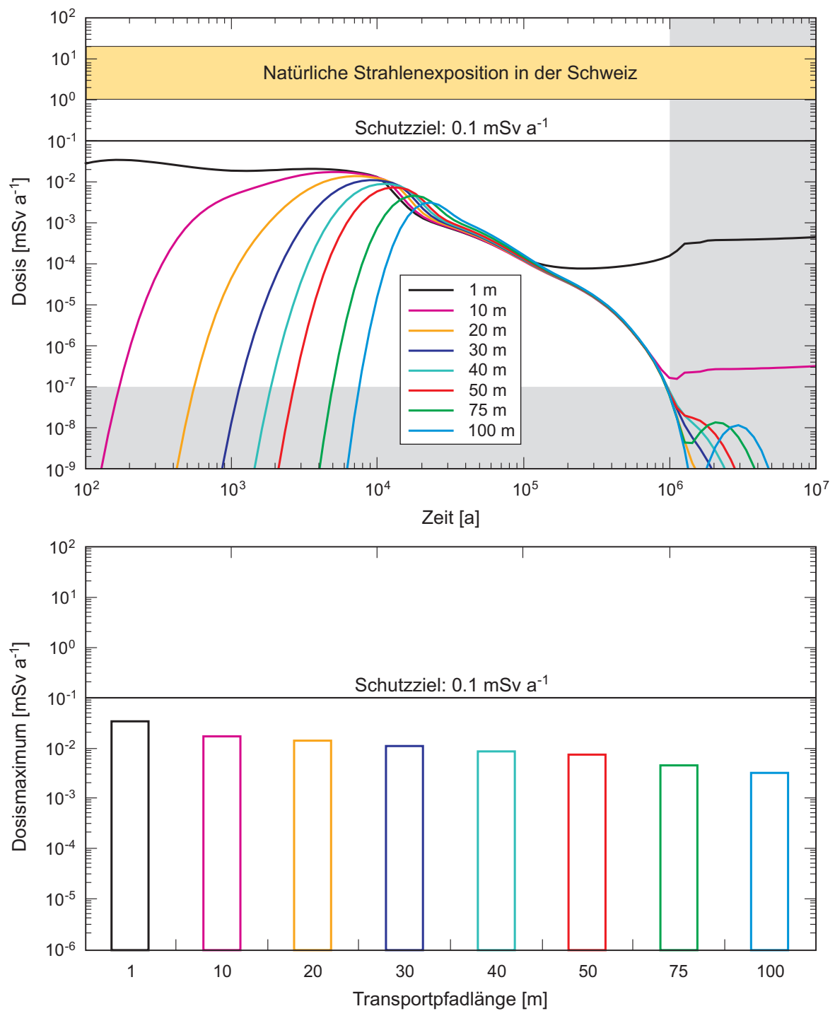
Fig. A5.3-6: Einfluss der Transportpfadlänge auf die berechneten Dosismaxima für ein SMA-Lager in einem homogen-porösen Wirtgestein für K = 10^{-10} \text{ m/s} .
