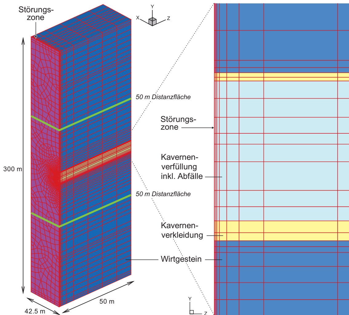
Fig. A4.3-2: Modellgeometrie für VPAC-Rechnungen (homogen-poröses Wirtgestein mit vertikalen Störungszone(n)).
