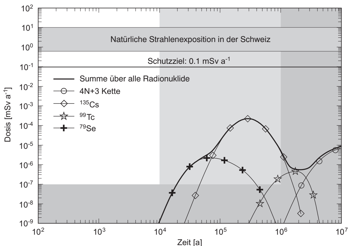
Fig. 2.4-2: Zeitlicher Verlauf der im Projekt Kristallin-I für ein HAA-Lager berechneten Gesamtdosis für den Referenzfall.
