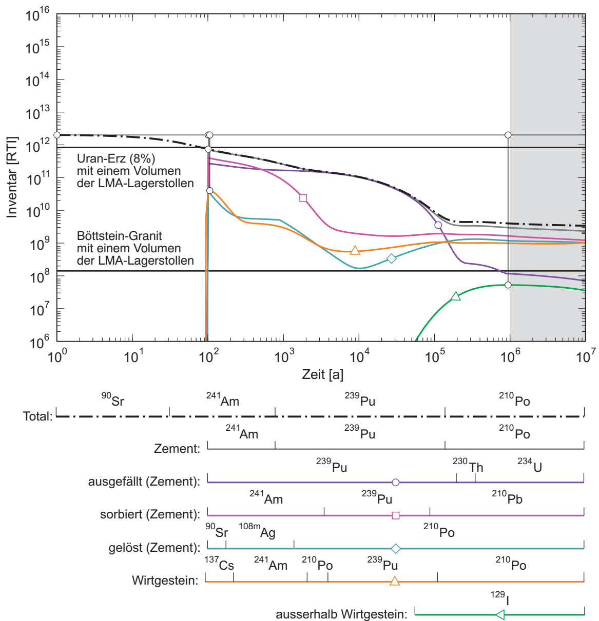
Fig. 4.7-3a: Entwicklung und Aufteilung der Radiotoxizität für langlebige mittelaktive Abfälle auf die verschiedenen Komponenten des Nahfelds, das Wirtgestein und das Gebiet ausserhalb des Wirtgesteins für K = 10^{-13} m/s.
