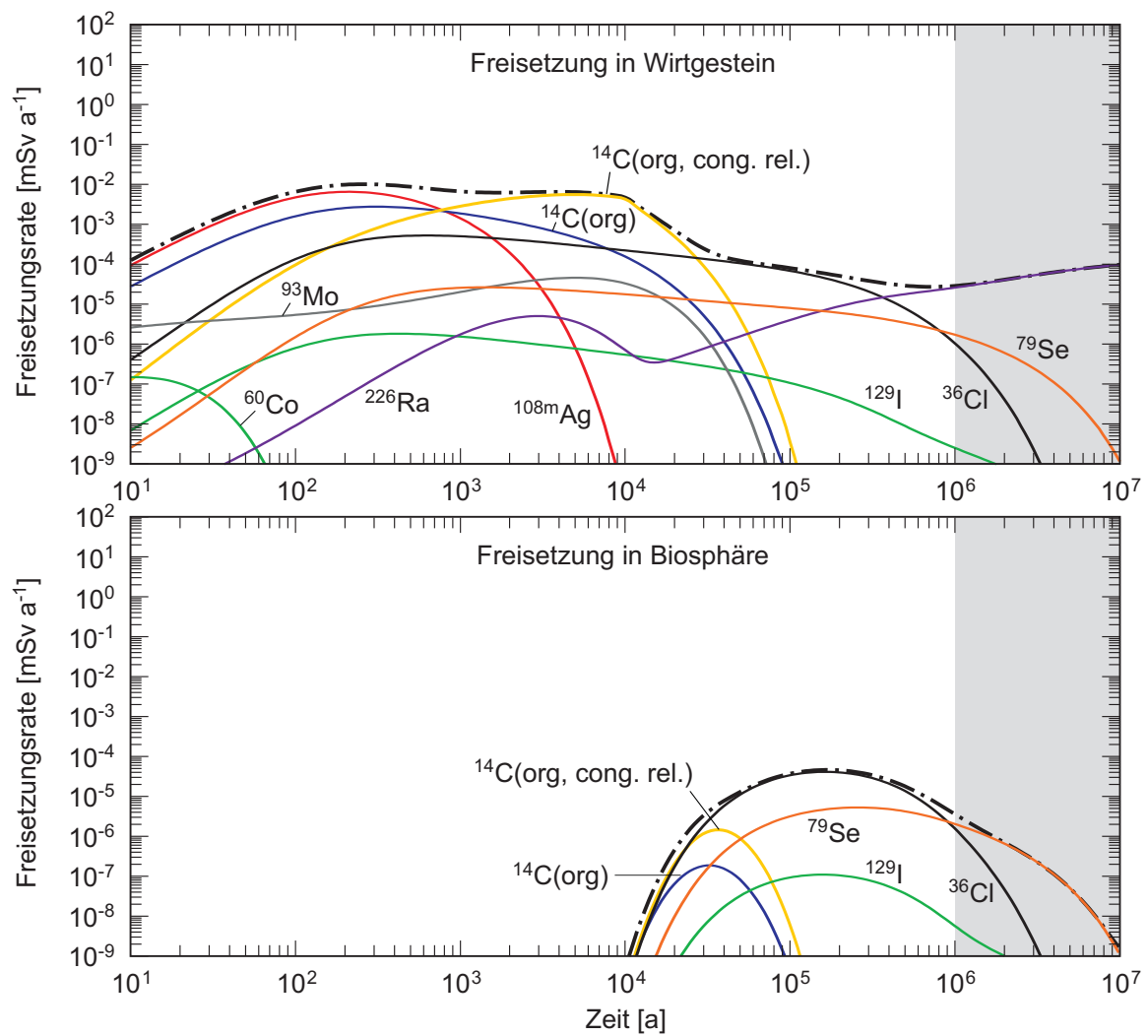
Fig. 4.7-10a: Radionuklid-Transferraten für SMA für K = 10^{-13} m/s.
