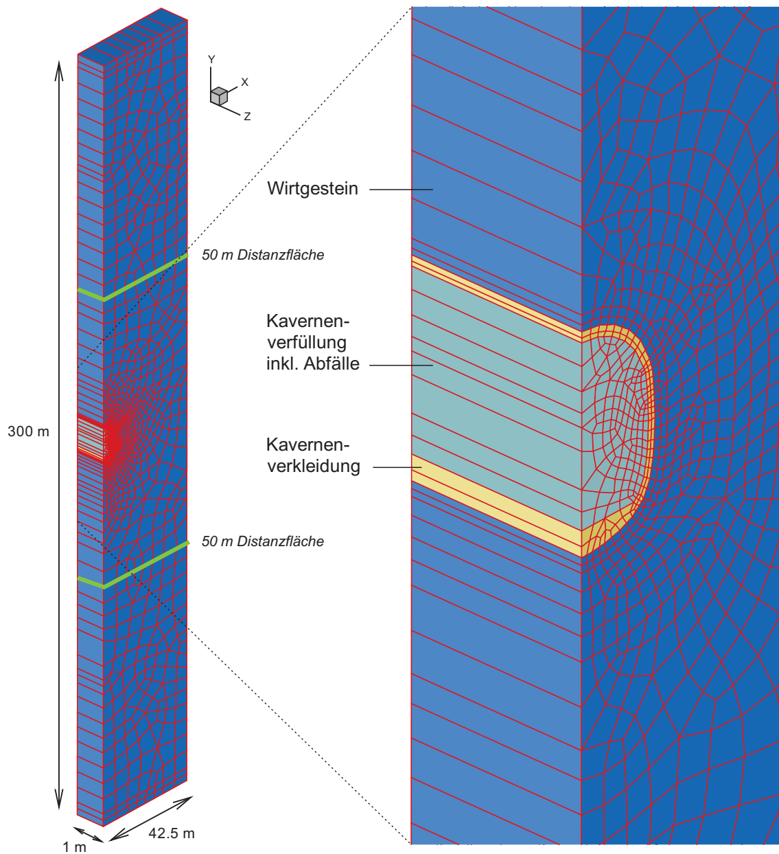
Fig. A4.3-1: Modellgeometrie für VPAC-Rechnungen (homogen-poröses Wirtgestein ohne Klüftung).
