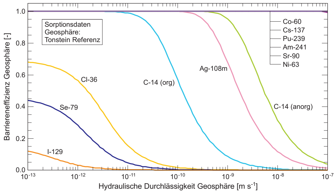
Fig. A5.5-5: Barriereffizienz als Funktion der hydraulischen Durchlässigkeit (homogenporöses WG, i = 0.1 \text{ m/m} , L = 40 \text{ m} , Sorption: Tonstein).
