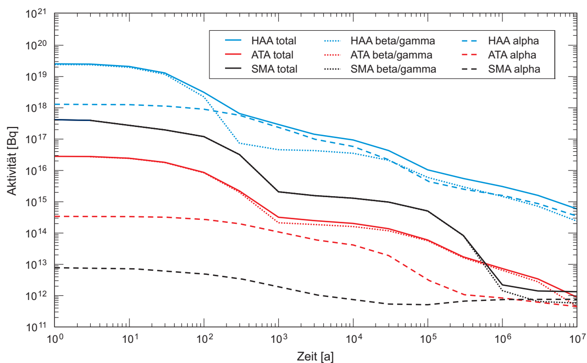
Fig. 3.2-1a: Zeitliche Entwicklung der Aktivität der Abfallkategorien gemäss Definition KEV.
