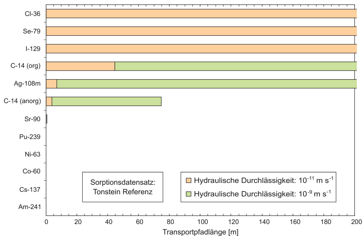
Fig. A5.5-17: Nuklidspezifische Reichweite (99 % Zerfall) im homogen-porösen Wirtgestein (Sorptions: Tonstein).
