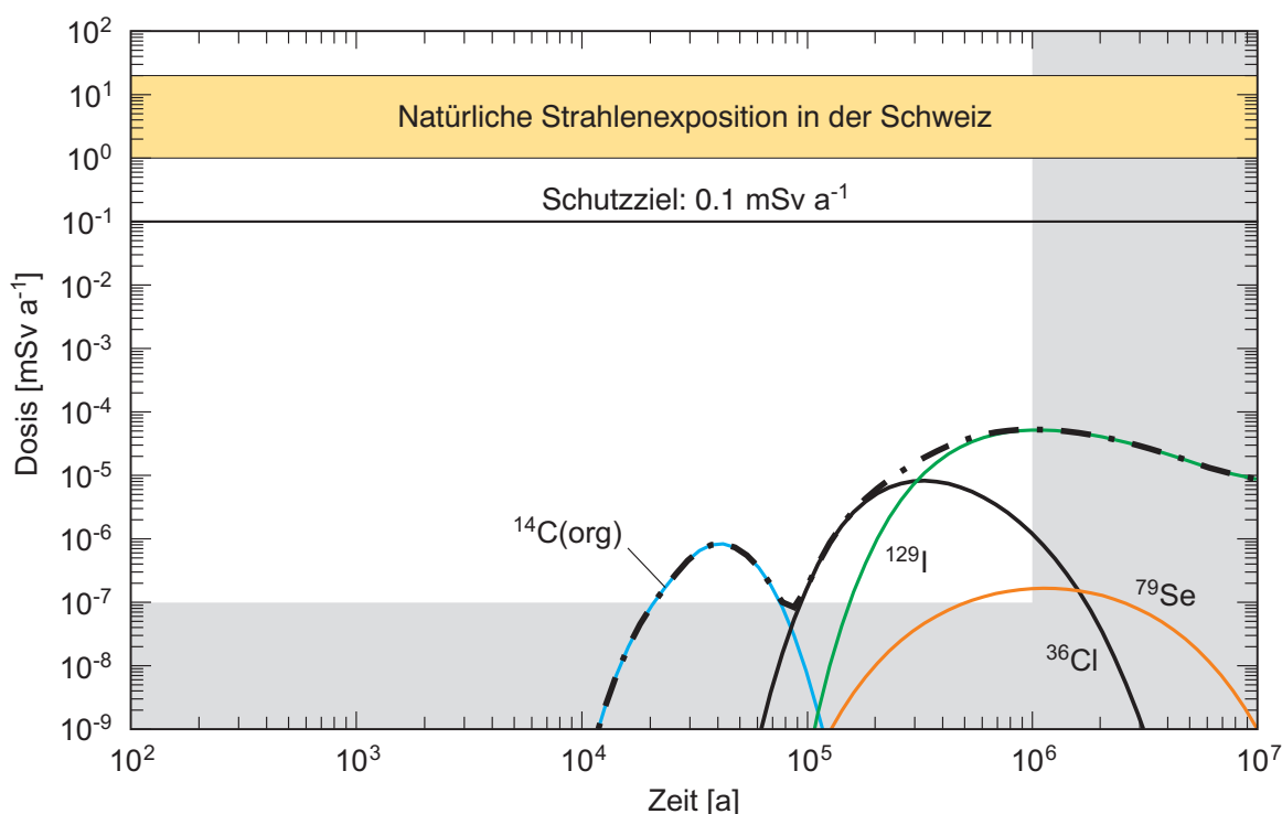
Fig. 2.4-3: Zeitlicher Verlauf der im Projekt Entsorgungsnachweis für ein HAA-Lager berechneten Gesamtdosis für den Referenzfall.
