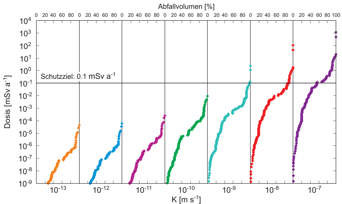
Fig. 3.3-1a: Resultate der Rechenfall-Familie R1: Homogen-poröses Wirtgestein ohne Störungszonen, ausgewertet mit dem Geosphären-Sorptionsdatensatz "Tonstein".
