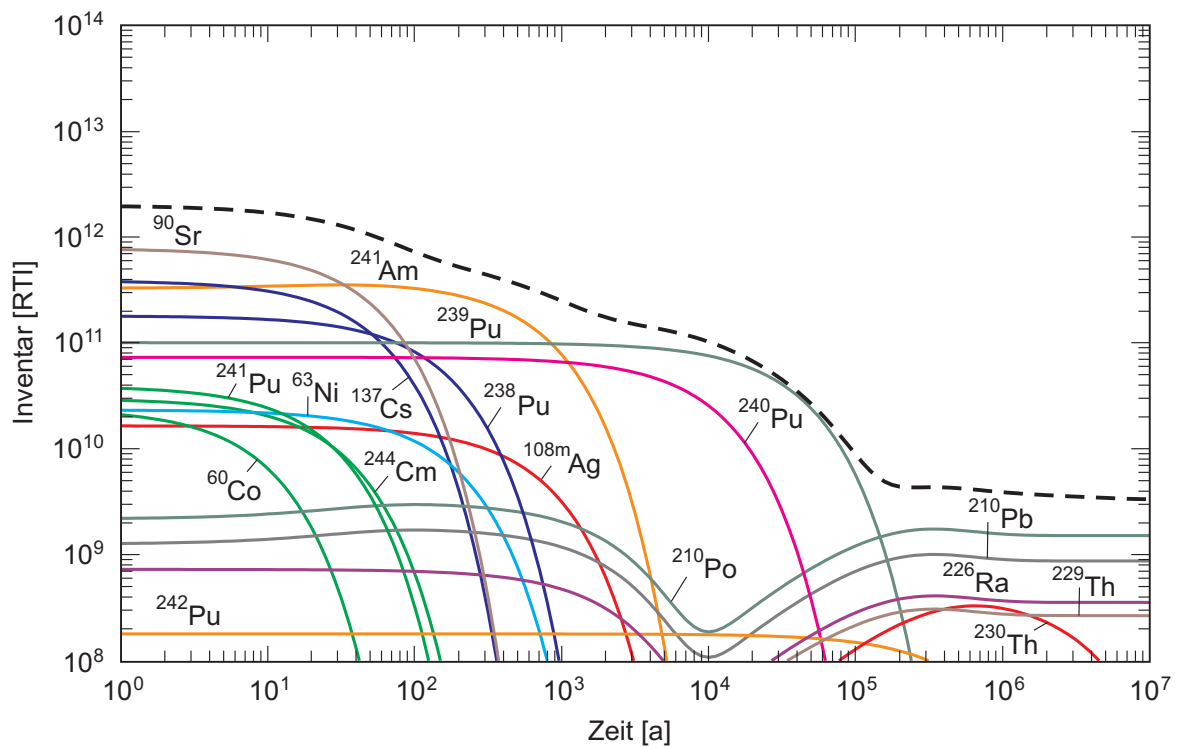
Fig. A5.5-3: Radiotoxizität als Funktion der Zeit für LMA (Referenzzuteilung).
