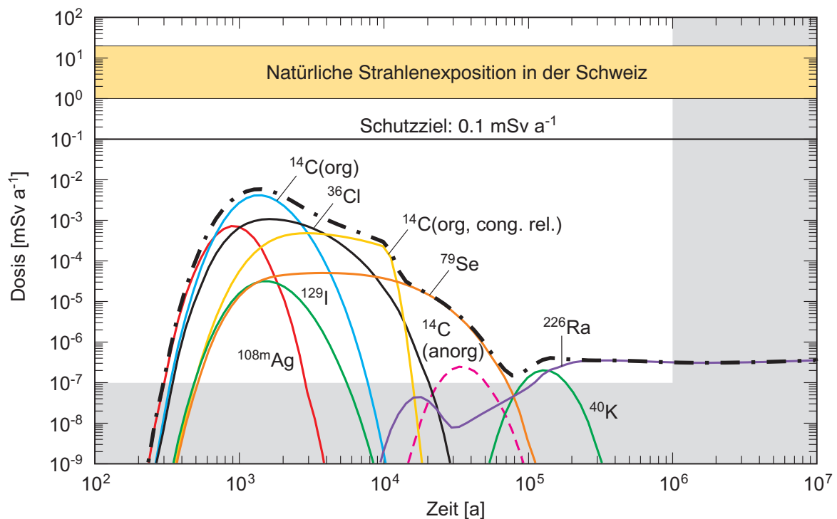
Fig. 3.3-7: Berechnete Dosen für ein SMA-Lager in einem homogen-porösen Wirtgestein (AZ).
