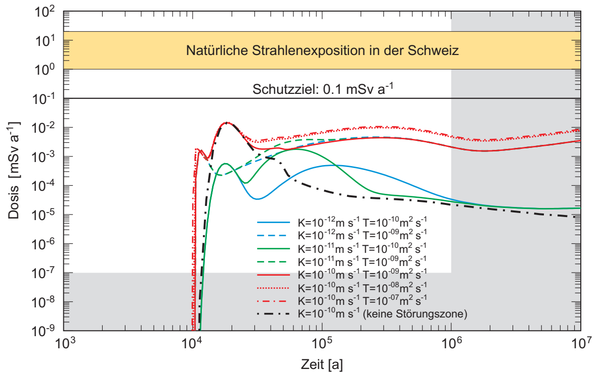
Fig. A5.2-3: Einfluss der Transmissivität einer Störungszone senkrecht zur Achse der Lagerstollen auf die berechnete Dosis für das HAA-Lager.
