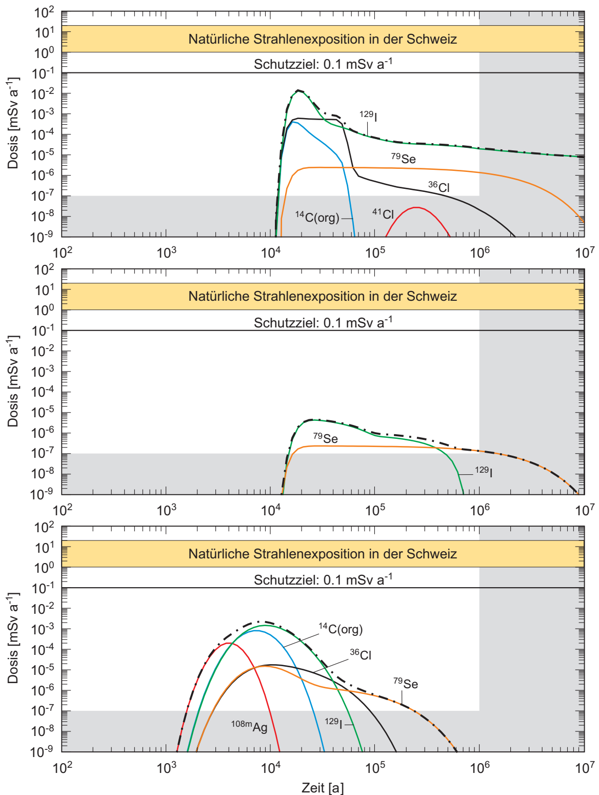
Fig. 4.7-4b: Berechnete Dosen für ein HAA-Lager in einem homogen-porösen Wirtsgestein für K = 10^{-10} \text{ m/s} .
