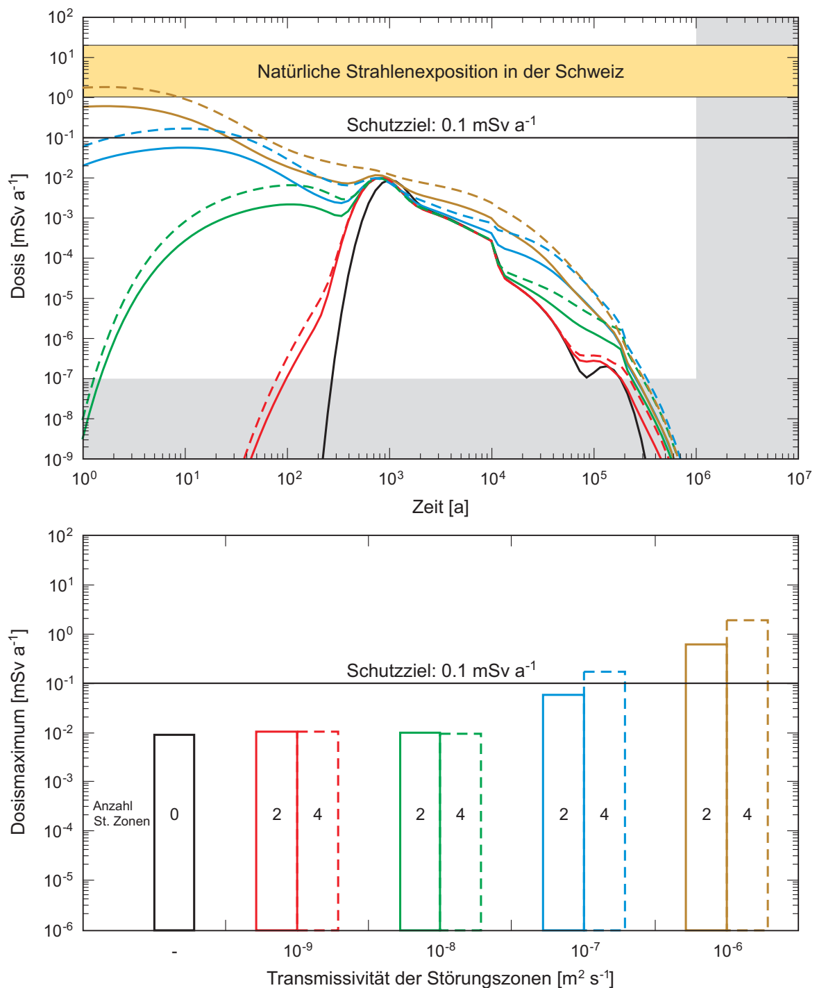
Fig. A5.2-5: Einfluss der Anzahl und Transmissivität von Störungszonen senkrecht zur Achse der Lagerkavernen auf die berechneten Dosismaxima für das SMA-Lager in einem homogen-porösen Wirtgestein.
