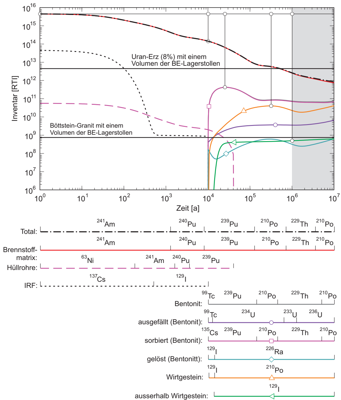
Fig. 4.7-1b: Entwicklung und Aufteilung der Radiotoxizität für abgebrannte Brennelemente auf die verschiedenen Komponenten des Nahfelds, das Wirtgestein und das Gebiet ausserhalb des Wirtgesteins für K = 10^{-10} m/s.
