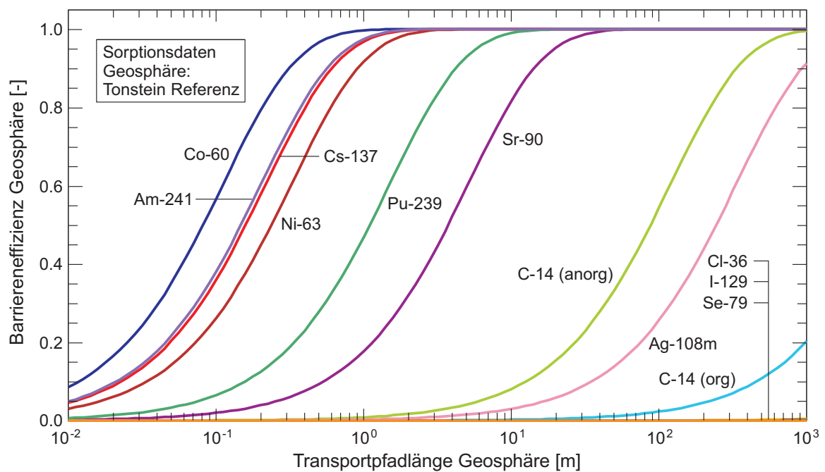
Fig. A5.5-14: Barriereneffizienz als Funktion der Transportpfadlänge (geklüftetes Wirtgestein, i = 0.1 m/m, T = 10^{-8} m 2 /s, Sorption: Tonstein).
