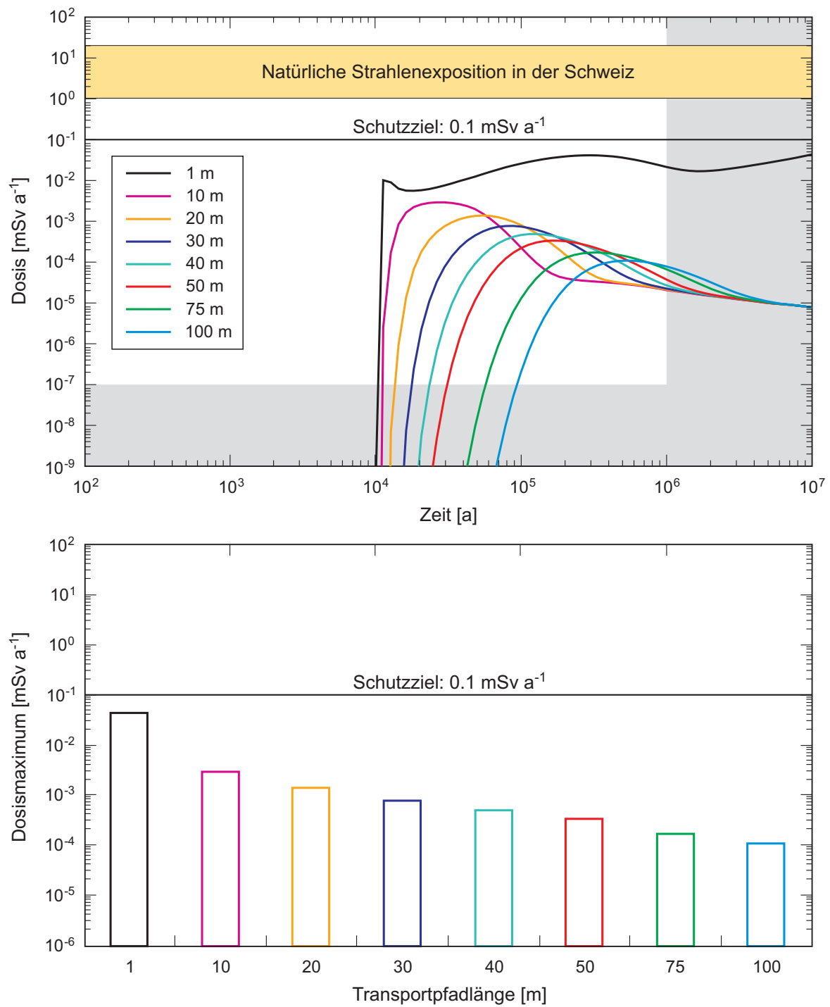
Fig. A5.3-1: Einfluss der Transportpfadlänge auf die berechneten Dosismaxima für ein HAA-Lager (BE) in einem homogen-porösen Wirtgestein für K = 10^{-13} \text{ m/s} .
