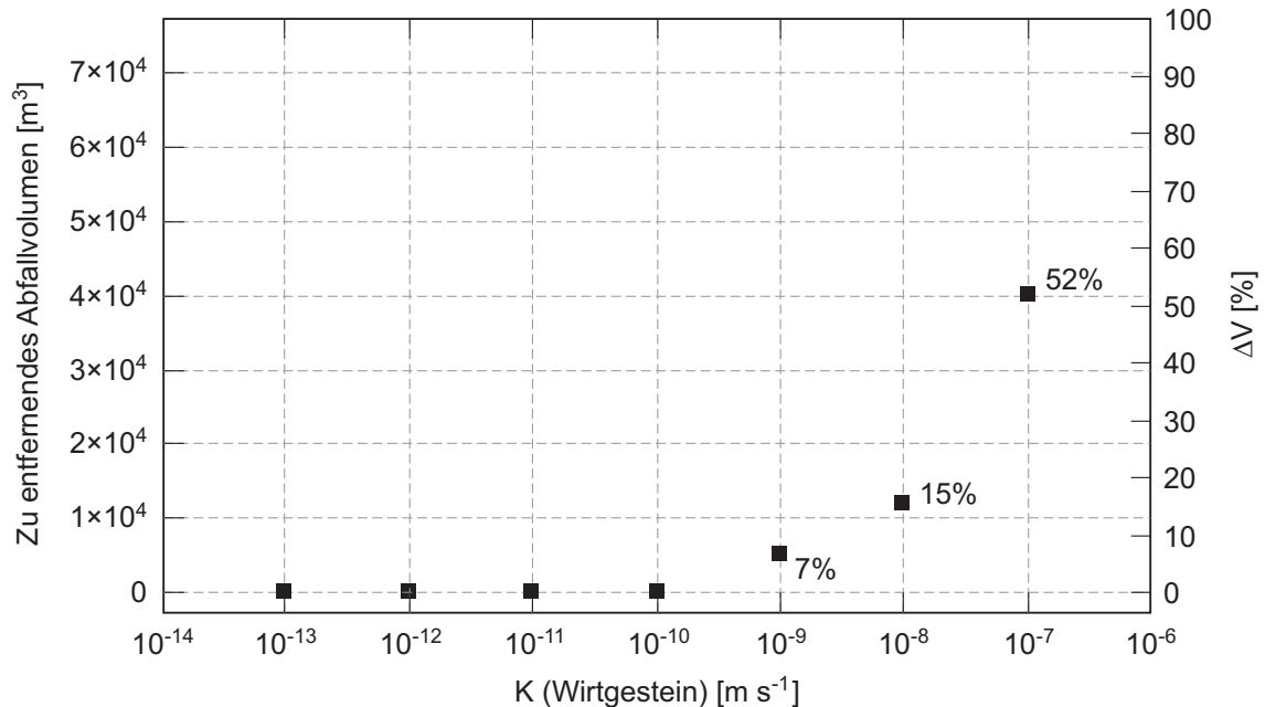
Fig. 3.3-2: Aus dem SMA-Lager zu entfernendes Abfallvolumen als Funktion der hydraulischen Durchlässigkeit eines homogen-porösen Wirtgesteins, damit die gewählte Dosislimite gerade noch unterschritten wird.
