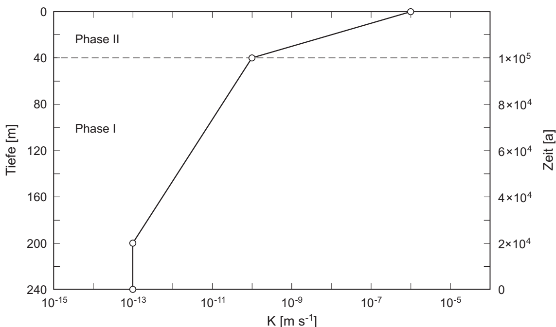
Fig. 2.5-10: Schematische Darstellung der hydraulischen Durchlässigkeit des Opalinustons als Funktion der Tiefe bzw. der Zeit für ein SMA-Lager.
