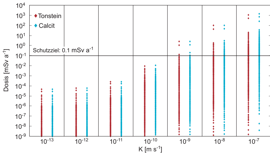
Fig. 3.3-1b: Resultate der Rechenfall-Familie R1: Homogen-poröses Wirtgestein ohne Störungzonen, ausgewertet mit den Geosphären-Sorptionsdatensätzen "Tonstein" und "Calcit".
