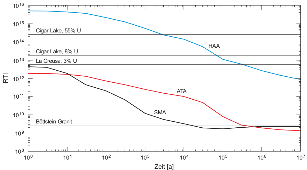
Fig. 3.2-2a: Zeitliche Entwicklung der Radiotoxizität der Abfallkategorien gemäss Definition KEV.
