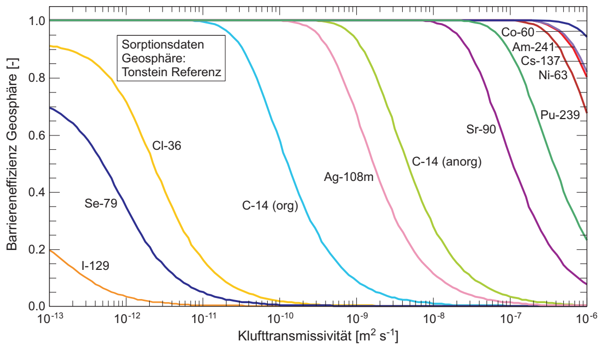
Fig. A5.5-7: Barriereneffizienz als Funktion der Transmissivität (geklüftetes WG, i = 0.1 \text{ m/m} , L = 40 \text{ m} , Sorption: Tonstein).
