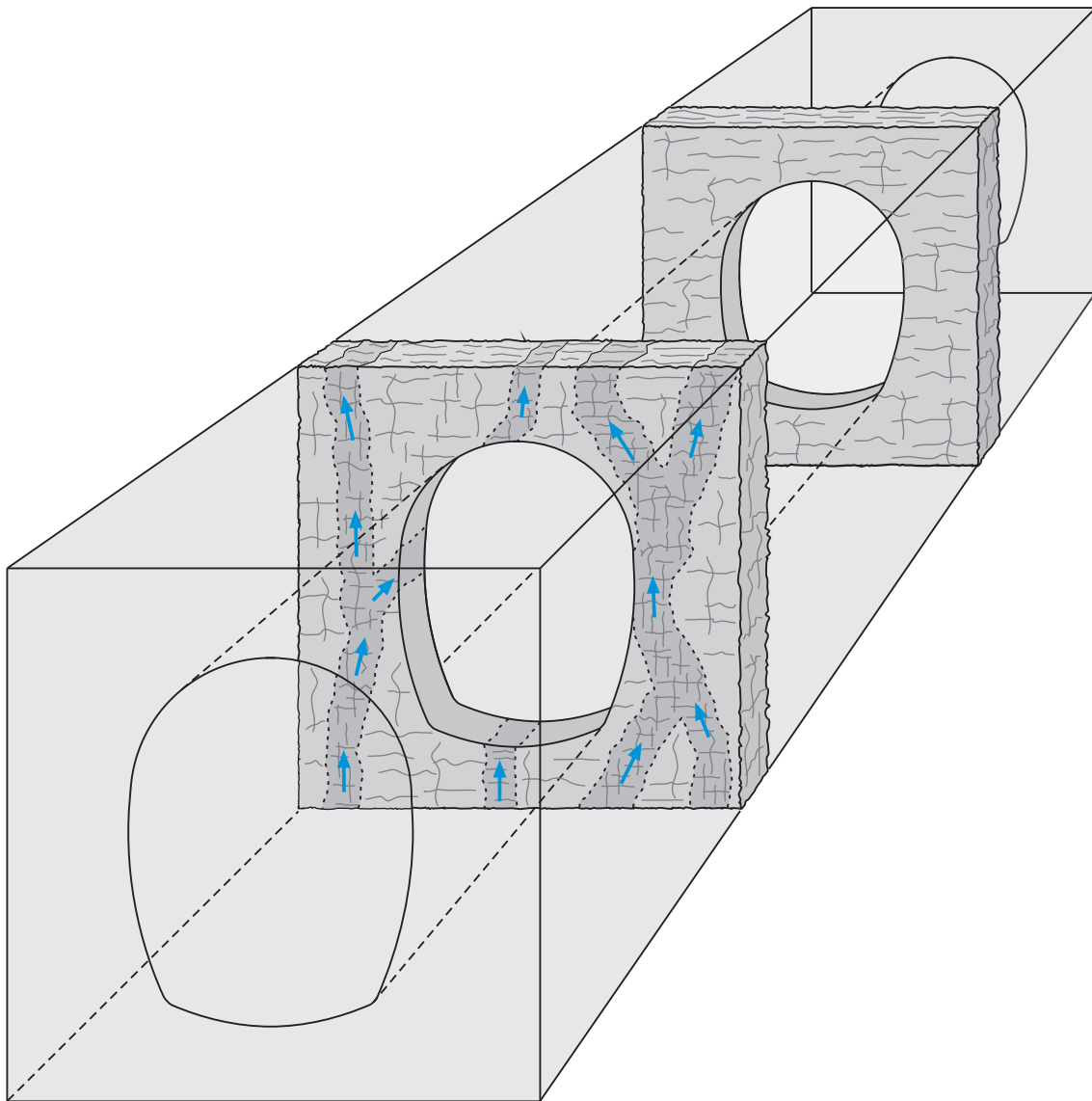
Fig. 2.5-4 Konzeptualisierung von Störungszonen, die eine SMA-Kaverne schneiden.
