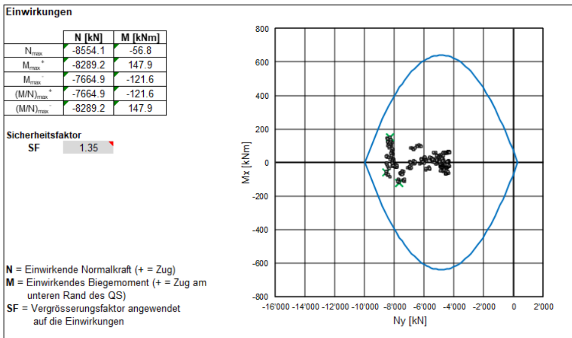
Fig. F-24: Tragsicherheitsnachweis, Schnitt A, 40 Jahre, Spritzbetonschale (C30/37): 50 cm
