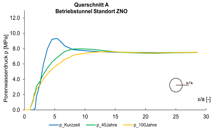
Fig. I-2: Porenwasserdruck entlang der Abfragelinie Parament
