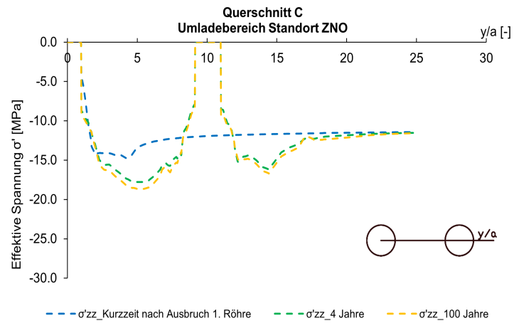
Fig. I-32: Spannung ( \sigma'_{zz} ) entlang der Abfragelinie Parament
