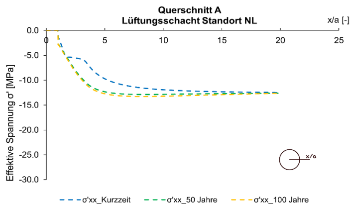
Fig. M-20: Spannung ( \sigma'_{xx} ) entlang der Abfragelinie
