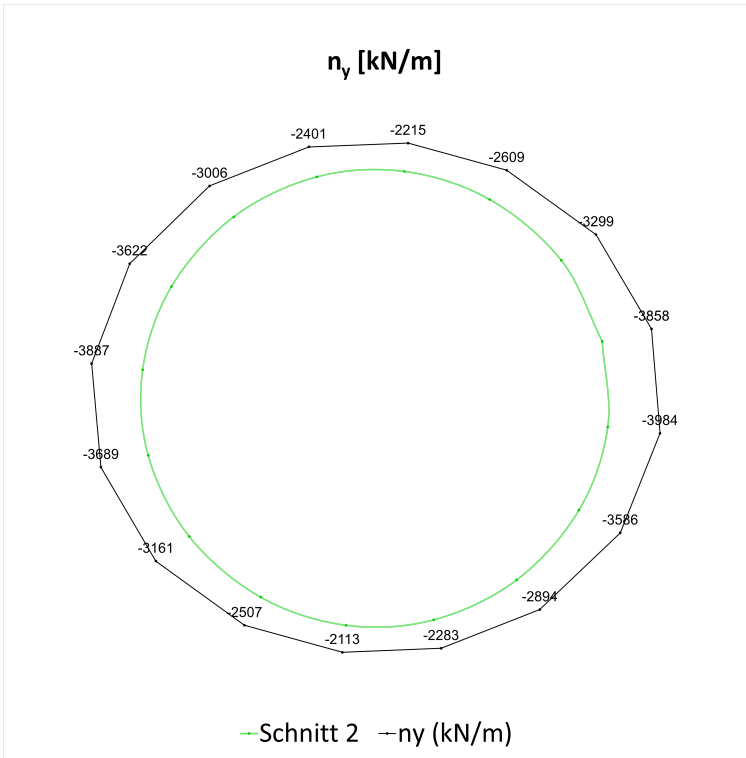
Fig. C-66 Normalkraft ( N_y ) in Umfangsrichtung, Schnitt 2, 100 Jahre
