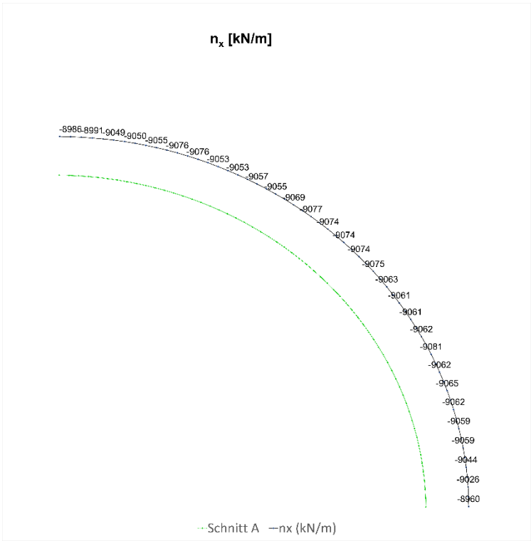
Fig. N-32: Normalkraft ( N_x ) in Umfangsrichtung, Schnitt A, 100 Jahre
