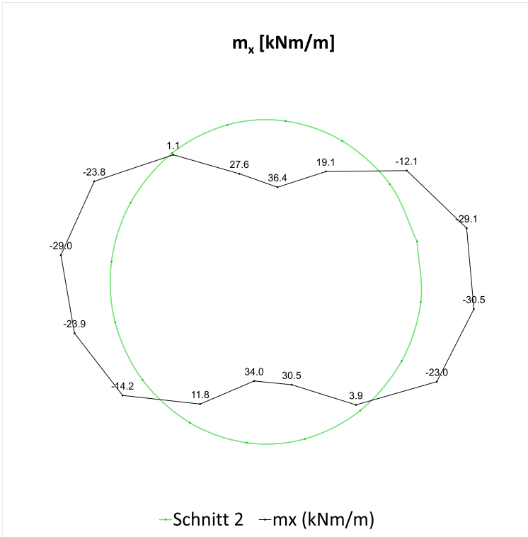
Fig. C-67 Biegemoment ( M_x ), Schnitt 2, 100 Jahre
