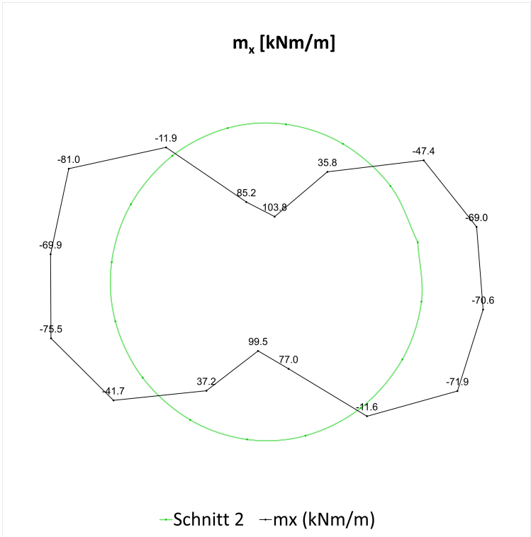
Fig. F-67: Biegemoment ( M_x ), Schnitt 2, 100 Jahre
