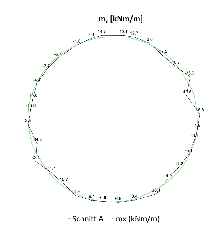
Fig. C-22 Biegemoment ( M_x ), Schnitt A, 100 Jahre
