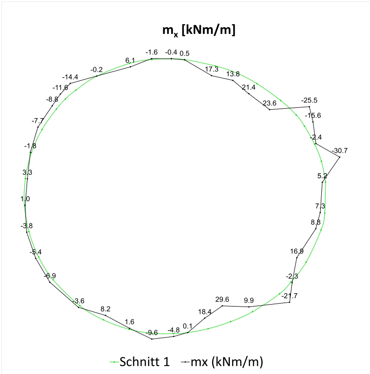
Fig. C-41 Biegemoment ( M_x ), Schnitt 1, 40 Jahre
