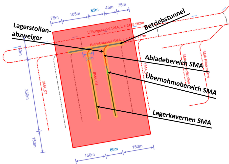
Fig. 2-5: Abgrenzung des Berechnungsmodells SMA
