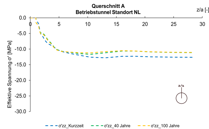
Fig. F-9: Spannung ( \sigma'_{zz} ) entlang der Abfragelinie Firste
