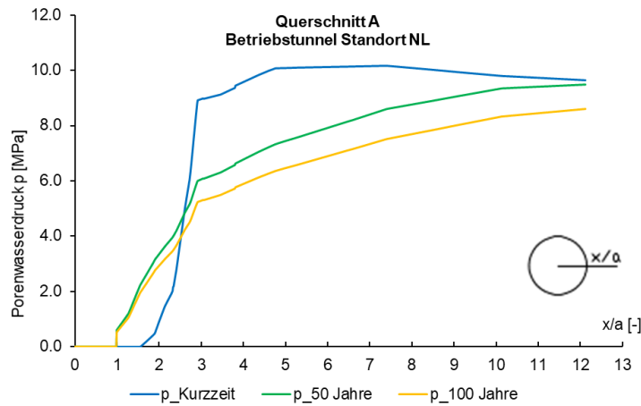
Fig. G-2: Porenwasserdruck entlang der Abfragelinie Parament
