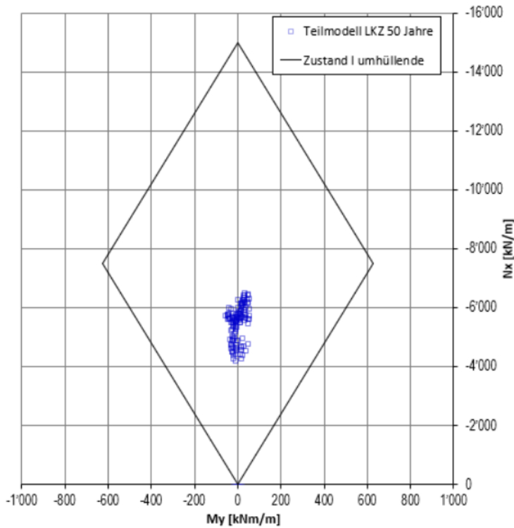
Fig. K-14: Gebrauchstauglichkeitsnachweis, Schnitt 3, 50 Jahre, Spritzbetonschale (C30/37): 50 cm
