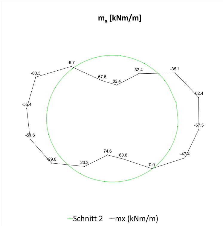
Fig. I-67: Biegemoment ( M_x ), Schnitt 2, 100 Jahre
