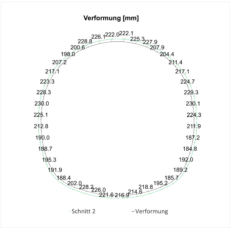
Fig. G-54: Verformung des Querschnitts 2, Kurzzeit
