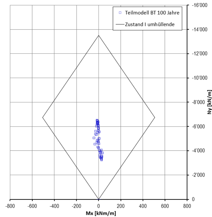
Fig. K-10: Gebrauchstauglichkeitsnachweis, Schnitt A, 100 Jahre, Spritzbetonschale (C30/37): 45 cm
