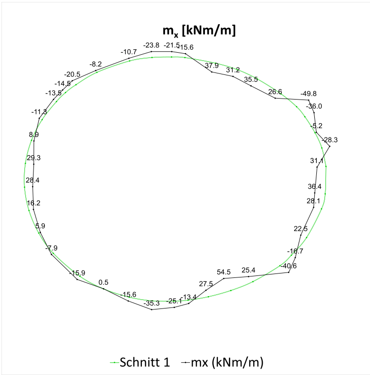
Fig. I-41: Biegemoment ( M_x ), Schnitt 1, 40 Jahre
