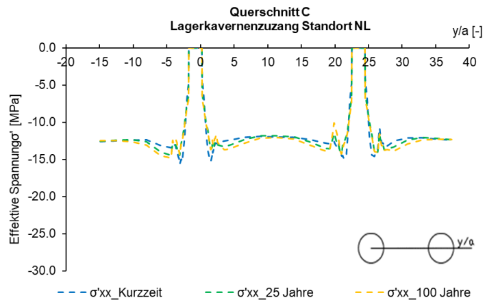
Fig. G-30: Spannung ( \sigma'_{xx} ) entlang der Abfragelinie Parament
