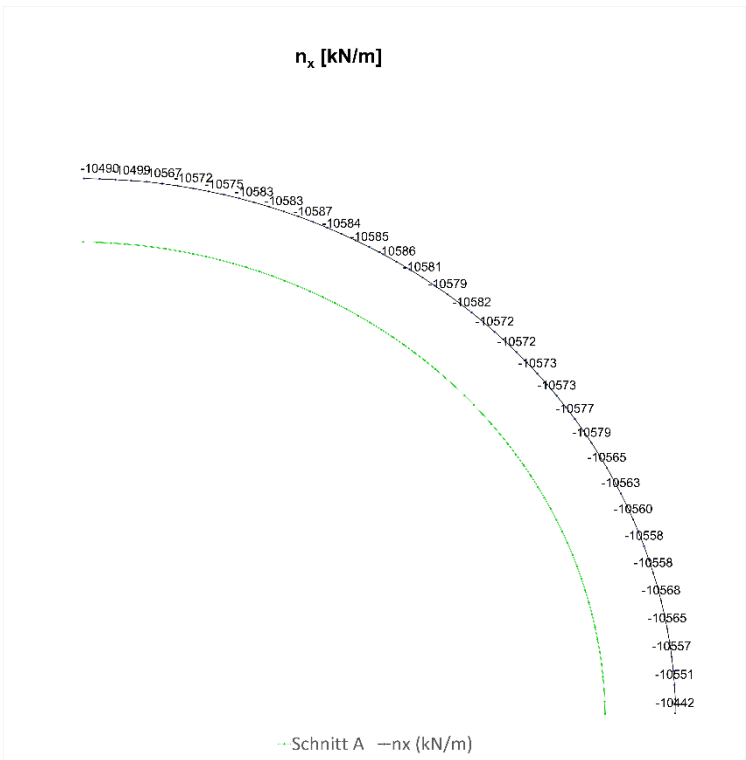
Fig. M-32: Normalkraft ( N_x ) in Umfangsrichtung, Schnitt A, 100 Jahre
