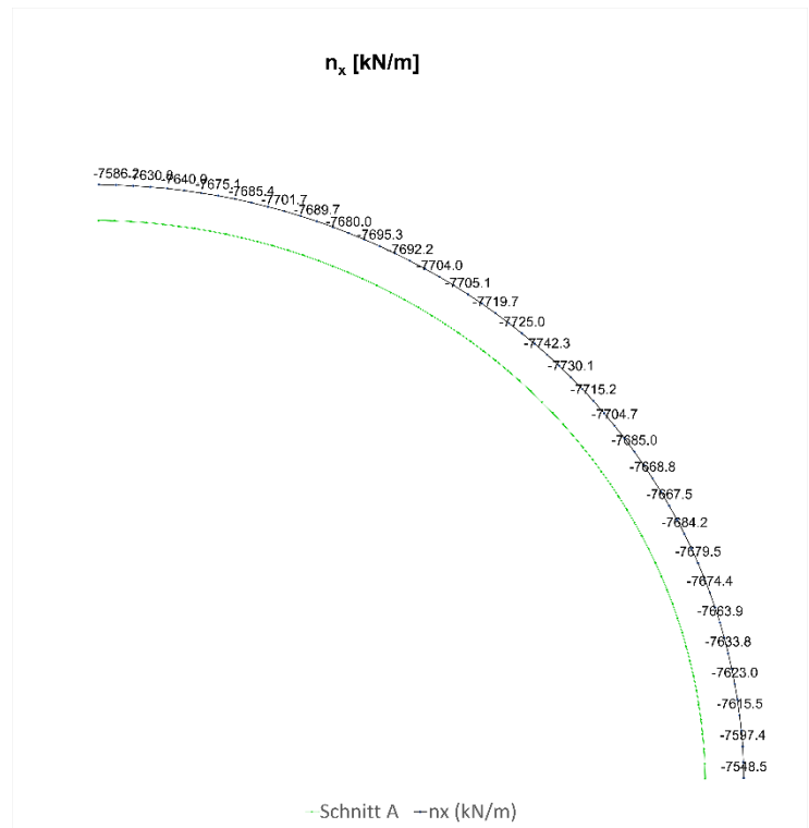
Fig. N-8: Normalkraft ( N_x ) in Umfangsrichtung, Schnitt A, Kurzzeit
