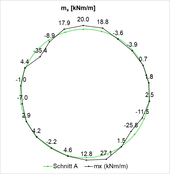
Fig. J-19: Biegemoment ( M_x ), Schnitt A, 50 Jahre
