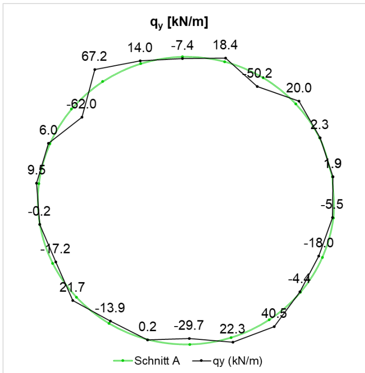
Fig. J-20: Querkraft ( Q_y ), Schnitt A, 50 Jahre
