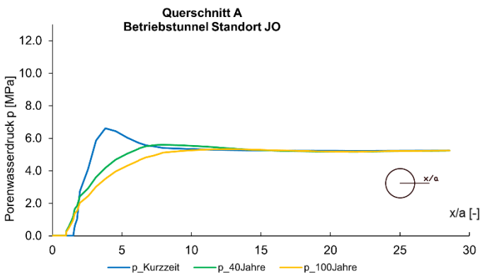
Fig. C-2 Porenwasserdruck entlang der Abfragelinie Parament
