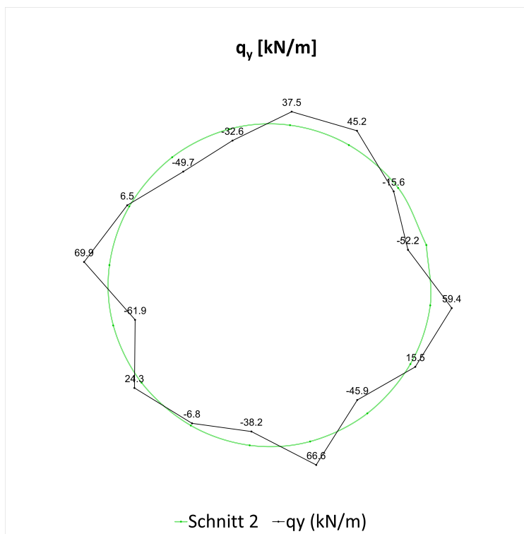
Fig. F-65: Querkraft ( Q_y ), Schnitt 2, 4 Jahre
