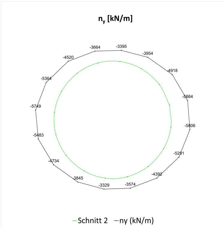
Fig. I-66: Normalkraft ( N_y ) in Umfangsrichtung, Schnitt 2, 100 Jahre
