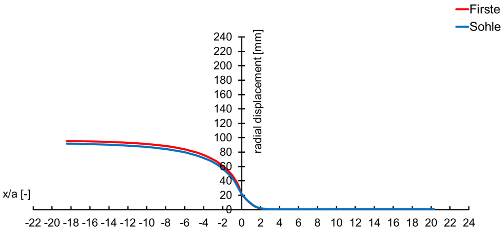
Fig. D-53: Radialverschiebung vs. Ortsbrustposition, Schnitt 2, Kurzzeit
