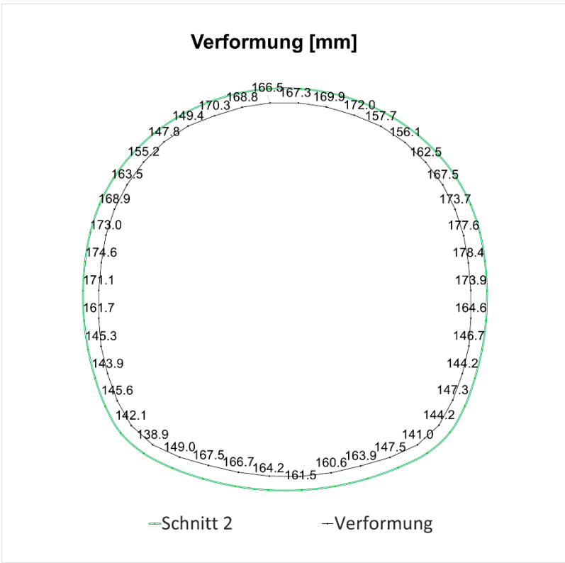
Fig. J-54: Verformung des Querschnitts 2, Kurzzeit
