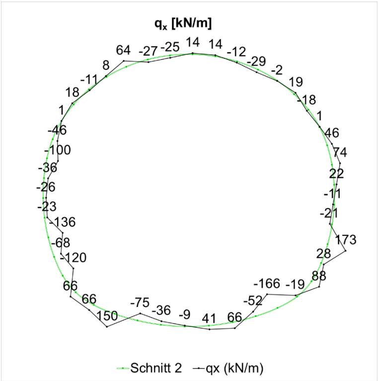
Fig. J-66: Querkraft ( Q_x ), Schnitt 2, 100 Jahre
