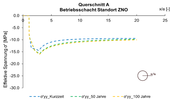
Fig. N-3: Spannung ( \sigma'_{yy} ) entlang der Abfragelinie
