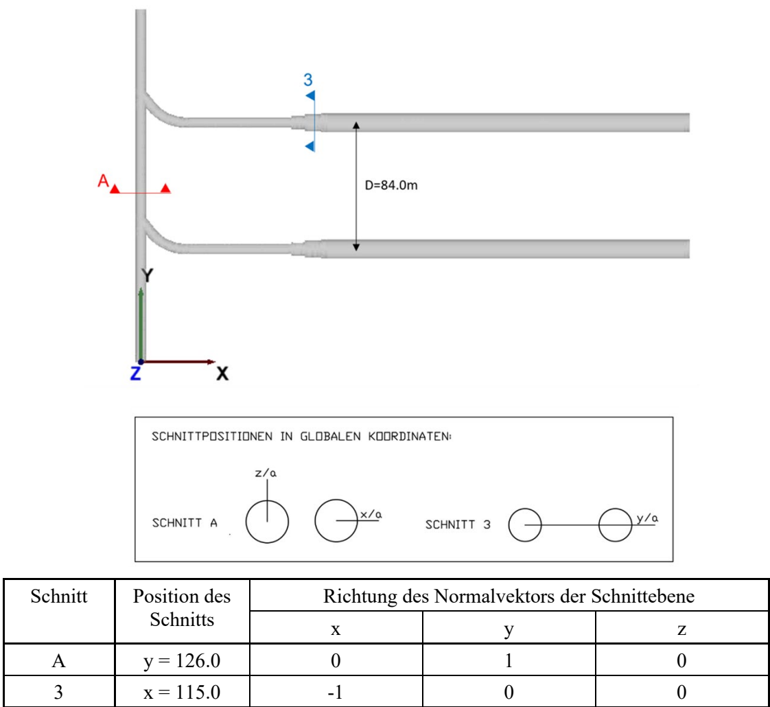
Fig. H-2: Definition der Schnittebenen SMA
