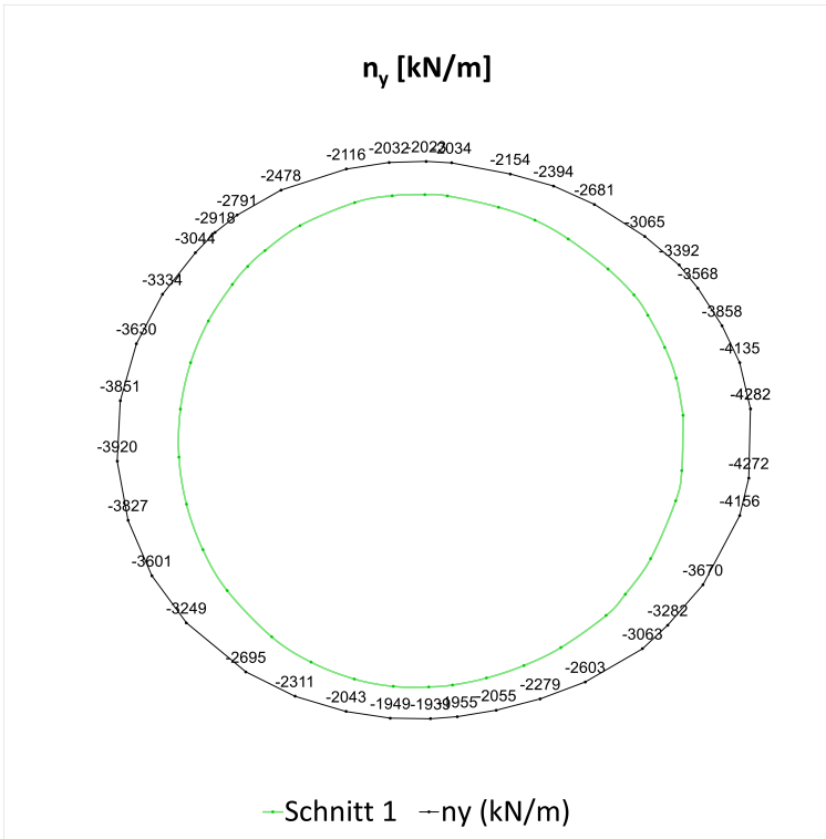
Fig. C-40 Normalkraft ( N_y ) in Umfangsrichtung, Schnitt 1, 40 Jahre
