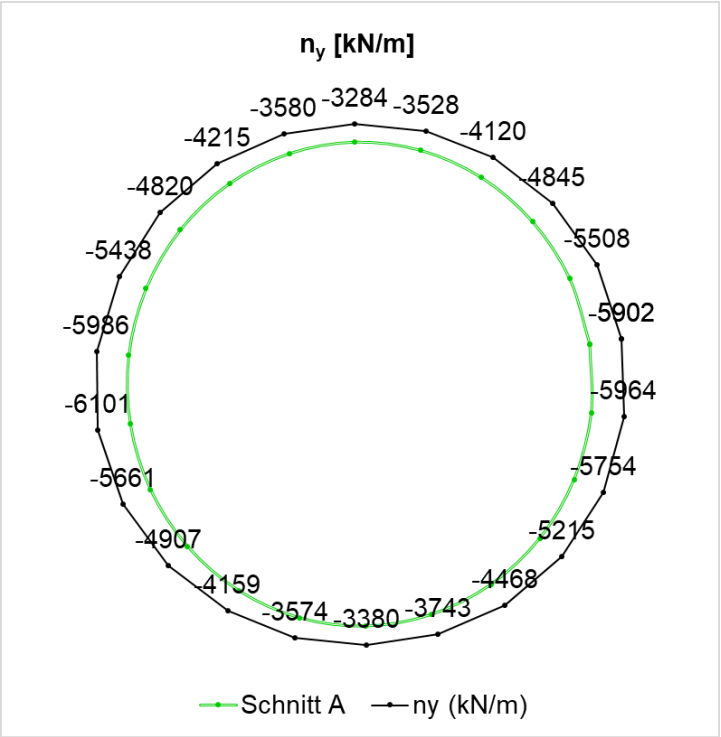
Fig. J-18: Normalkraft ( N_y ) in Umfangsrichtung, Schnitt A, 50 Jahre
