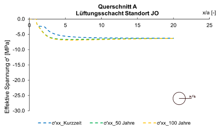
Fig. L-2: Spannung ( \sigma'_{xx} ) entlang der Abfragelinie
