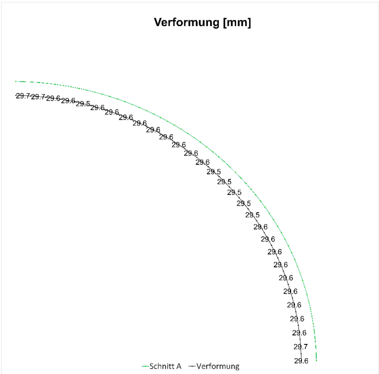
Fig. N-6: Verformungen am Schnitt A, 50 Jahre
