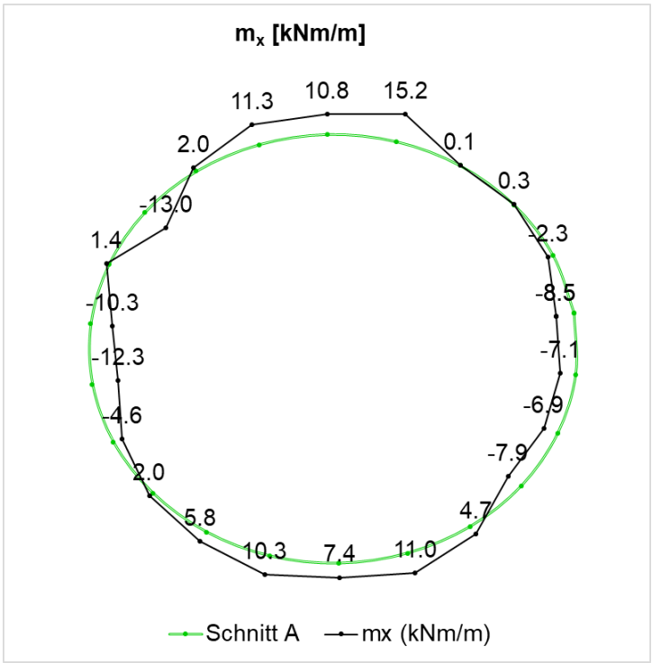
Fig. D-19: Biegemoment ( M_x ), Schnitt A, 50 Jahre
