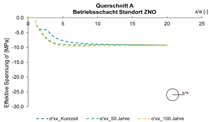
Fig. N-2: Spannung ( \sigma'_{xx} ) entlang der Abfragelinie
