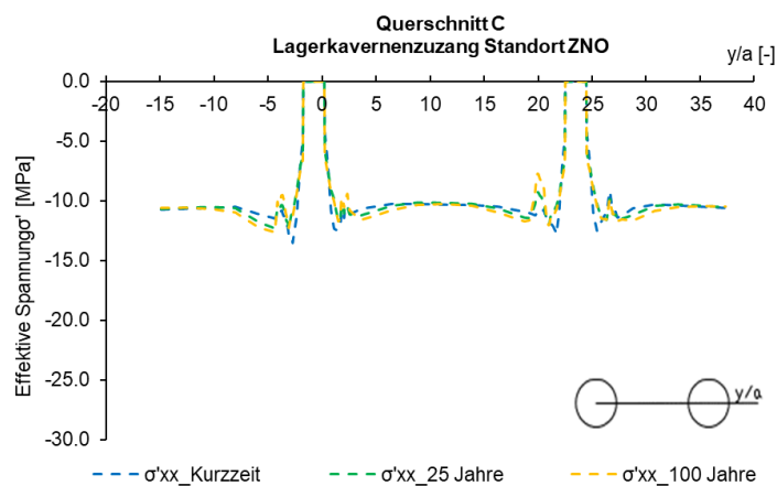
Fig. J-30: Spannung ( \sigma'_{xx} ) entlang der Abfragelinie Parament
