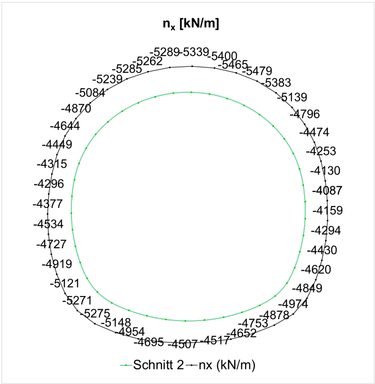
Fig. G-61: Normalkraft ( N_x ) in Umfangsrichtung, Schnitt 2 , 25 Jahre
