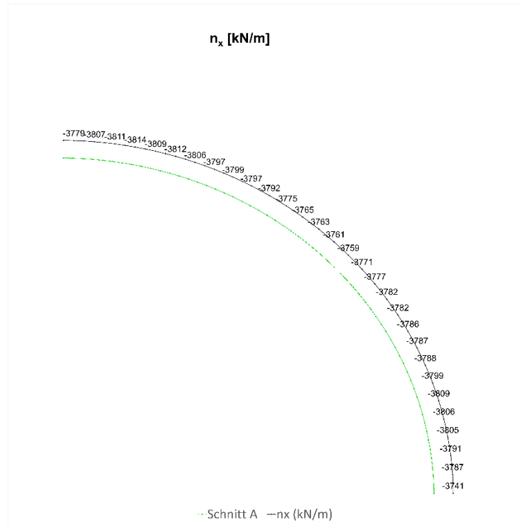
Fig. L-8: Normalkraft ( N_x ) in Umfangsrichtung, Schnitt A, Kurzzeit
