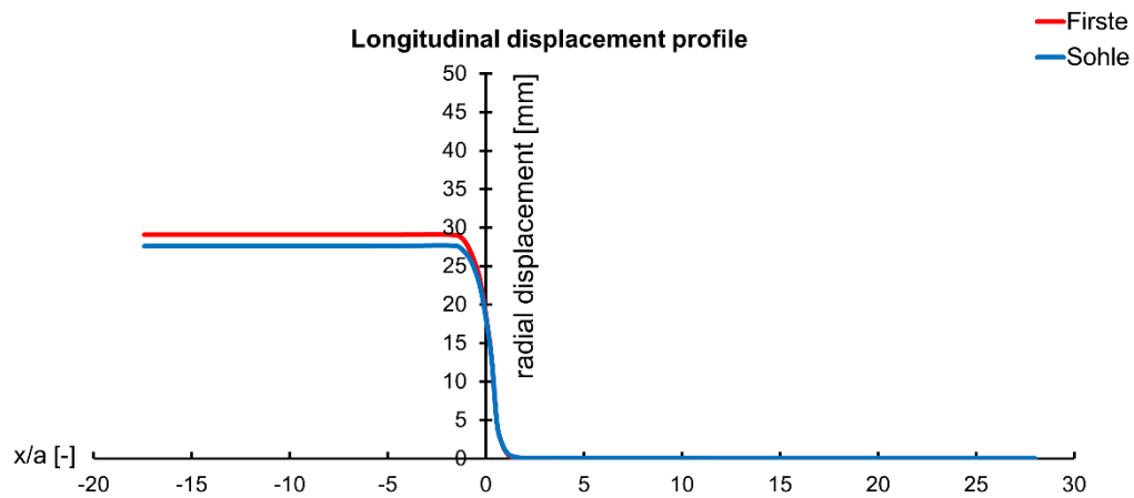
Fig. I-52: Radialverschiebung vs. Ortsbrustposition, Lagerstollen, Schnitt 2
