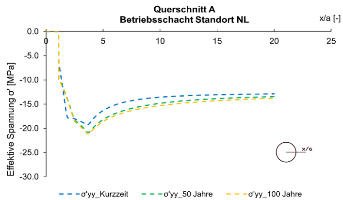
Fig. M-3: Spannung ( \sigma'_{yy} ) entlang der Abfragelinie
