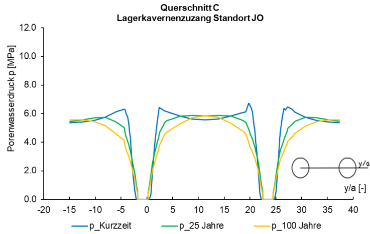
Fig. D-29: Porenwasserdruck entlang der Abfragelinie Parament
