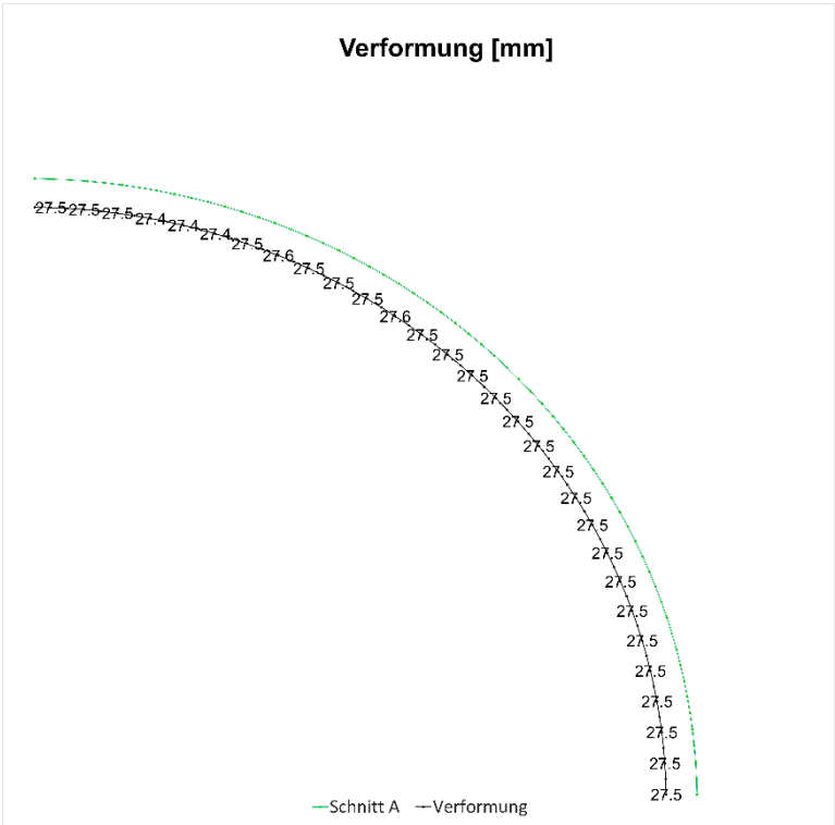
Fig. N-5: Verformungen am Schnitt A, Kurzzeit
