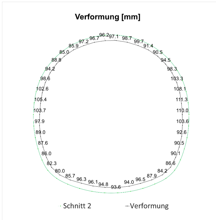
Fig. D-55: Verformung des Querschnitts 2, 25 Jahre
