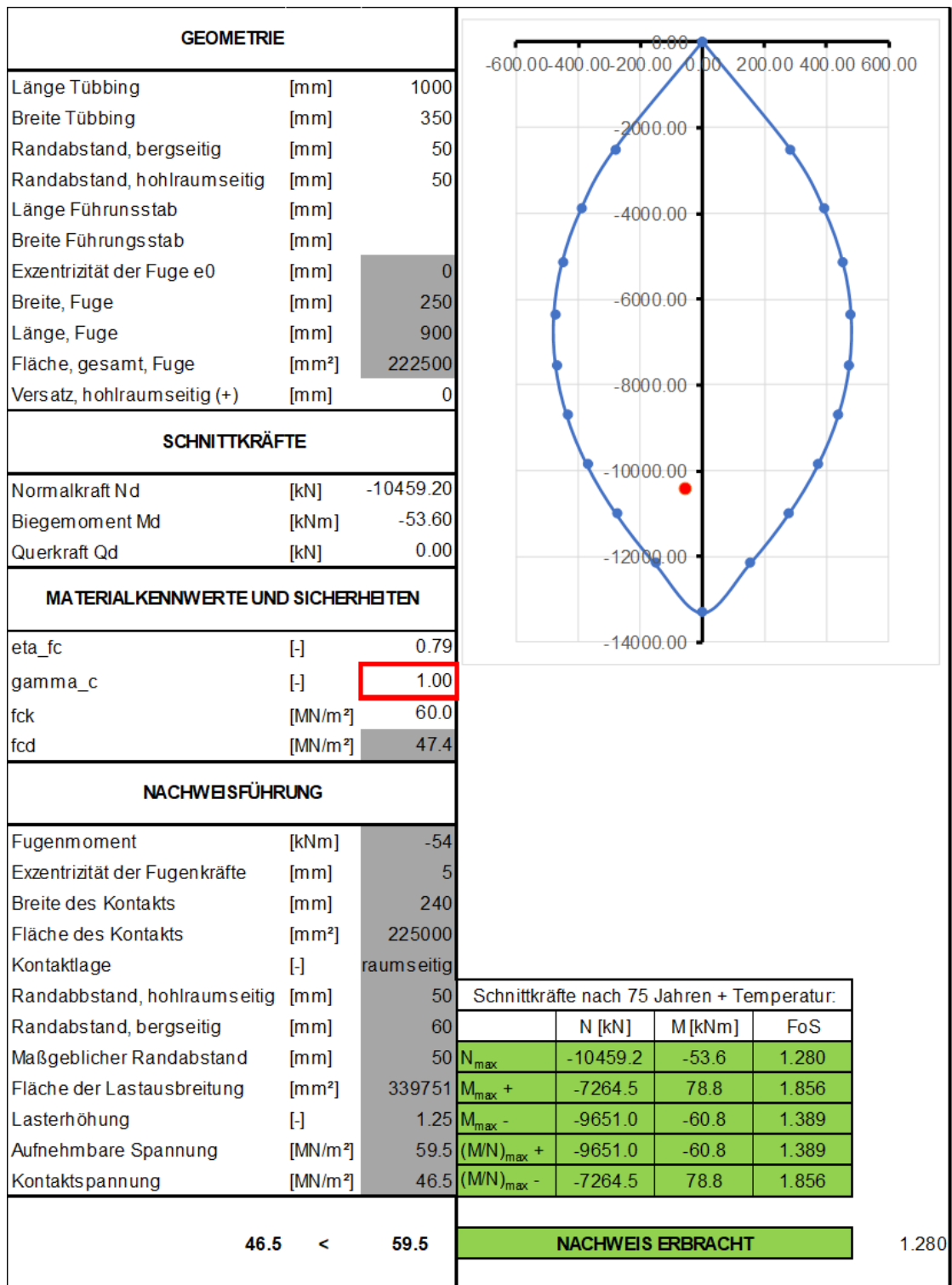
Fig. I-74: Längsfugennachweis, Schnitt 2, 75 Jahre, SF=1, Tübbing (C60/75): 35 cm
