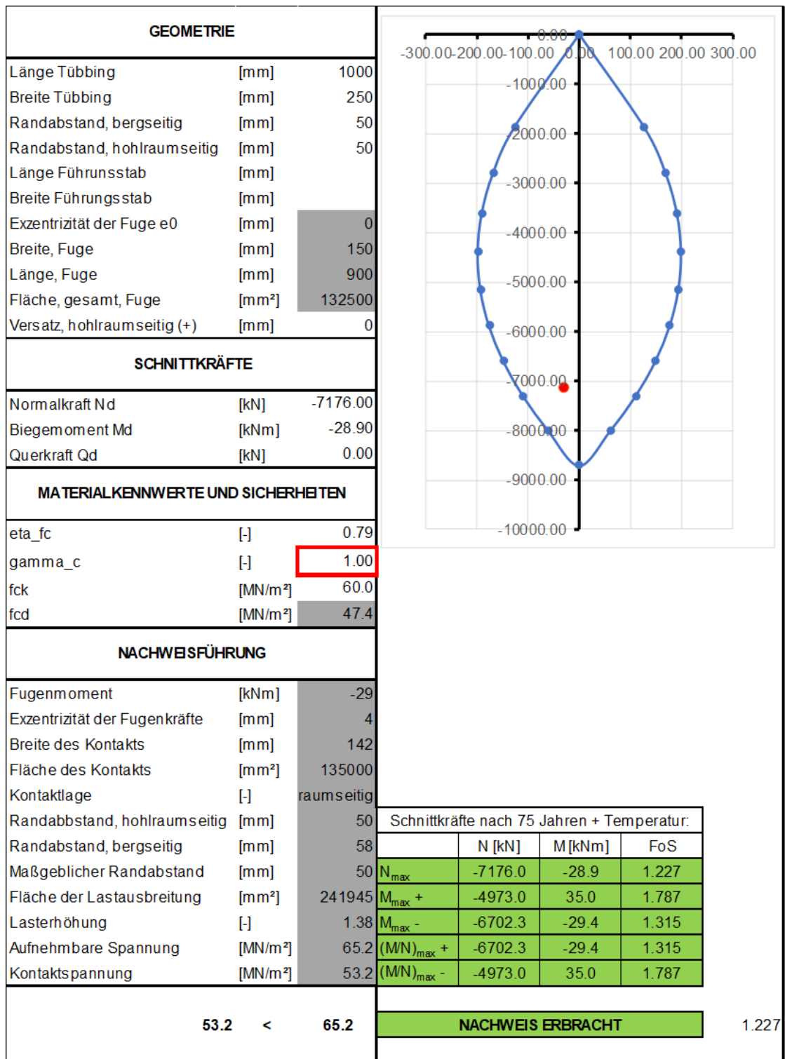
Fig. C-74 Längsfugennachweis, Schnitt 2, 75 Jahre, SF=1, Tübbing (C60/75): 25 cm
