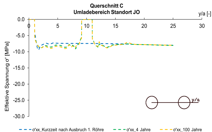
Fig. C-30 Spannung ( \sigma'_{xx} ) entlang der Abfragelinie Parament
