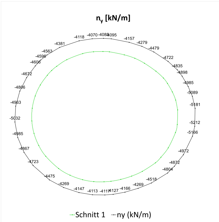
Fig. I-40: Normalkraft ( N_y ) in Umfangsrichtung, Schnitt 1, 40 Jahre
