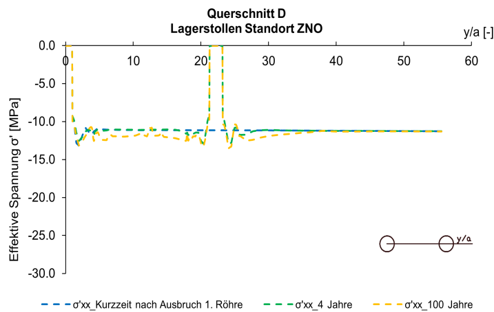
Fig. I-49: Spannung ( \sigma'_{xx} ) entlang der Abfragelinie Parament
