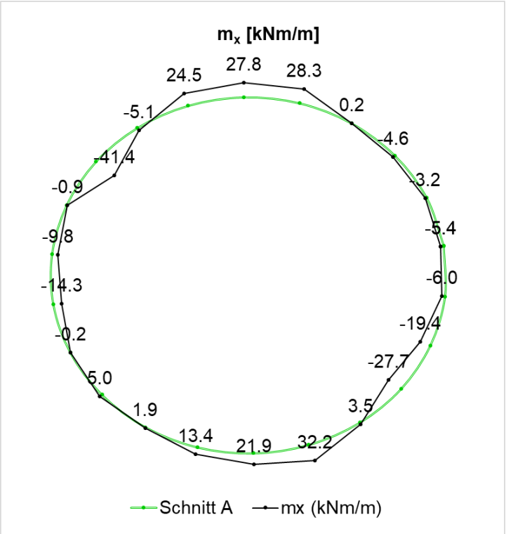
Fig. J-22: Biegemoment ( M_x ), Schnitt A, 100 Jahre
