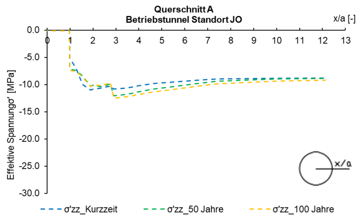
Fig. D-8: Spannung ( \sigma'_{zz} ) entlang der Abfragelinie Parament
