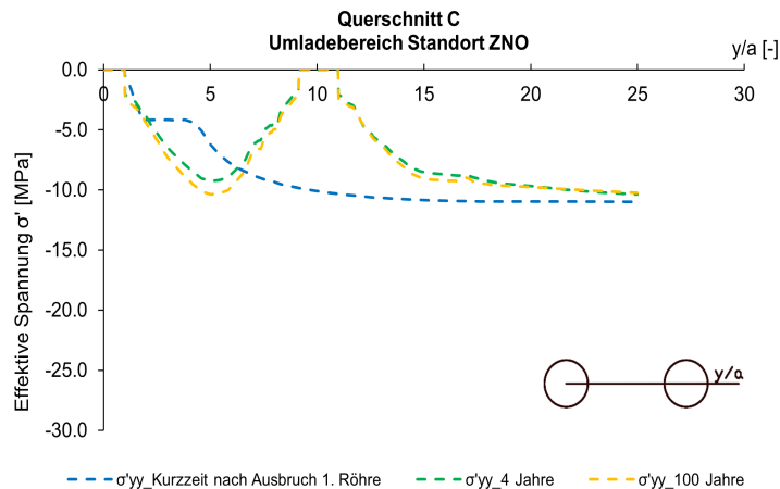
Fig. I-31: Spannung ( \sigma'_{yy} ) entlang der Abfragelinie Parament
