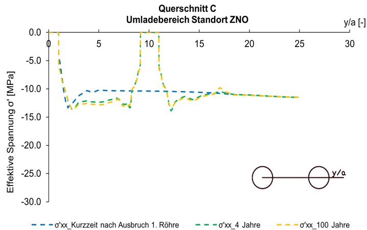
Fig. I-30: Spannung ( \sigma'_{xx} ) entlang der Abfragelinie Parament
