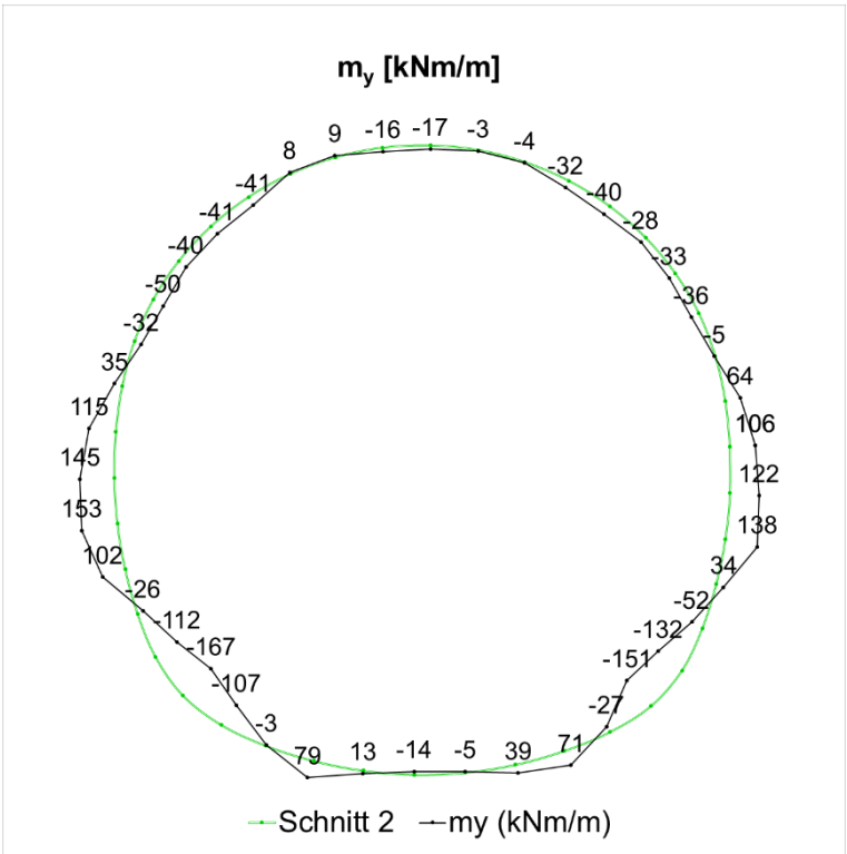
Fig. J-65: Biegemoment ( M_y ), Schnitt 2, 100 Jahre
