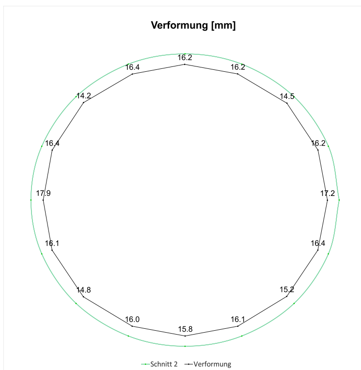
Fig. C-53 Verformungen des Querschnitts, Schnitt 2, Kurzzeit
