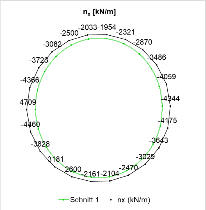
Fig. D-44: Normalkraft ( N_x ) in Umfangsrichtung, Schnitt 1, 100 Jahre
