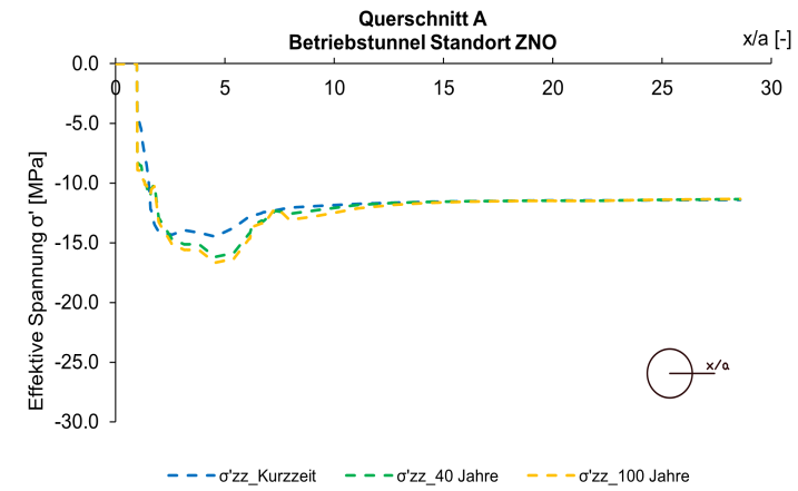
Fig. I-8: Spannung ( \sigma'_{zz} ) entlang der Abfragelinie Parament
