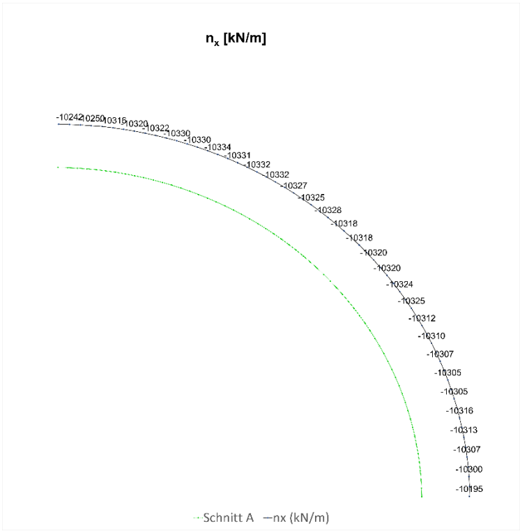
Fig. M-29: Normalkraft ( N_x ) in Umfangsrichtung, Schnitt A, 50 Jahre
