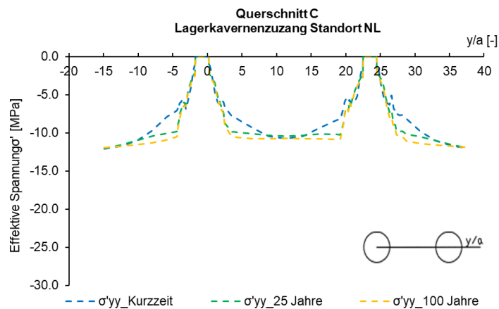
Fig. G-31: Spannung ( \sigma'_{yy} ) entlang der Abfragelinie Parament
