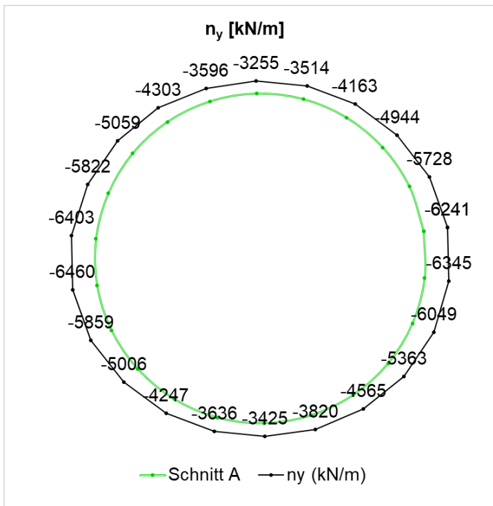
Fig. J-21: Normalkraft ( N_y ) in Umfangsrichtung, Schnitt A, 100 Jahre
