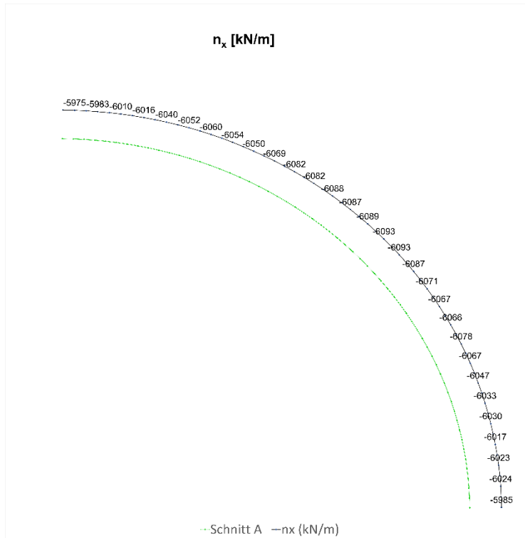
Fig. N-26: Normalkraft ( N_x ) in Umfangsrichtung, Schnitt A, Kurzzeit
