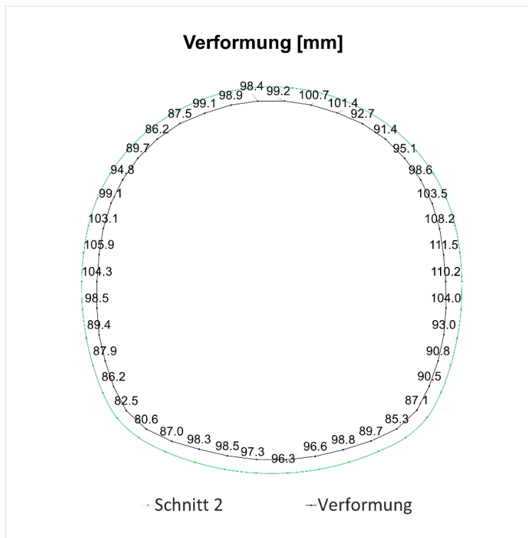
Fig. D-56: Verformung des Querschnitts 2, 100 Jahre
