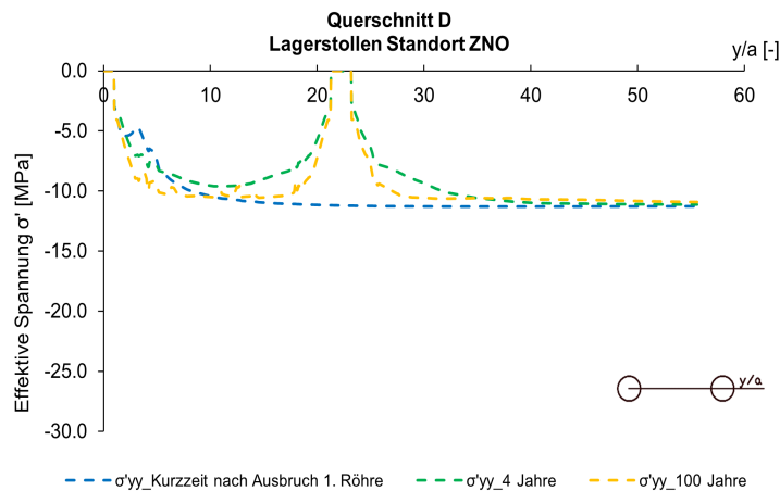
Fig. I-50: Spannung ( \sigma'_{yy} ) entlang der Abfragelinie Parament
