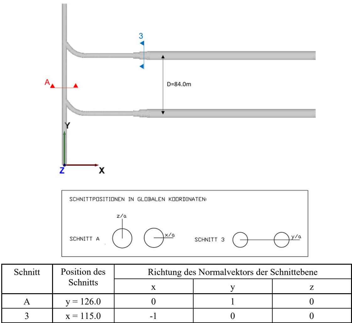
Fig. K-2: Definition der Schnittebenen SMA
