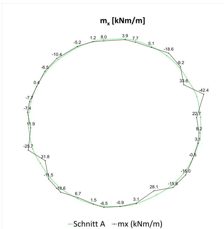
Fig. C-19 Biegemoment ( M_x ), Schnitt A, 40 Jahre
