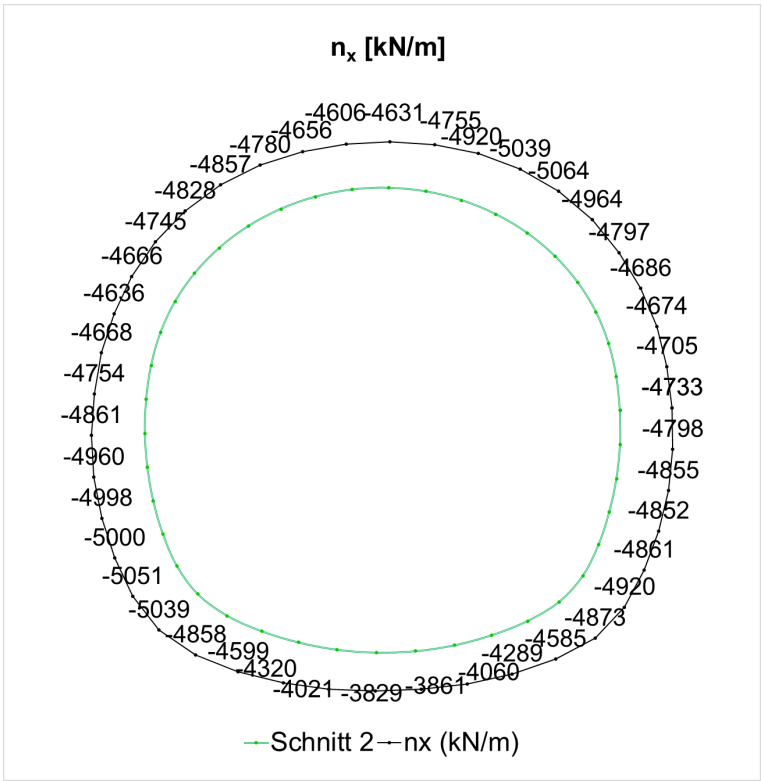
Fig. J-61: Normalkraft ( N_x ) in Umfangsrichtung, Schnitt 2 , 25 Jahre
