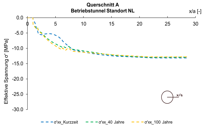
Fig. F-4: Spannung ( \sigma'_{xx} ) entlang der Abfragelinie Parament
