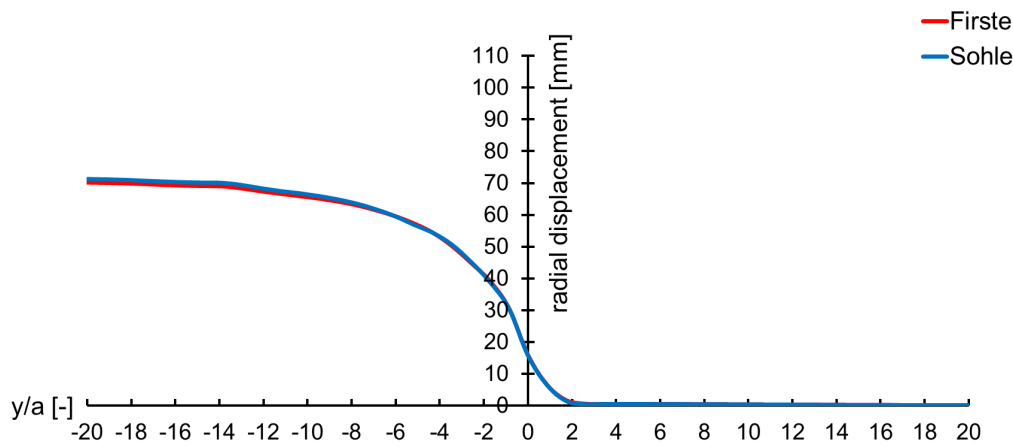
Fig. J-10: Radialverschiebung vs. Ortsbrustposition, Schnitt A, Kurzzeit
