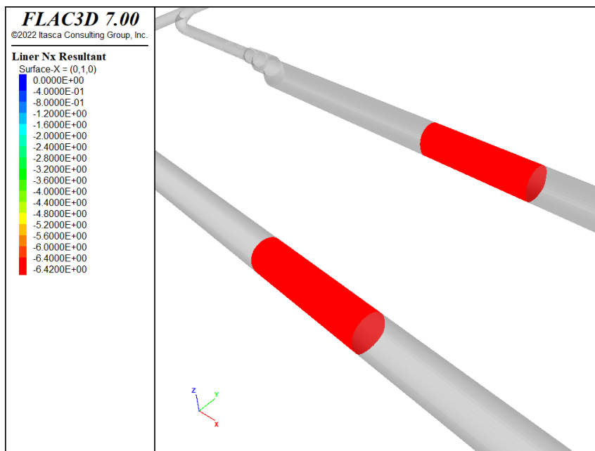
Fig. J-60: Normalkraft N_x (MN/m) in Umfangsrichtung, 100 Jahre
