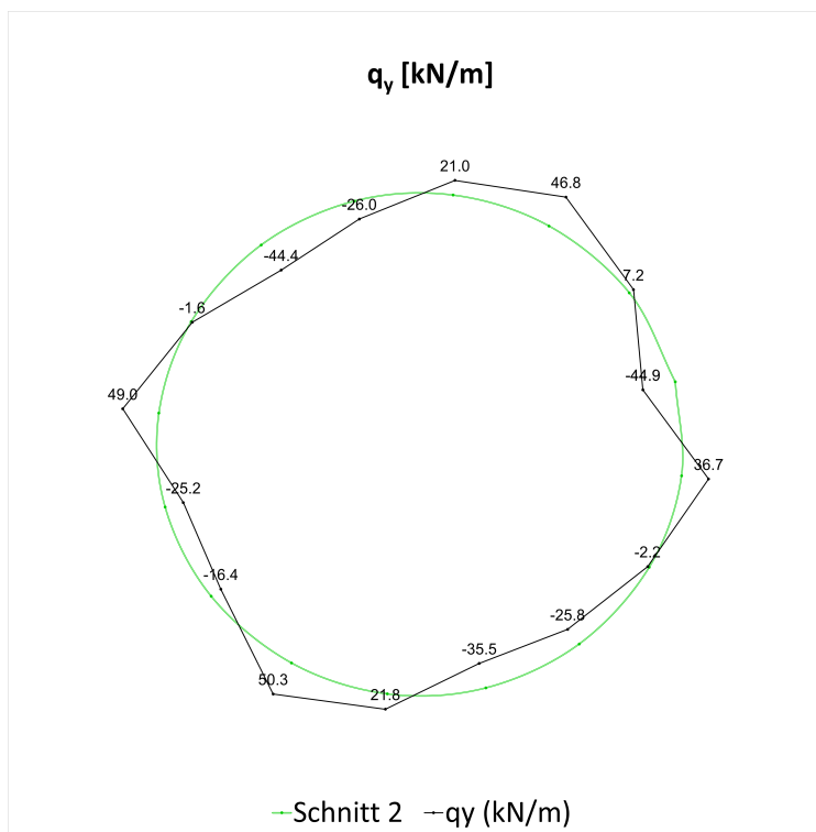
Fig. I-65: Querkraft ( Q_y ), Schnitt 2, 4 Jahre
