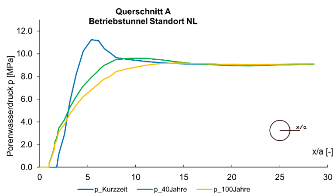
Fig. F-2: Porenwasserdruck entlang der Abfragelinie Parament
