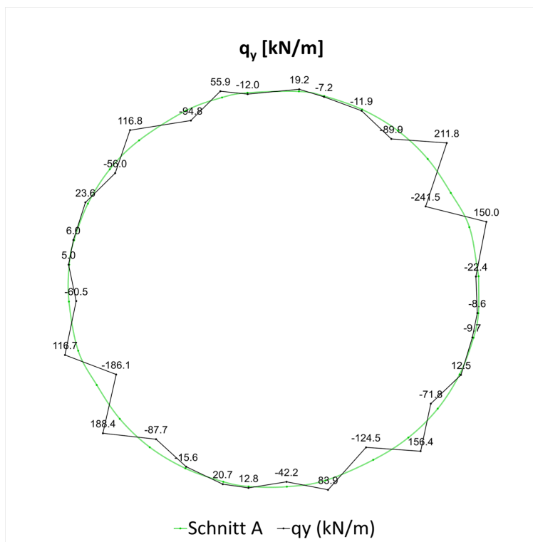
Fig. C-23 Querkraft ( Q_y ), Schnitt A, 100 Jahre
