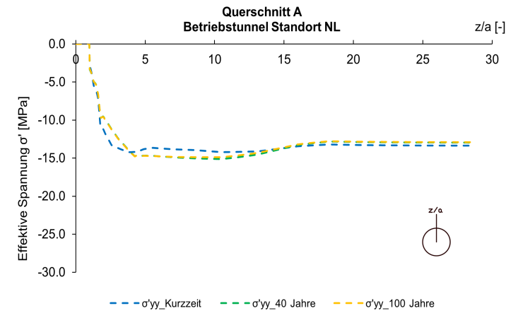
Fig. F-7: Spannung ( \sigma'_{yy} ) entlang der Abfragelinie Firste
