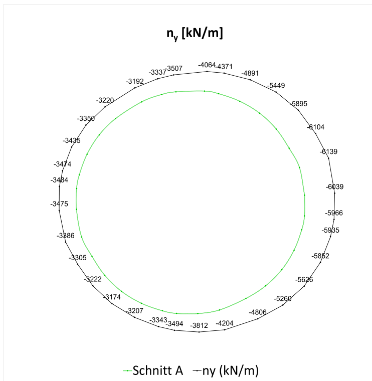
Fig. F-18: Normalkraft ( N_y ) in Umfangsrichtung, Schnitt A, 40 Jahre
