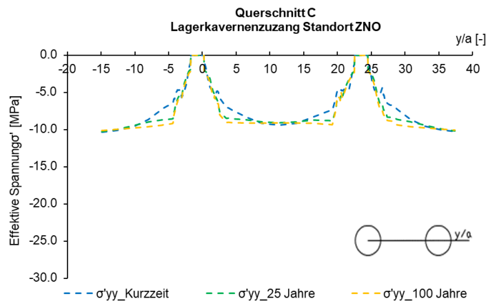
Fig. J-31: Spannung ( \sigma'_{yy} ) entlang der Abfragelinie Parament
