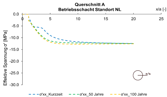
Fig. M-2: Spannung ( \sigma'_{xx} ) entlang der Abfragelinie
