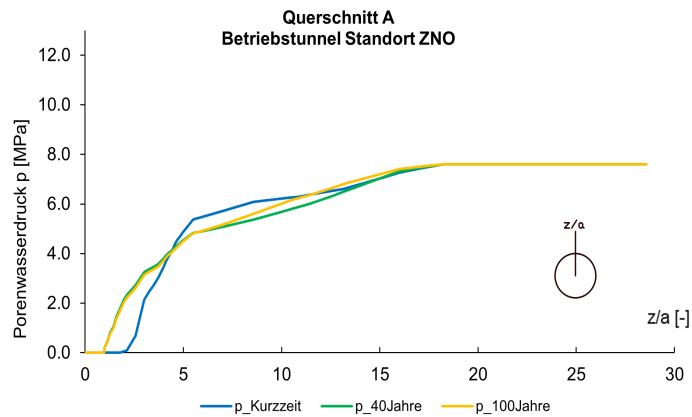
Fig. I-3: Porenwasserdruck entlang der Abfragelinie Firste
