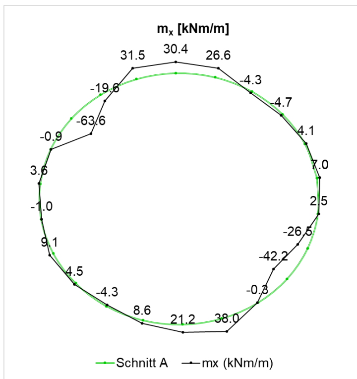
Fig. G-22: Biegemoment ( M_x ), Schnitt A, 100 Jahre
