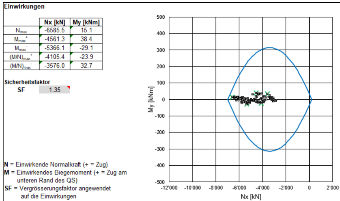
Fig. E-13: Tragsicherheitsnachweis, Schnitt 3, 50 Jahre, Spritzbetonschale (C30/37): 35 cm
